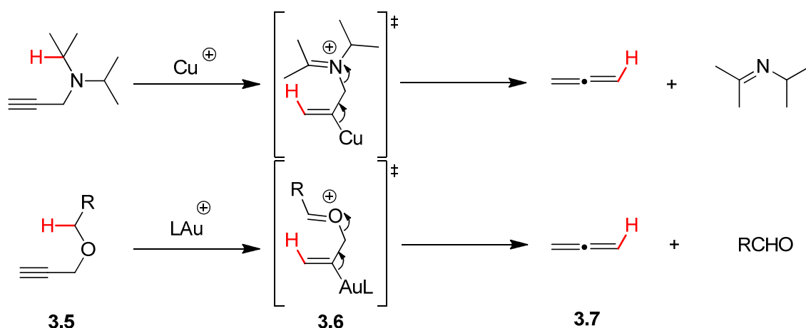
Schéma 110: Principe de la transformation proposée
