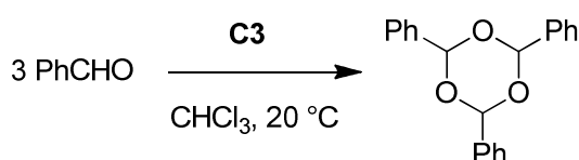
Schéma 208: Processus compétitif consommant le benzaldéhyde
