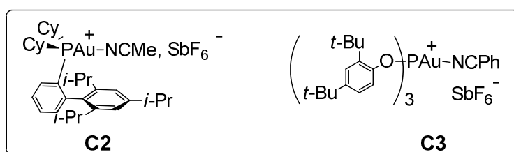
Schéma 185: Choix du système catalytique
