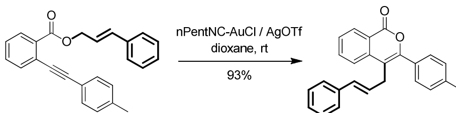
Schéma 52: Alkylation d'un intermédiaire vinyl or 78
