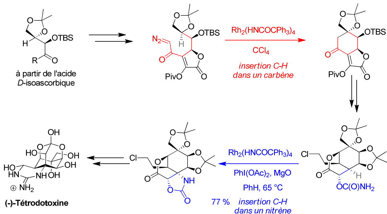
Schéma 66: Synthèse totale de la (-)-Tétrodotoxine utilisant deux insertions C-H dans un carbène puis dans un nitrène 102
