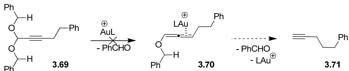
Schéma 129: Tentative infructueuse d'isomérisation d'un alcyne
