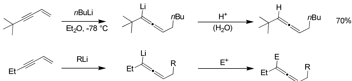
Schéma 102: addition 1,4 sur un ényne
