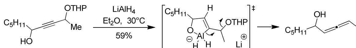
Schéma 105: Utilisation d'un hydrure métallique comme nucléophile intramoléculaire
