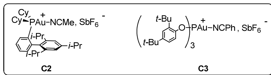
Schéma 161: Détermination des conditions de catalyse
