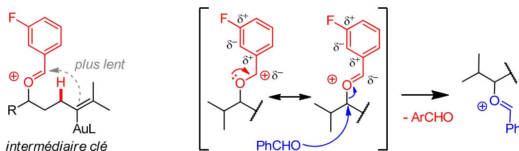
Schéma 202: Effet du fluor en position méta du benzyle
