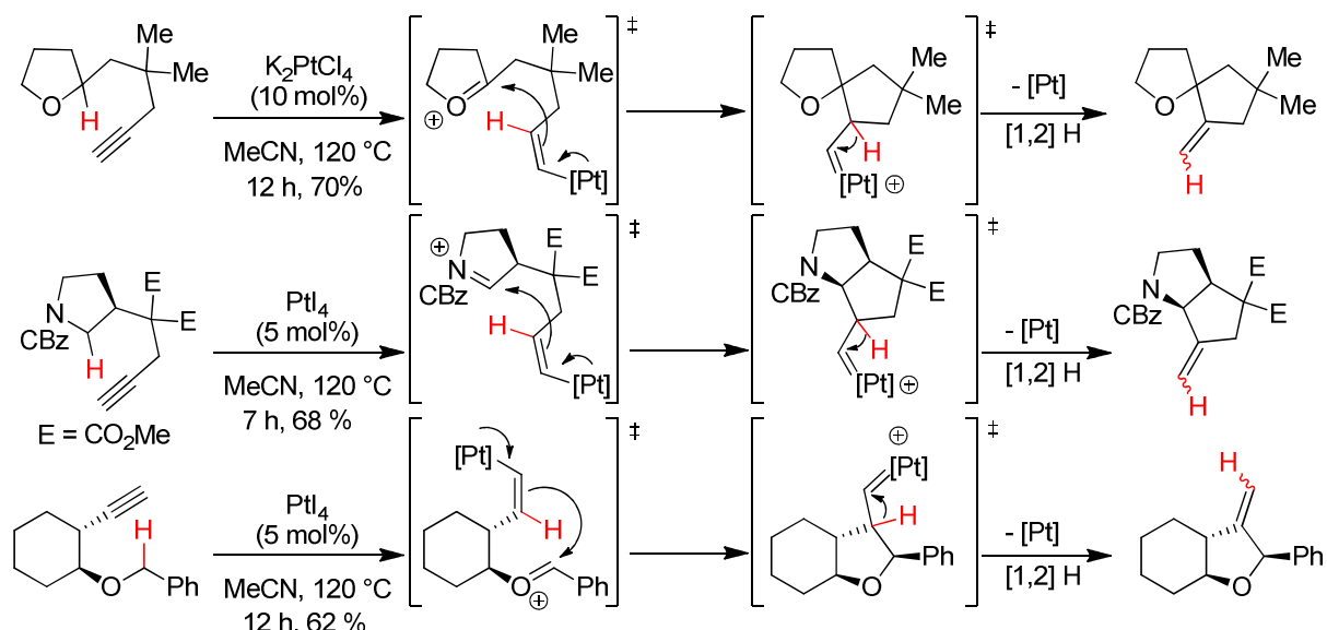
Schéma 142: Méthodologie au platine développée par Sames
