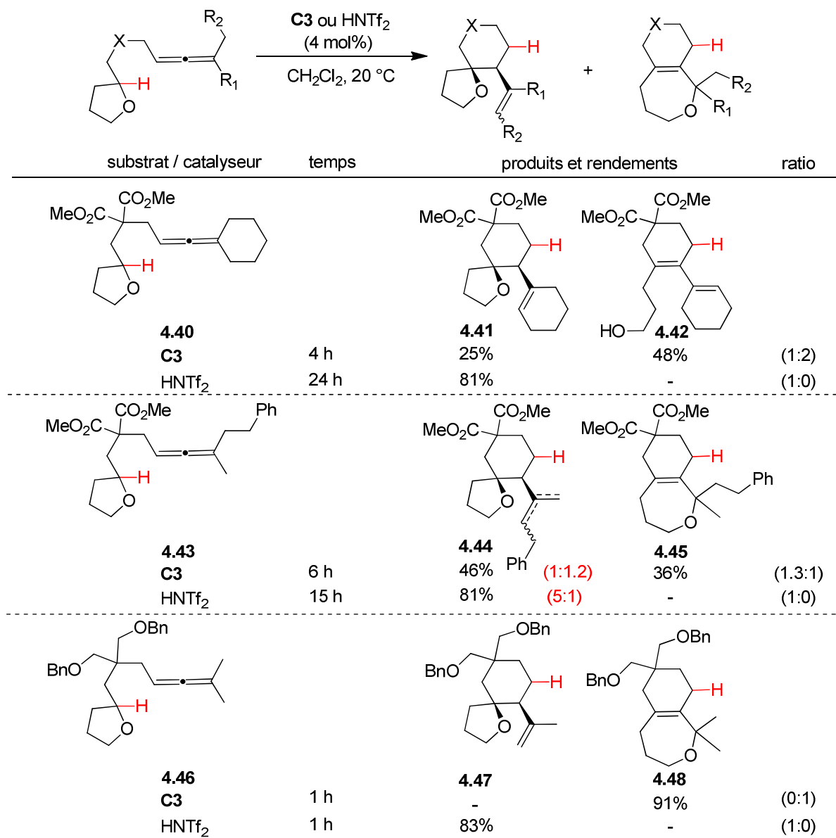
Schéma 153: Etendue de la réaction
