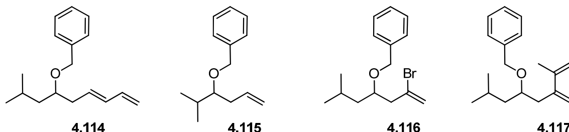
Schéma 173: Différents substrats non réactifs testés
