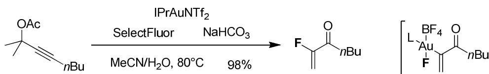
Schéma 49: Élimination réductrice d'un vinyl or (III) menant à une fluoro-oléfine 73
