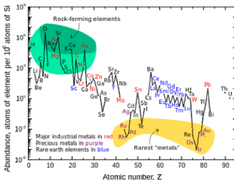
Schéma 1: Abondance relative des métaux précieux utilisés en catalyse 1
