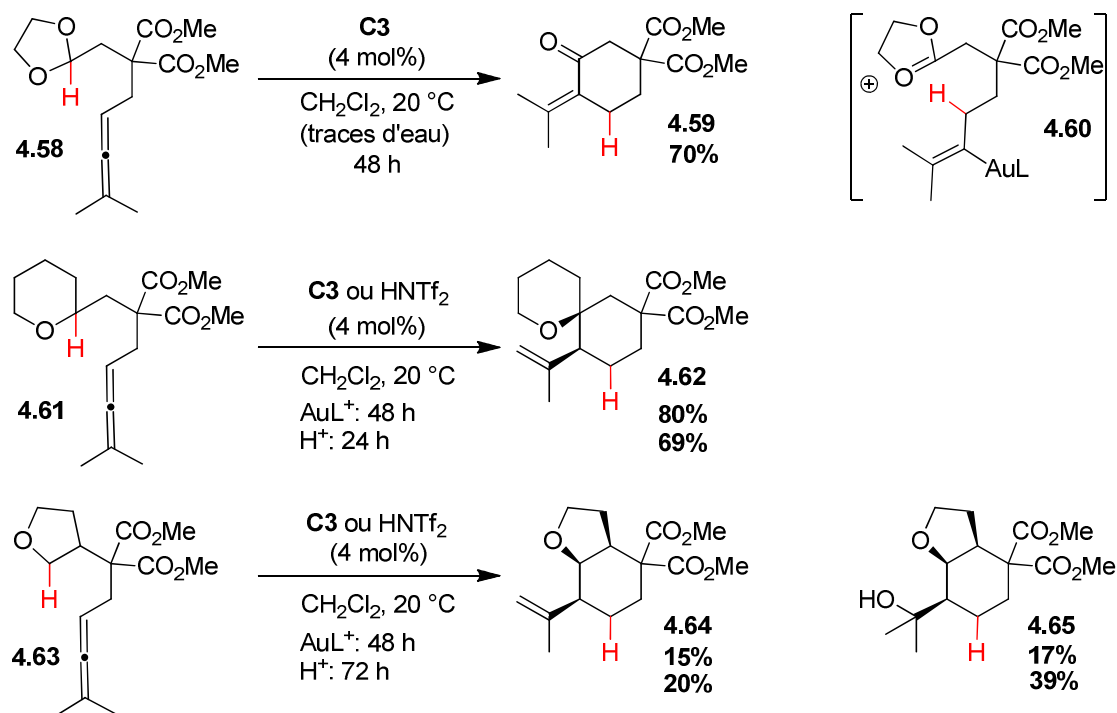
Schéma 156: Utilisation de différents donneurs d'hydruure
