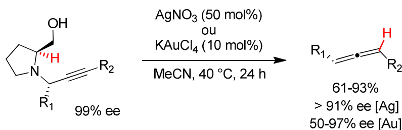
Schéma 109: Modifications de Che et coll.
