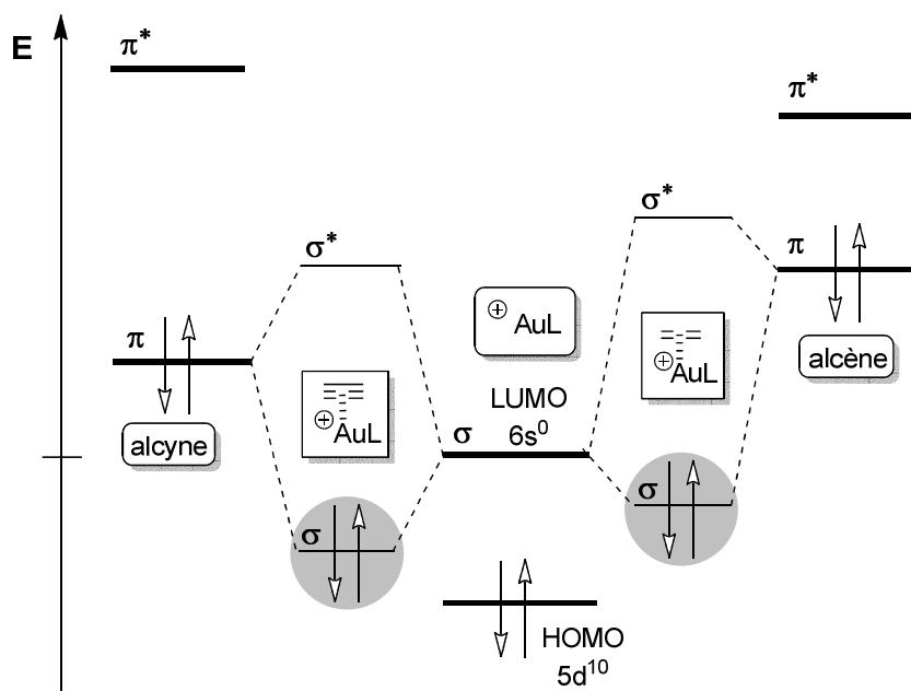
Schéma 16: Principe de l'activation électrophile des systèmes \pi par un complexe d'or
