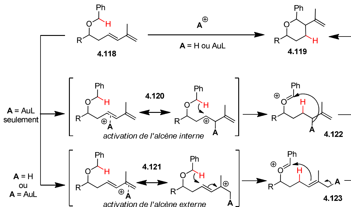
Schéma 174: Mécanismes envisagés pour l'activation des diènes par catalyse
