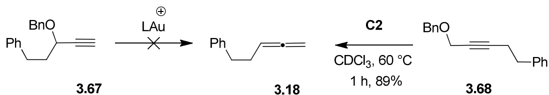
Schéma 128: Préparation d'allènes terminaux
