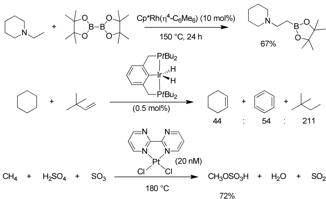
Schéma 61: Valorisation d'alcanes non réactifs par fonctionnalisation C-H 93
