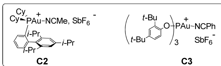
Schéma 185: Choix du système catalytique
