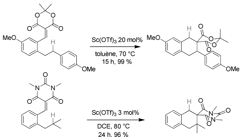
Schéma 80: Utilisation de liaisons C-H ( sp^3 ) benzyliques ou tertiaires comme donneurs d'hydrure 117,118
