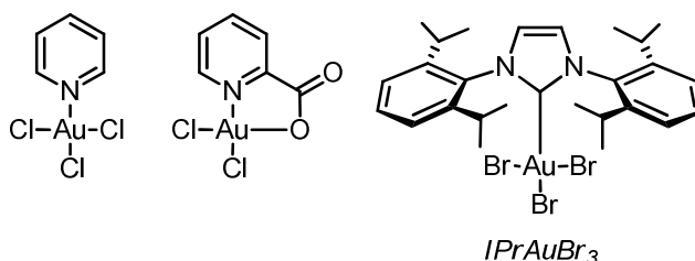
Schéma 7: Des complexes d'or (III) utilisés en catalyse homogène
