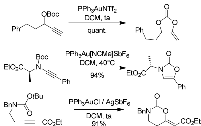
Schéma 22: Utilisation de la fonction tert butoxycarbonate comme nucléophile intramoléculaire 33
