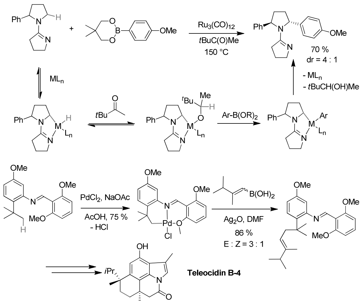
Schéma 62: Exemples d'activations de liaisons C-H ( sp^3 ) dirigées par des imines 94a
