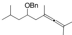
Schéma 171: allène tétrasubstitué 4.109
