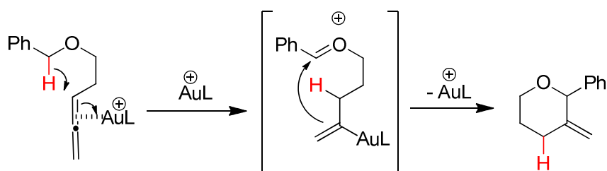
Schéma 159: Principe de la transformation
