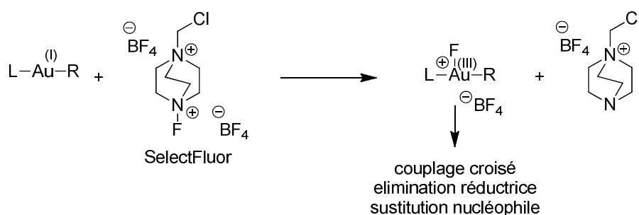
Schéma 45: Concept de l'utilisation du SelectFluor pour la catalyse à l'or
