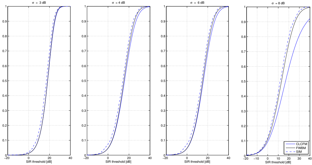
Figure 1: Comparaison des méthodes FWBM, CLCFM et avec les résultats issus de simulations. Influence de l'écart-type de l'effet de masque \sigma [dB] ( r = 0.2 Km and \eta = 3.0 ).
