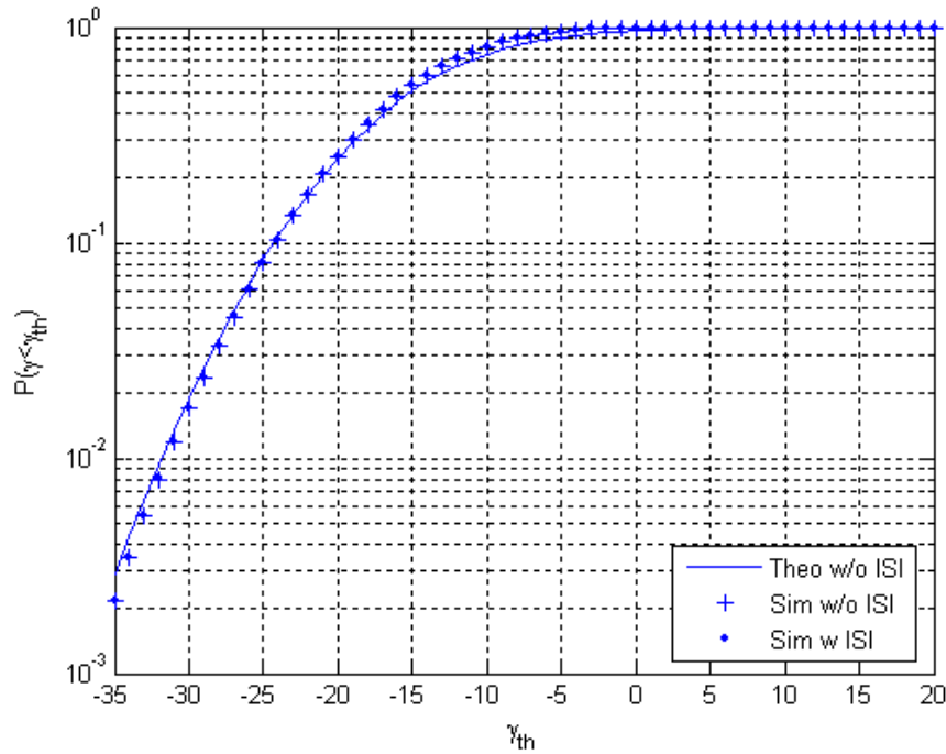
Figure 3: Comparaison entre résultats de simulations et expressions analytiques de la probabilité de coupure avec et sans ISI en utilisant le RT pour 18 BSs interférentes.
