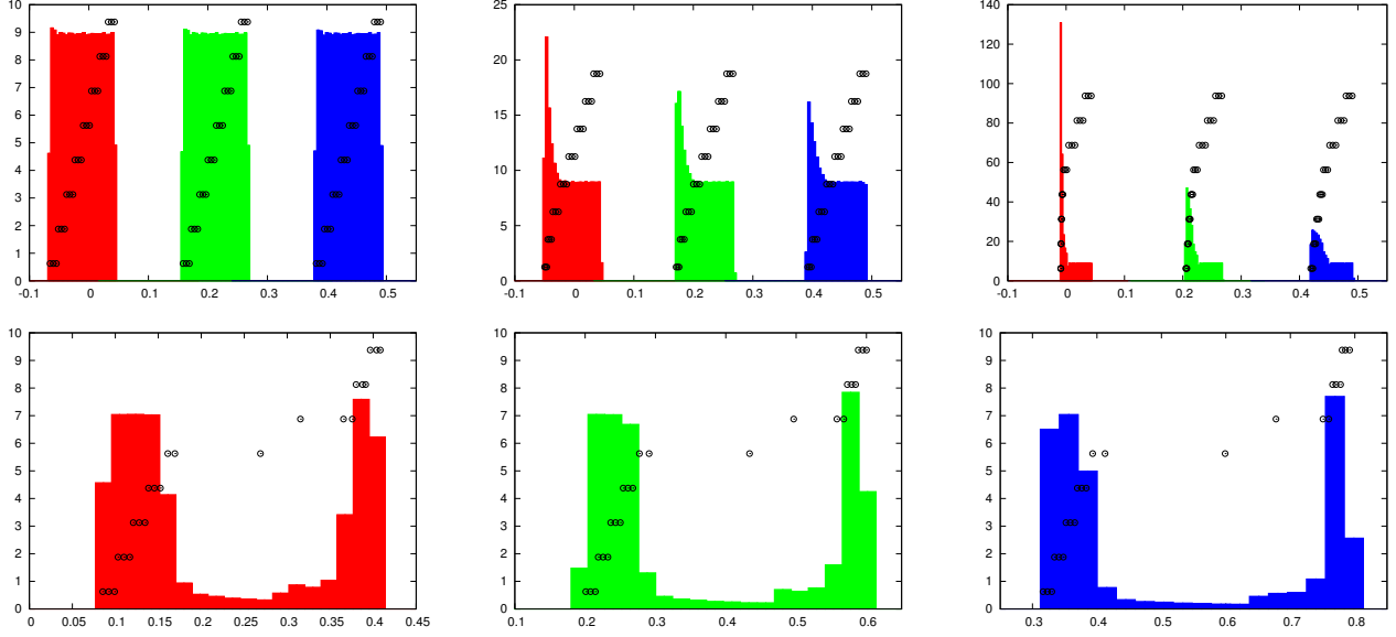
FIGURE 3.34 – Cas test 5 (Euler) : Valeurs propres approchées ( v_{LR}^{\text{Roe},*} - c_{LR}^{\text{Roe},*} )( \xi_\eta ) _{\eta \in \mathcal{P}_\pi} (rouge/gris), v_{LR}^{\text{Roe},*} ( \xi_\eta ) _{\eta \in \mathcal{P}_\pi} (vert/gris clair) et ( v_{LR}^{\text{Roe},*} + c_{LR}^{\text{Roe},*} )( \xi_\eta ) _{\eta \in \mathcal{P}_\pi} (bleu/gris foncé) correspondant à chaque élément stochastique avec leurs fonctions de densité pour x = 0.15 , x = 0.2 , x = 0.25 (en haut) et x = 0.9 (en bas). Calculs à l’instant t = 1 avec \text{Nr} = 3 et \text{No} = 2 .
