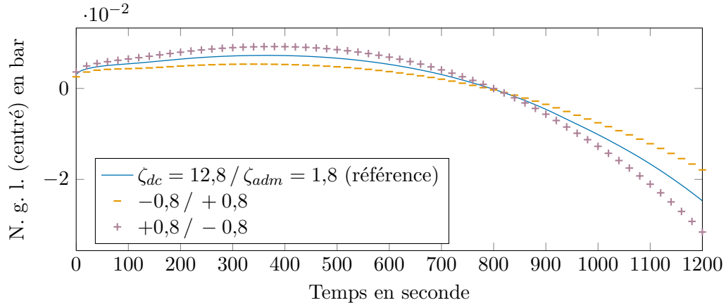
Figure 6.3. : Effet d’une perturbation du coefficient M_{\bar{v}r} sur la réponse du n. g. l. lors d’un essai R.G.L. 4. Les moyennes temporelles des courbes leur ont été soustraites. Le calage des autres coefficients et paramètres n’a pas été ajusté après les perturbations car elles sont de faible amplitude. L’effet des perturbations est amplifié 5 fois.
