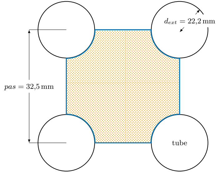
Figure 5.2. : Schéma d'un sous-canal de l'écoulement secondaire diphasique. Le rayon hydraulique est égal au rapport de la surface marquée par des points orange par le périmètre en trait épais bleu. Le diamètre hydraulique vaut 4 fois le rayon hydraulique.
