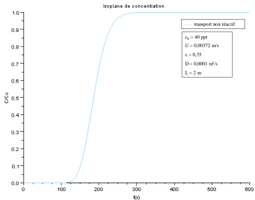
Figure 35 : Concentration normalisée en fonction du temps en régime convectif–dispersif en conditions réelles ( L=2 m et Q=10 m 3 .h -1 ) dans le cadre d'un transport non réactif
