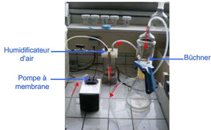
Figure 135 : Photographie du dispositif expérimental pour sécher la résine
