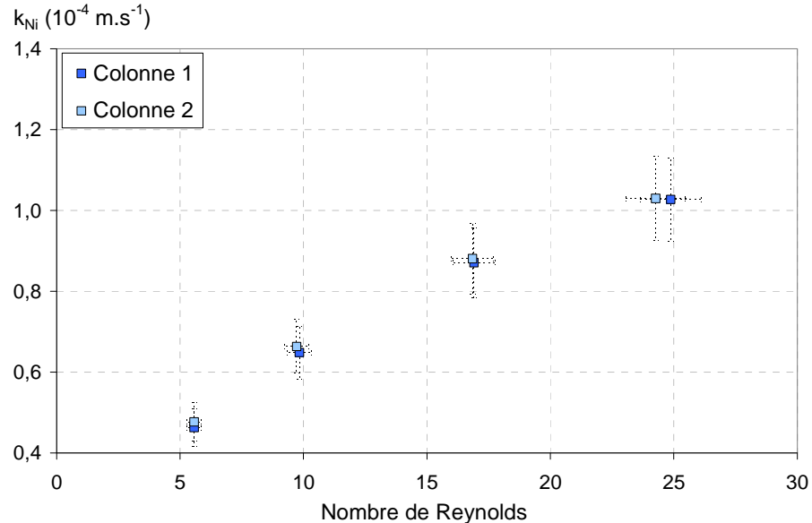
Figure 72 : Evolution du MTC du Nickel en fonction du nombre de Reynolds (pour une vitesse de filtre comprise entre 3,72 \cdot 10^{-3} et 1,66 \cdot 10^{-2} m.s -1 ), pour une hauteur d'IRN97H de 4,5 cm (Colonne 1 \blacksquare ) et de 4,4 cm (Colonne 2 \square ), avec une concentration de Nickel en entrée de 20,3 ppm
