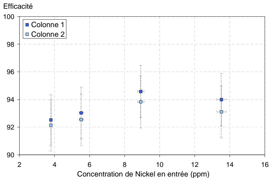
Figure 74 : Evolution de l'efficacité en fonction de la concentration de Nickel en entrée (comprise entre 3,8 et 13,5 ppm), pour une hauteur d'IRN97H de 4,6 cm (Colonne 1 \blacksquare ) et de 4,4 cm (Colonne 2 \square ), avec une vitesse de filtre de 1,02 \cdot 10^{-2} \text{ m.s}^{-1}
