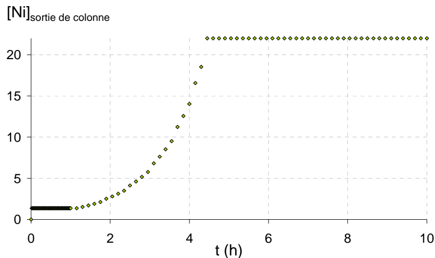
Figure 106 : Simulation sur OPTIPUR option Nernst (losange citron vert) présentant l'évolution de la concentration de nickel en sortie de colonne en fonction du temps en condition type cas de référence ( L=4,5 cm ; U_z=1,13.10^{-2} m.s -1 ; C_{Ni}^{entrée}=21,5 ppm)
