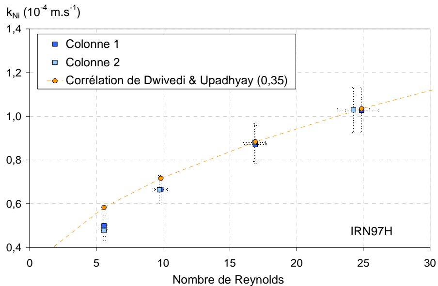
Figure 88 : Evolution du MTC du Nickel obtenu expérimentalement (Colonne 1 \blacksquare , 2 \square ) et à partir de la corrélation de Dwivedi & Upadhyay (avec une porosité de 0,35 \bullet pour la Colonne 1) en fonction du nombre de Reynolds (pour une vitesse de filtre comprise entre 3,72 \cdot 10^{-3} et 1,66 \cdot 10^{-2} \text{ m.s}^{-1} ), pour une hauteur d'IRN97H de 4,5 cm (Colonne 1 \blacksquare ) et de 4,4 cm (Colonne 2 \square ), avec une concentration de Nickel en entrée de 20,3 ppm ;
