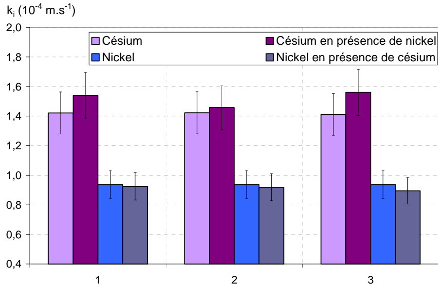
Figure 85 : Evolution du MTC du Nickel et du Césium en fonction des constituants présents dans la solution initiale
