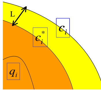
Figure 50 : Schéma représentatif des concentrations dans une bille de résine en fonction de leur localisation
