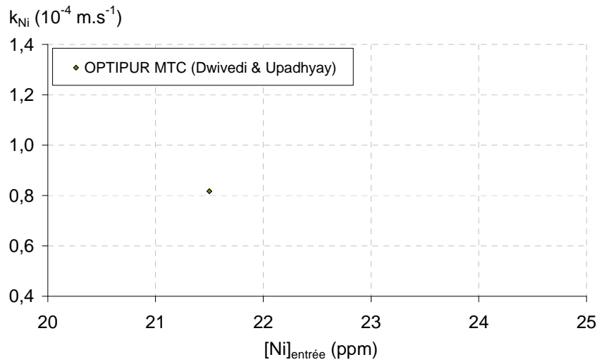
Figure 109 : Coefficient de transfert de masse du Nickel en fonction de la concentration de nickel en entrée en condition type cas de référence ( L=4,5 cm ; U_z=1,13 \cdot 10^{-2} m.s -1 ; C_{Ni}^{entrée}=21,5 ppm) obtenu grâce à OPTIPUR option MTC (obtenue par la corrélation de Dwivedi & Upadhyay)
