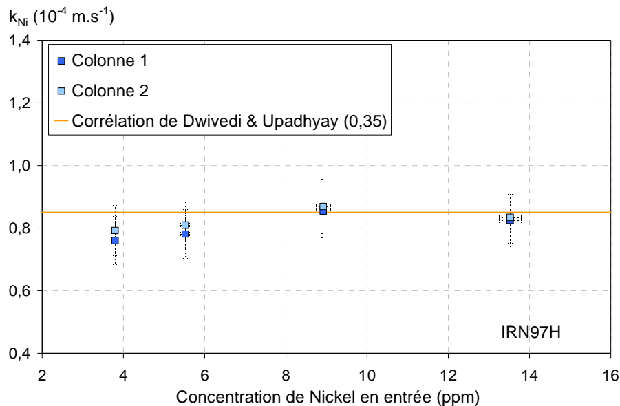
Figure 90 : Evolution du MTC du Nickel obtenu expérimentalement (Colonnes 1 et 2) et à partir de la corrélation de Dwivedi & Upadhyay (pour la Colonnes 1 avec une porosité de 0,35) en fonction de la concentration de Nickel en entrée (comprise entre 3,8 et 13,5 ppm), avec une vitesse de filtre de 1,02 \cdot 10^{-2} \text{ m.s}^{-1} , pour une hauteur d'IRN97H de 4,6 cm (Colonnes 1) et de 4,4 cm (Colonnes 2)
