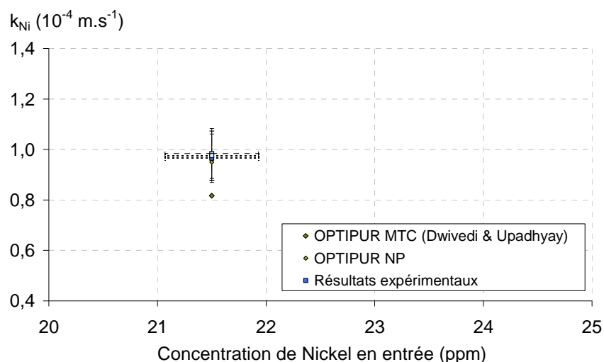
Figure 111 : Coefficient de transfert de masse du Nickel en fonction de la concentration de nickel en entrée en condition type cas de référence ( L=4,5 cm ; U_z=1,13.10^{-2} m.s ^{-1} ; C_{Ni}^{entrée}=21,5 ppm) obtenu grâce à OPTIPUR option MTC (obtenue par la corrélation de Dwivedi & Upadhyay) (losange vert foncé) ; OPTIPUR option NP (losange vert clair) et des résultats expérimentaux (carré bleu : foncé, moyen et clair).
