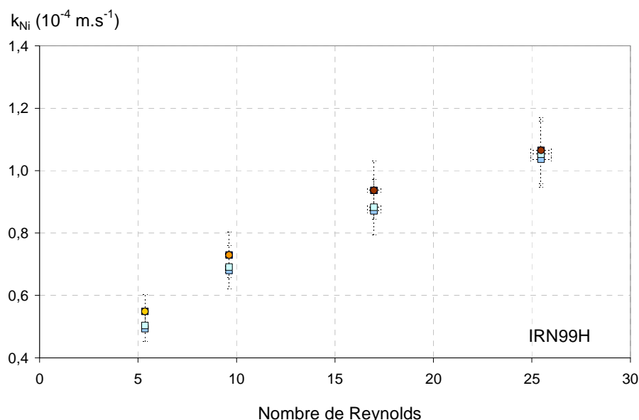
Figure 113 : Evolution du MTC du Nickel obtenu expérimentalement (Colonne 1 \square , 2 \square et 3 \square ) et à partir de la corrélation de Dwivedi & Upadhyay (avec une porosité de 0,34 \bullet , de 0,35 \bullet et de 0,36 \bullet ) en fonction du nombre de Reynolds (pour une vitesse de filtre comprise entre 3,77 \cdot 10^{-3} et 1,70 \cdot 10^{-2} m.s -1 ), pour une hauteur d'IRN99H de 4,4 cm (Colonne 1 \square ), de 4,4 cm (Colonne 2 \square ) et de 4,2 cm (Colonne 3 \square ), et avec une concentration de Nickel en entrée de 18,40 ppm
