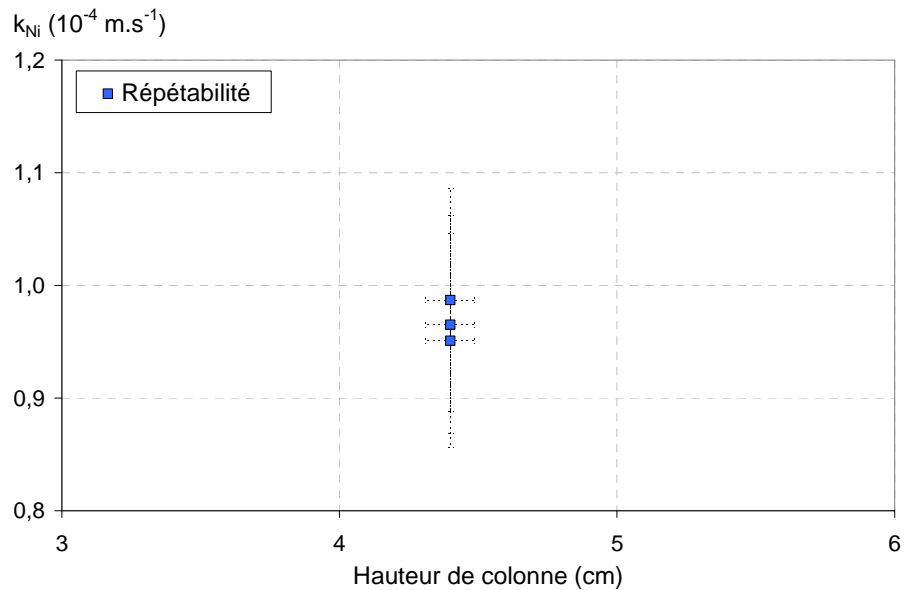
Figure 68 : Essai de répétabilité sur le MTC du Nickel réalisé trois fois de suite sur la même colonne remplie d'IRN97H sur une hauteur de 4,4 cm (colonne 1 ■), avec une concentration de Nickel en entrée de 21,5 ppm et une vitesse de filtre de 1,13.10^{-2} \text{ m.s}^{-1}
