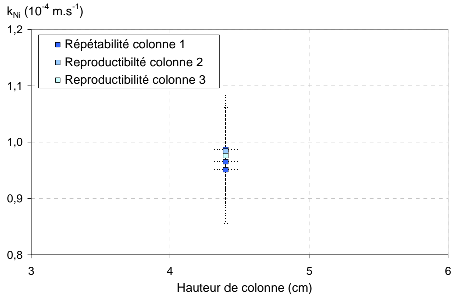
Figure 69 : Essai de répétabilité et de reproductibilité sur le MTC du Nickel pour une hauteur d'IRN97H de 4,5 cm (colonne 1 \blacksquare , colonne 2 \square et colonne 3 \square ), avec une concentration de Nickel en entrée de 21,5 ppm et une vitesse de filtre de 1,13 \cdot 10^{-2} \text{ m.s}^{-1} .
