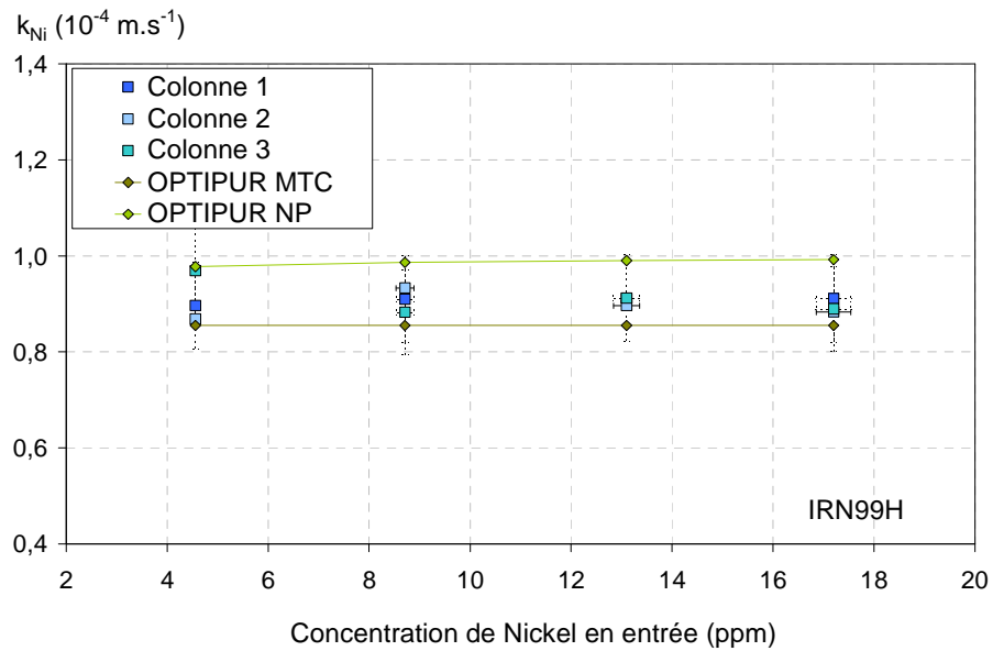
Figure 117 : Evolution du MTC du Nickel obtenu expérimentalement (Colonne 1 ■ et 2 ■ ) et par simulation sur OPTIPUR (option MTC ◆ et option NP ◆ pour la Colonne 1) en fonction de la concentration de Nickel en entrée (comprise entre 3,8 et 13,5 ppm), avec une vitesse de filtre de 1,02 \cdot 10^{-2} \text{ m.s}^{-1} , pour une hauteur d'IRN97H de 4,6 cm (Colonne 1 ■ ) et de 4,4 cm (Colonne 2 ■ )
