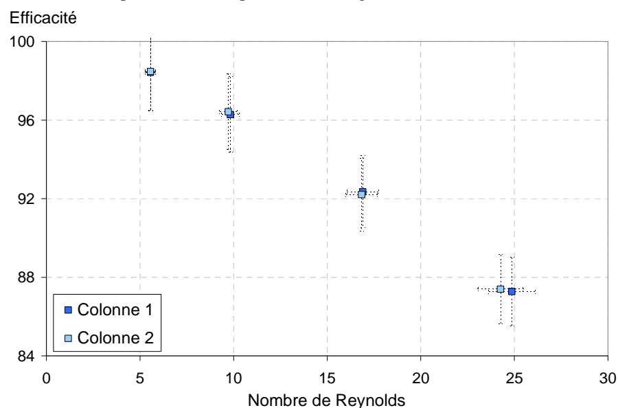
Figure 71 : Evolution de l'efficacité en fonction du nombre de Reynolds (pour une vitesse de filtre comprise entre 3,72 \cdot 10^{-3} et 1,66 \cdot 10^{-2} \text{ m.s}^{-1} ), pour une hauteur d'IRN97H de 4,5 cm (Colonne 1 \blacksquare ) et de 4,4 cm (Colonne 2 \square ), avec une concentration de Nickel en entrée de 20,3 ppm
