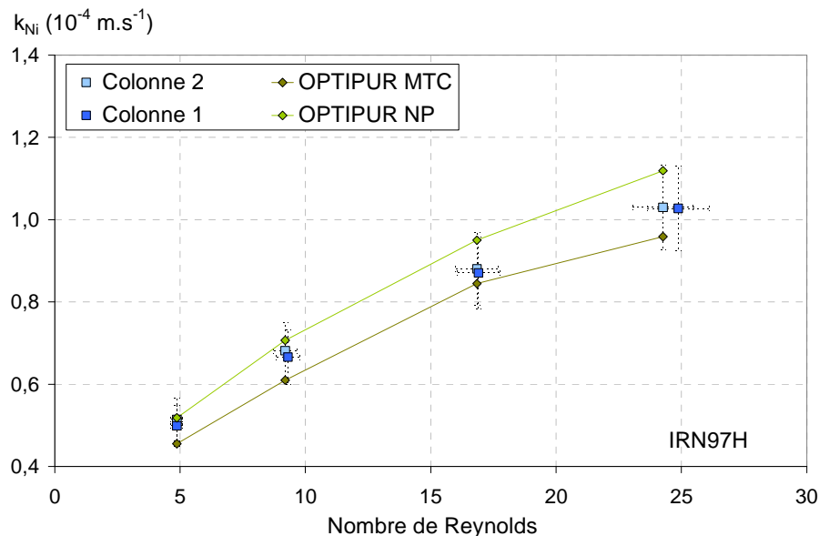
Figure 114 : Evolution du MTC du Nickel obtenu expérimentalement (Colonne 1 \square et 2 \square ) et à partir de la simulation sur OPTIPUR (option MTC \blacklozenge et option NP \blacklozenge ) en fonction du nombre de Reynolds (pour une vitesse de filtre comprise entre 3,77 \cdot 10^{-3} et 1,70 \cdot 10^{-2} \text{ m.s}^{-1} ), avec une concentration de Nickel en entrée de 18,40 ppm et pour une hauteur d'IRN97H de 4,4 cm (Colonne 1 \square ) et de 4,4 cm (Colonne 2 \square )
