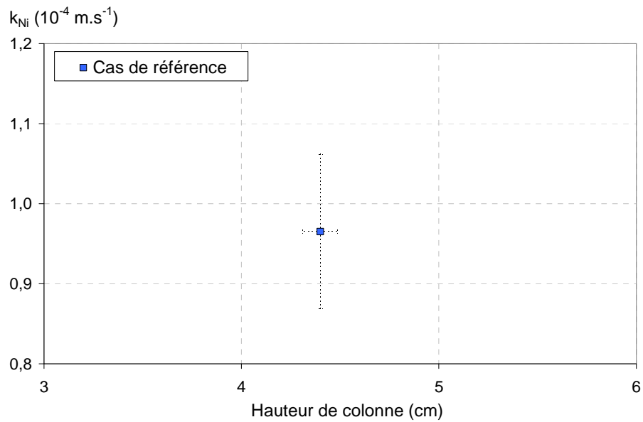
Figure 67 : Calcul du MTC du Nickel réalisée dans le cadre du cas de référence pour l'IRN97H ( d_p = 5,23.10^{-4} \text{ m} et \varepsilon = 0,35 ), avec une hauteur de 4,4 cm (■), une concentration de Nickel en entrée de 21,5 ppm et une vitesse de filtre de 1,13.10^{-2} \text{ m.s}^{-1} .
