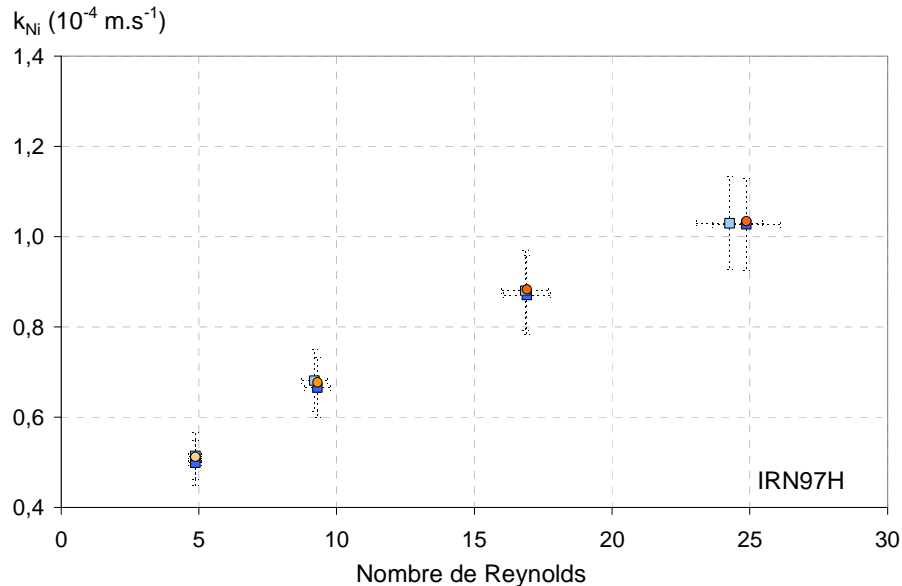
Figure 112 : Evolution du MTC du Nickel obtenu expérimentalement (Colonne 1 \blacksquare et 2 \blacksquare ) et à partir corrélation de Dwivedi & Upadhyay (avec une porosité de 0,35 \bullet , une porosité de 0,37 \circ et une porosité de 0,40 \circ ) en fonction du nombre de Reynolds (pour une vitesse de filtre comprise entre 3,72 \cdot 10^{-3} et 1,66 \cdot 10^{-2} \text{ m.s}^{-1} ), pour une hauteur d'IRN97H de 4,5 cm (Colonne 1 \blacksquare ) et de 4,4 cm (Colonne 2 \blacksquare ), avec une concentration de Nickel en entrée de 20,3 ppm
