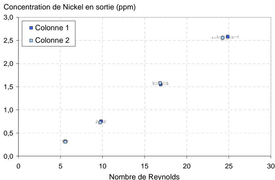
Figure 70 : Evolution de la concentration de Nickel en sortie en fonction du nombre de Reynolds (pour une vitesse de filtre comprise entre 3,72 \cdot 10^{-3} et 1,66 \cdot 10^{-2} \text{ m.s}^{-1} ), pour une hauteur d'IRN97H de 4,5 cm (Colonne 1 \blacksquare ) et de 4,4 cm (Colonne 2 \square ), avec une concentration de Nickel en entrée de 20,3 ppm
