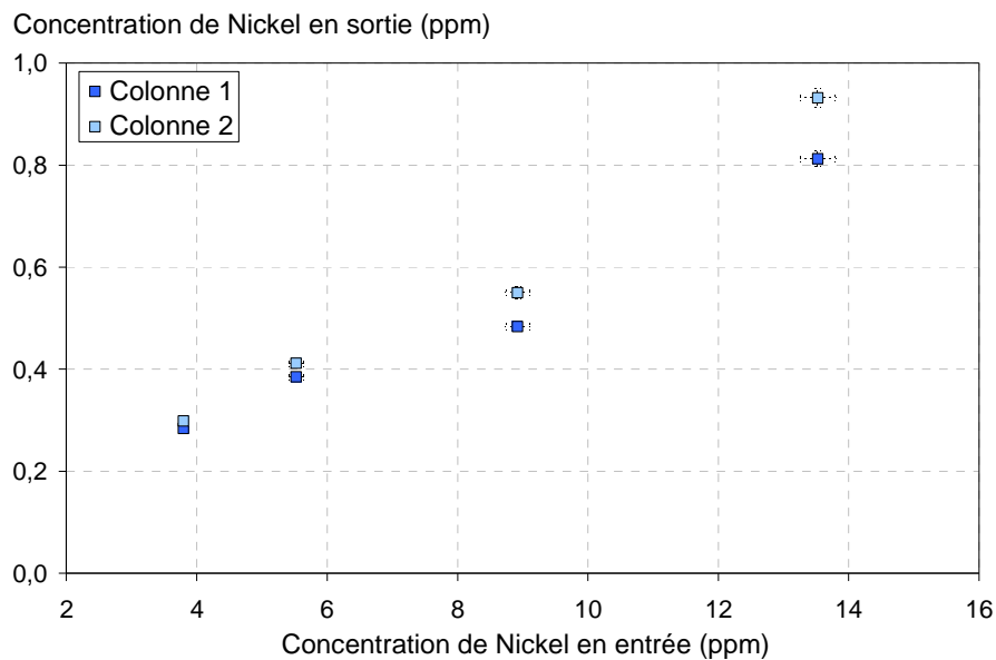
Figure 73 : Evolution de la concentration de Nickel en sortie en fonction de la concentration de Nickel en entrée (comprise entre 3,8 et 13,5 ppm), pour une hauteur d'IRN97H de 4,6 cm (Colonne 1 \blacksquare ) et de 4,4 cm (Colonne 2 \square ), avec une vitesse de filtre de 1,02 \cdot 10^{-2} \text{ m.s}^{-1}
