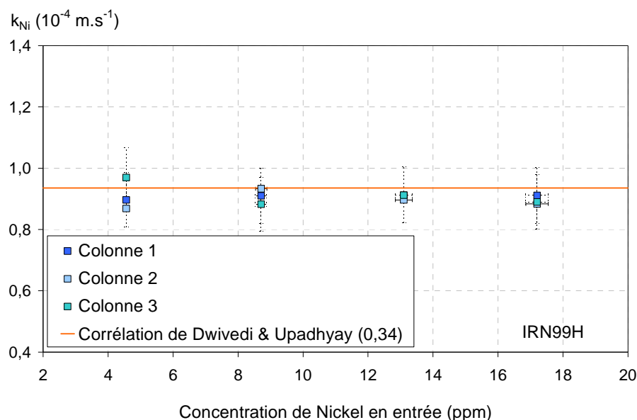
Figure 91 : Evolution du MTC du Nickel obtenu expérimentalement (Colonne 1 \blacksquare , 2 \square et 3 \blacksquare ) et à partir de la corrélation de Dwivedi & Upadhyay (pour la Colonne 1 \square avec une porosité calibrée de 0,34) en fonction de la concentration de Nickel en entrée (comprise entre 3,8 et 13,5 ppm), avec une vitesse de filtre de 1,02 \cdot 10^{-2} \text{ m.s}^{-1} , pour une hauteur d'IRN97H de 4,4 cm (Colonne 1 \blacksquare ), de 4,4 cm (Colonne 2 \square ) et de 4,2 cm (Colonne 3 \blacksquare )
