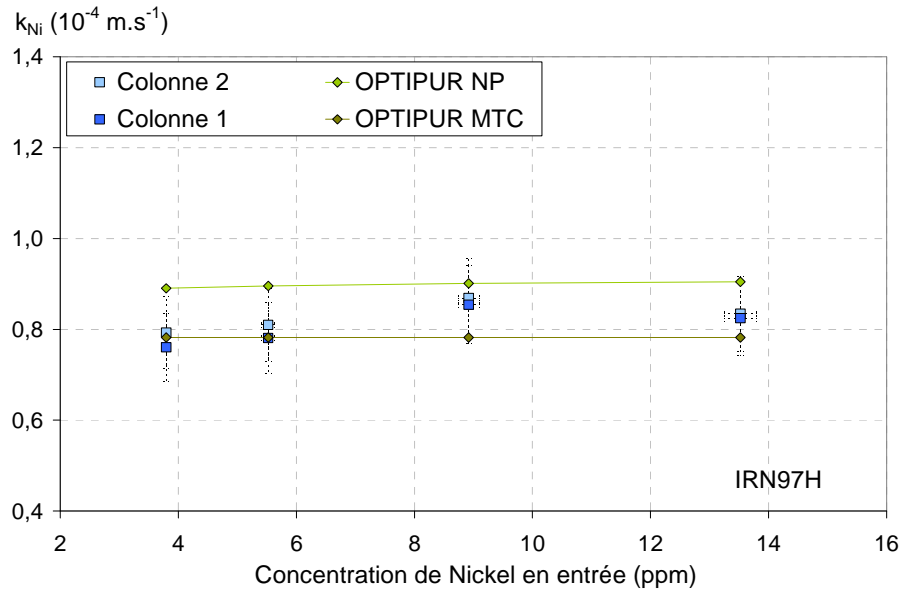
Figure 116 : Evolution du MTC du Nickel obtenu expérimentalement (Colonne 1 ■ , 2 ■ et 3 ■ ) et par simulation (option MTC ◆ et option NP ◆ pour la Colonne 1) en fonction de la concentration de Nickel en entrée (comprise entre 3,8 et 13,5 ppm), avec une vitesse de filtre de 1,02 \cdot 10^{-2} \text{ m.s}^{-1} , pour une hauteur d'IRN97H de 4,4 cm (Colonne 1 ■ ), de 4,4 cm (Colonne 2 ■ ) et de 4,2 cm (Colonne 3 ■ )
