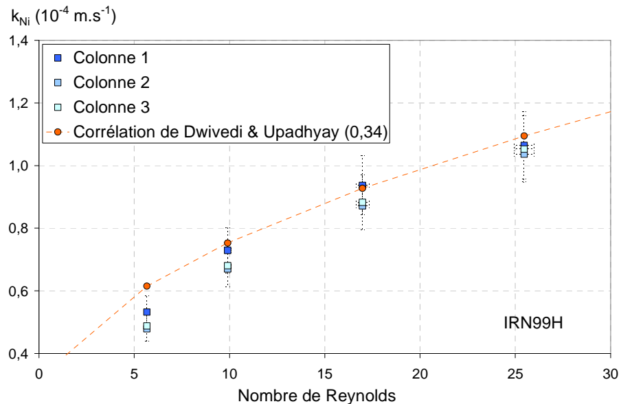
Figure 89 : Evolution du MTC du Nickel obtenu expérimentalement (Colonne 1 \blacksquare , 2 \square et 3 \square ) et à partir de la corrélation de Dwivedi & Upadhyay (avec une porosité de 0,34 \bullet pour la Colonne 1) en fonction du nombre de Reynolds (pour une vitesse de filtre comprise entre 3,77 \cdot 10^{-3} et 1,70 \cdot 10^{-2} \text{ m.s}^{-1} ), avec une concentration de Nickel en entrée de 18,40 ppm et pour une hauteur d'IRN99H de 4,4 cm (Colonne 1 \blacksquare ) et de 4,3 cm (Colonne 2 \square ), et de 4,2 cm (Colonne 3 \square ),
