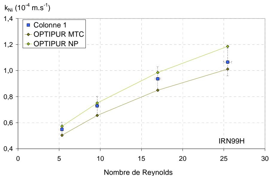
Figure 115 : Evolution du MTC du Nickel obtenu expérimentalement (Colonne 1 ■ ) et à partir de la simulation sur OPTIPUR (option MTC ◆ et option NP ◇ ) en fonction du nombre de Reynolds (pour une vitesse de filtre comprise entre 3,72 \cdot 10^{-3} et 1,66 \cdot 10^{-2} m.s -1 ), pour une hauteur d'IRN99H de 4,5 cm (Colonne 1 ■ ) et de 4,4 cm (Colonne 2 ■ ), avec une concentration de Nickel en entrée de 20,3 ppm
