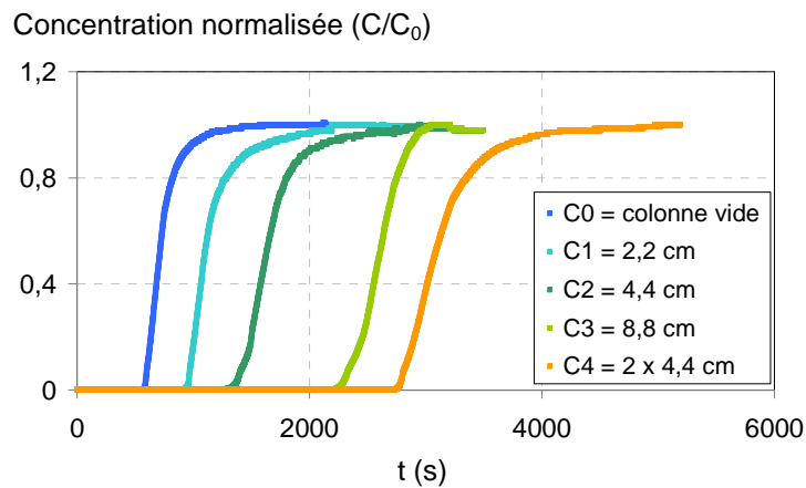
Figure 86 : Courbe d'éluion du traceur (chlorure) obtenue expérimentalement pour des colonnes de hauteur variable (comprise entre 0 et 8,8 cm)
