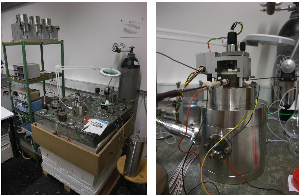
FIGURE 2.9 – Photographies du microscope à force atomique hydrothermal. À gauche, on distingue en hauteur les trois récipients pouvant contenir des solutions aqueuses. La photographie de droite est une vue de détail de la cellule hydrothermale dans laquelle est positionnée l'échantillon.
