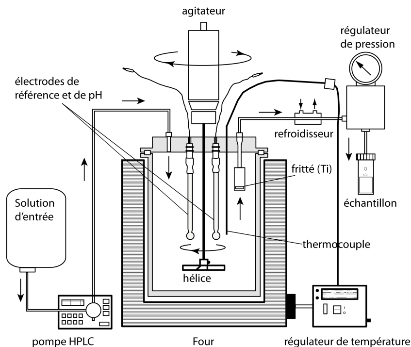
FIGURE 2.4 – Schéma d'un réacteur à circulation hydrothermal, utilisé pour les expériences de croissance cristalline de magnésite et d'hydromagnésite. Modifié d'après Saldi (2009).
