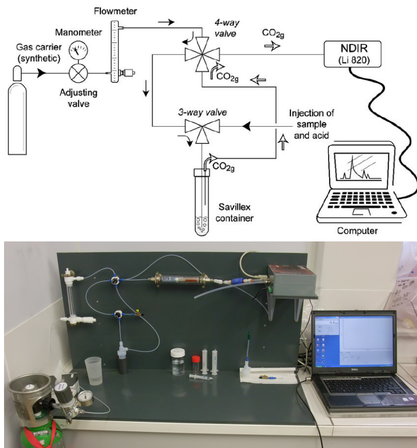
FIGURE 2.11 – Schéma (tiré de Bénézeth et al., 2011 ) et photo du dispositif analytique utilisé pour la mesure du carbone inorganique dissous par spectroscopie infrarouge non-dispersive.
