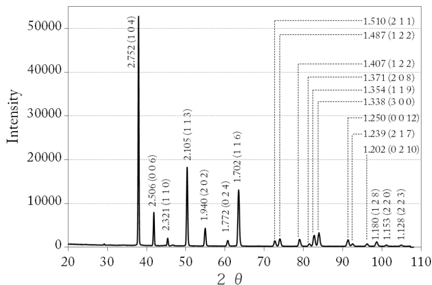
FIGURE 2.2 – Diffractogramme typique d'un échantillon de magnésite synthétisée. La distance réticulaire et l'indexation cristallographique des pics sont reportés. Tous les pics correspondent à la magnésite.
