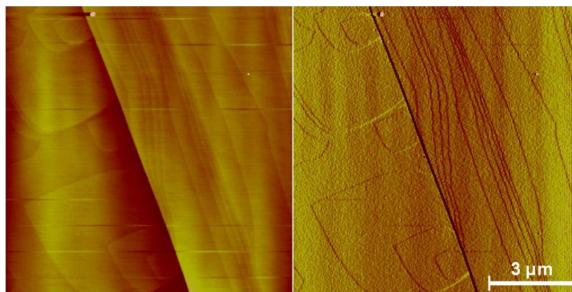
FIGURE 2.8 – Comparaison entre une image "en hauteur" (à droite) et "en déflexion" (à gauche) de marches cristallines observées pendant une expérience de croissance de la magnésite à 100°C. L'image en hauteur, reconstituée d'après les ajustements verticaux du tube piézoélectrique, contient des informations quantitatives sur la hauteur relative des différentes structures, tandis que l'image en déflexion, reconstituée d'après l'enregistrement de la déflexion du microlevier, permet d'observer un relief plus contrasté.
