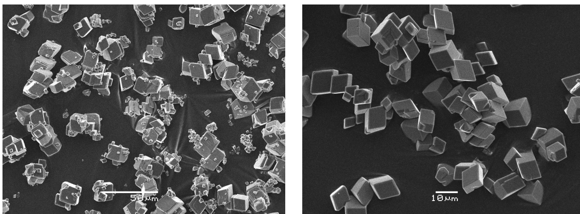
FIGURE 2.1 – Images MEB (électrons secondaires) de cristaux de magnésite synthétisés au cours de cette étude. À gauche, cristaux synthétisés à 225°C avant sélection granulométrique. À droite, exemple de cristaux obtenus après sélection granulométrique, et utilisés pour les expériences.
