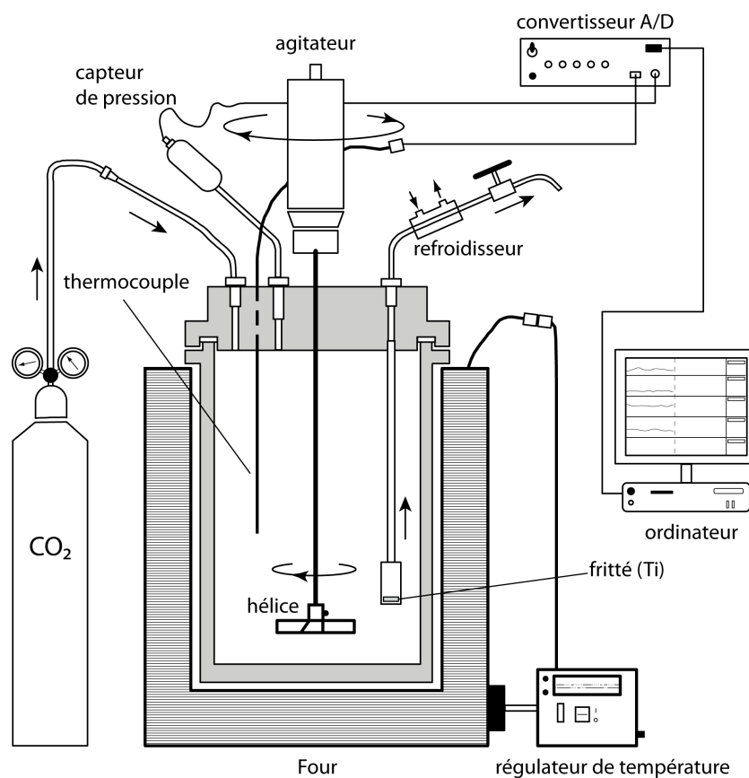
FIGURE 2.6 – Schéma d'un réacteur fermé en titane, utilisé pour la mesure de la solubilité de la magnésite en présence de citrate. Modifié d'après Saldi (2009).
