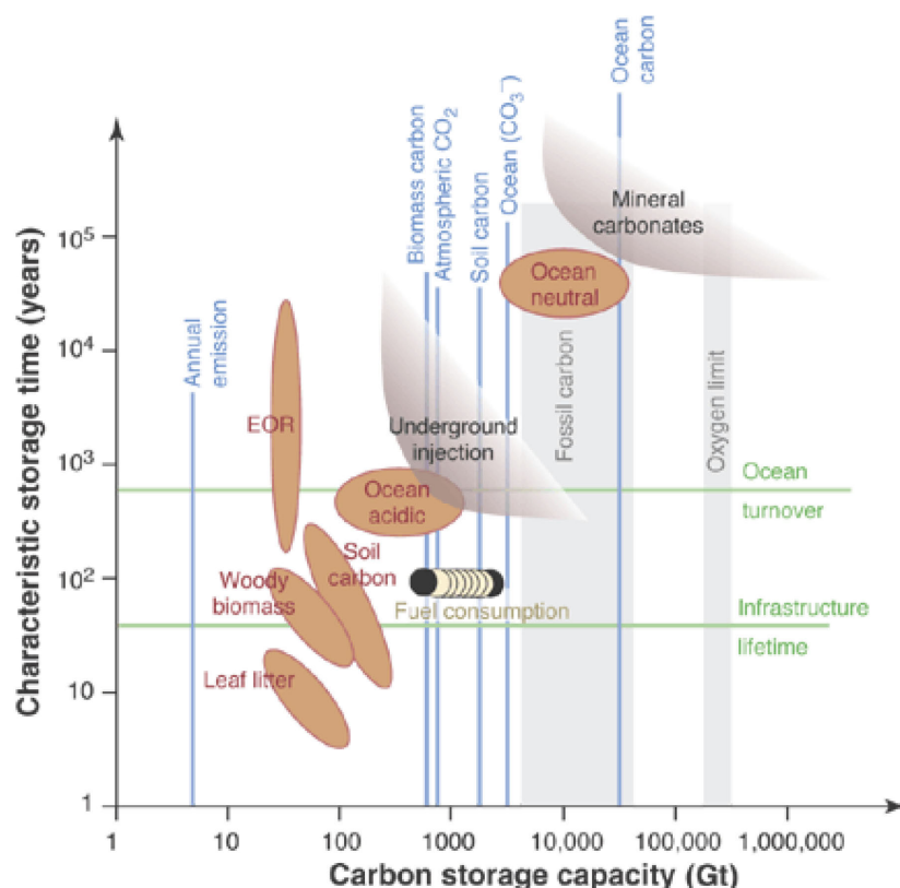
FIGURE 1.1 – Capacités disponibles et durées de temps estimées pour différentes méthodes de séquestration du CO 2 . Source : Lackner (2003).
