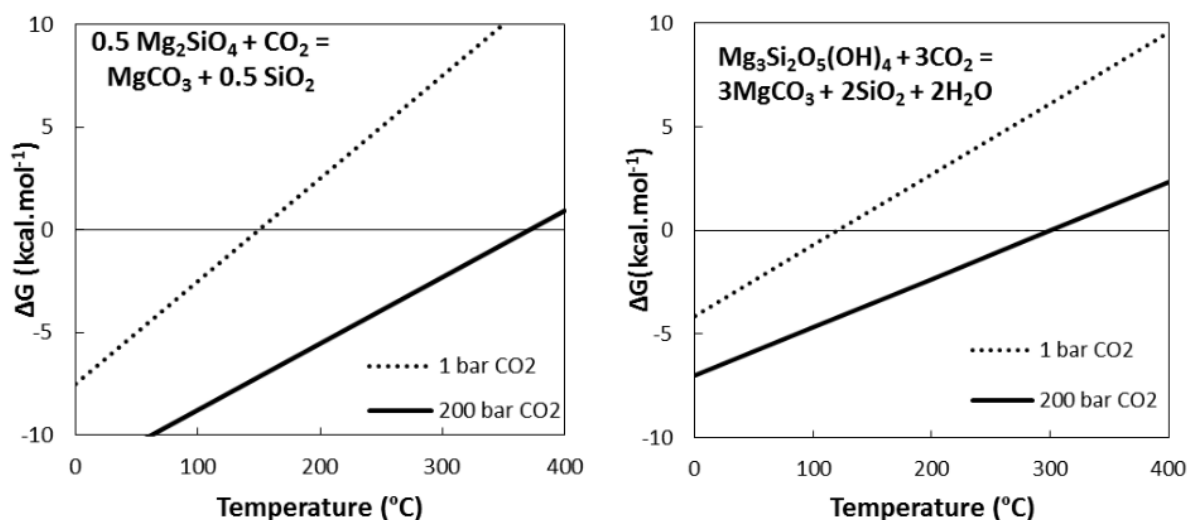
FIGURE 1.2 – Énergie libre de la réaction de carbonatation de la forstérite (gauche) et du chrysotile (droite) en fonction de la température. D'après Declercq et Oelkers (2012).
