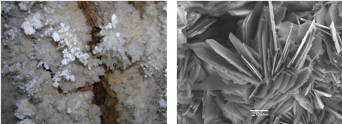
FIGURE 2.3 – Images des cristaux d'hydromagnésite naturelle utilisés dans l'étude. Gauche : efflorescences d'hydromagnésite sur concrétions d'aragonite dans les grottes du réseau André Lachambre. Droite : image MEB (électrons secondaires) des cristaux d'hydromagnésite constituant les efflorescences.
