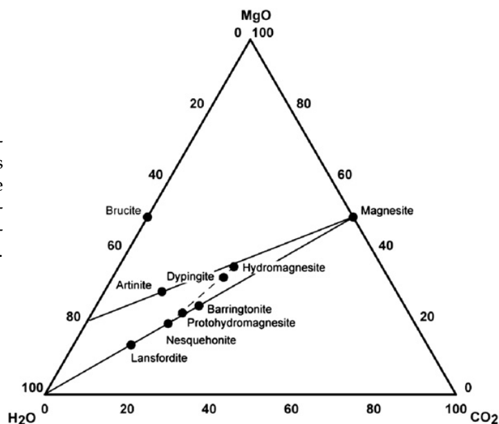
FIGURE 1.3 – Diagramme compositionnel représentant les phases minérales principales se formant dans le système MgO-CO 2 -H 2 O. La ligne pointillée représente les phases intermédiaires précipitées par Davies et Bubela (1973). Source : Bénézeth et al. (2011).
