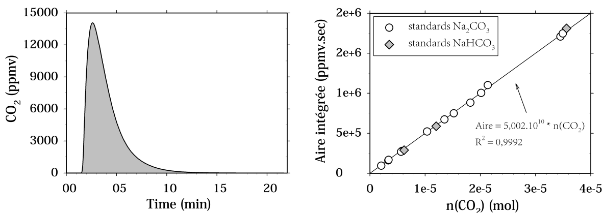
FIGURE 2.12 – Gauche : Évolution de la concentration en CO 2 dans le gaz porteur au cours du temps, après injection d'HCl dans l'échantillon à analyser. La droite de calibration (à droite) est établie en reliant la surface de l'aire grisée à la quantité de CO 2 dans l'échantillon.
