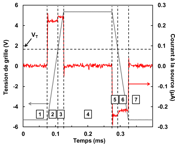
Figure 4.2-3 Courant à la source (courbe rouge) d'un a\text{-Si:H} TFT avec W/L = 50\mu\text{m}/10\mu\text{m} , dans le cas quasi-statique sous la tension V_{DS} nulle et sous la pulse de tension de grille (courbe grise).
