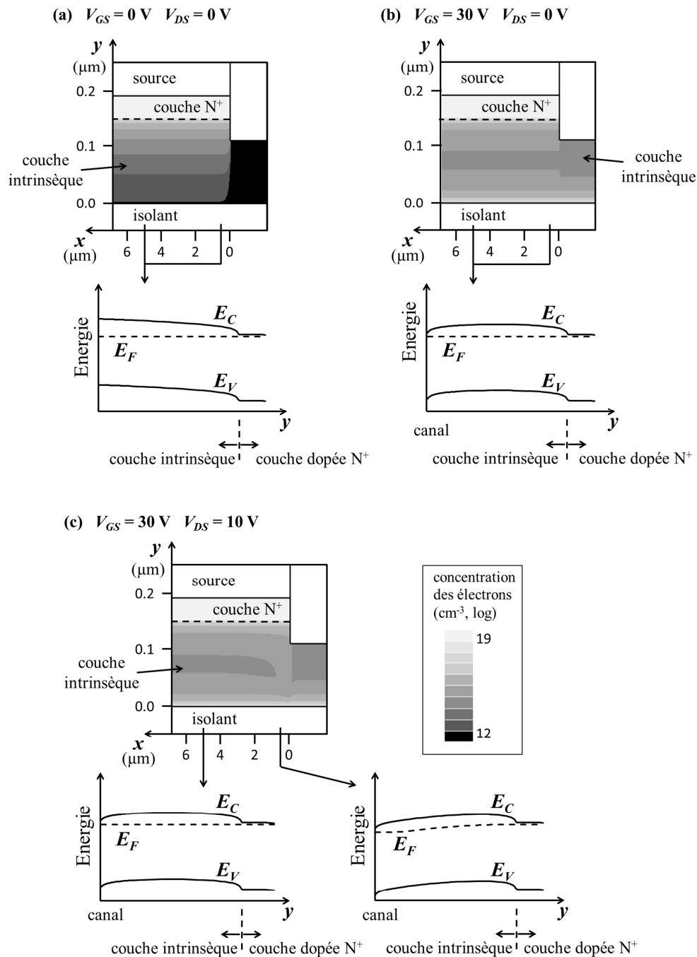
Figure 3.3-2 Concentration des électrons ( \text{cm}^{-3} , échelle logarithmique) près de la source quand (a) V_{GS} = V_{DS} = 0 \text{ V} , (b) V_{GS} = 30 \text{ V} et V_{DS} = 0 \text{ V} , et (c) V_{GS} = 30 \text{ V} et V_{DS} = 10 \text{ V} , avec le profil de la bande d'énergie en direction y aux positions x = 0,5 \mu\text{m} et x = 5 \mu\text{m} . E_C dénote l'énergie de conduction, E_V celle de valence, et E_F le quasi-niveau de Fermi des électrons.
