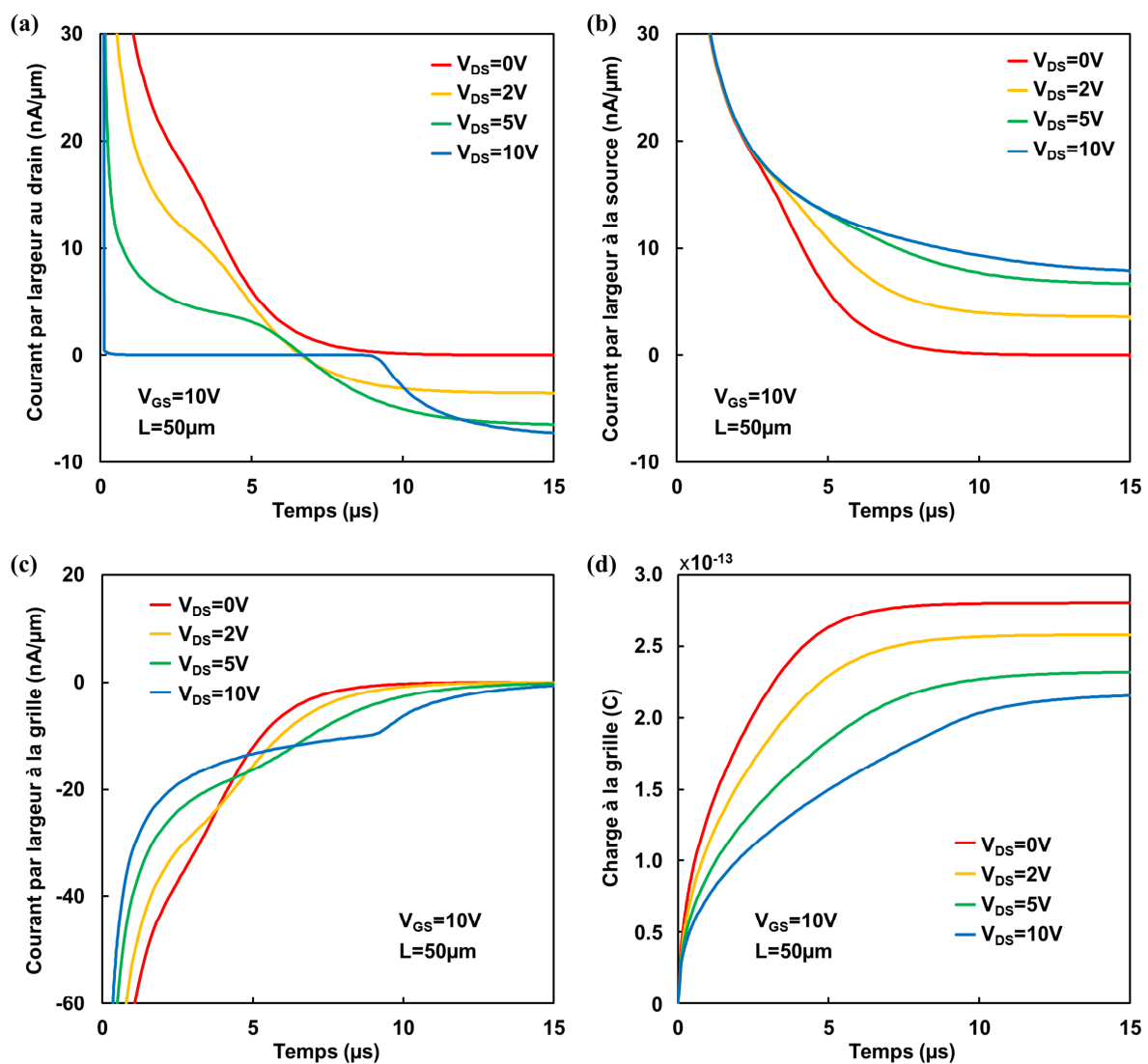
Figure 4.3-2 Simulation ATLAS du courant de transition de l'état éteint ( V_{GS} = 0\text{ V} ) à l'état allumé ( V_{GS} = 10\text{ V} ), (a) au drain, (b) à la source et (c) à la grille, pour plusieurs valeurs de V_{DS} . La figure (d) montre l'évolution temporelle de la charge stockée à la grille.
