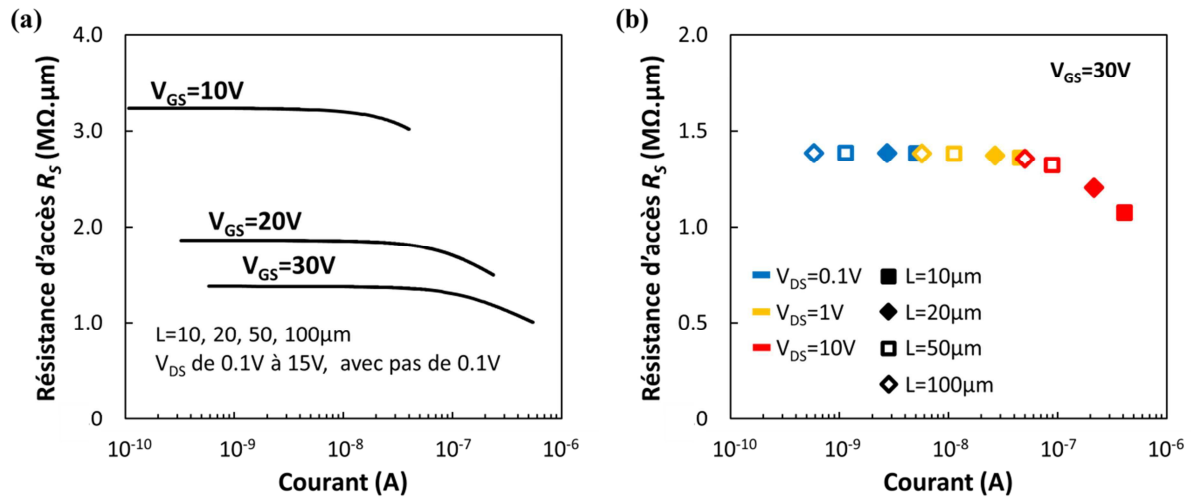
Figure 3.3-6 Résistance d'accès à la source ( R_S ) en fonction du courant : (a) représentation de tous les points obtenus en faisant varier V_{DS} et L , pour trois valeurs de V_{GS} (10, 20 et 30V) ; (b) quelques points sous V_{GS} = 30V , montrant que ces points se résument à une seule courbe.
