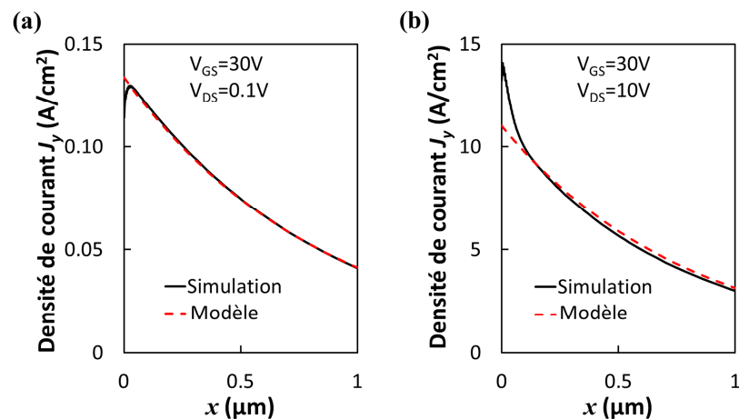
Figure 3.3-10 La comparaison entre la simulation et le modèle de la densité de courant en direction y , (a) quand V_{DS} = 0,1V et (b) quand V_{DS} = 10V .
