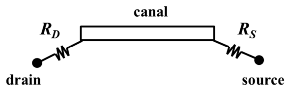
Figure 3.1-1 Résistance d'accès en série avec le canal
