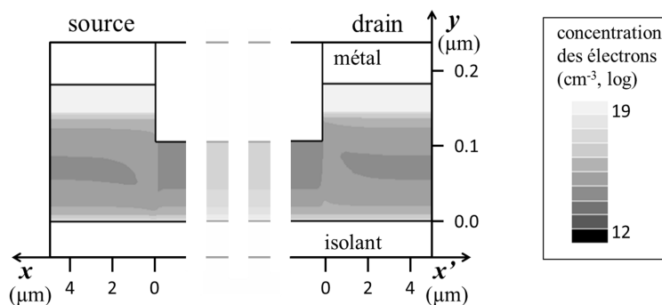
Figure 3.3-7 Concentration des électrons ( cm^{-3} , échelle logarithmique) près de la source et près du drain quand V_{GS} = 30V , V_{GD} = 20V et V_{DS} = 10V .
