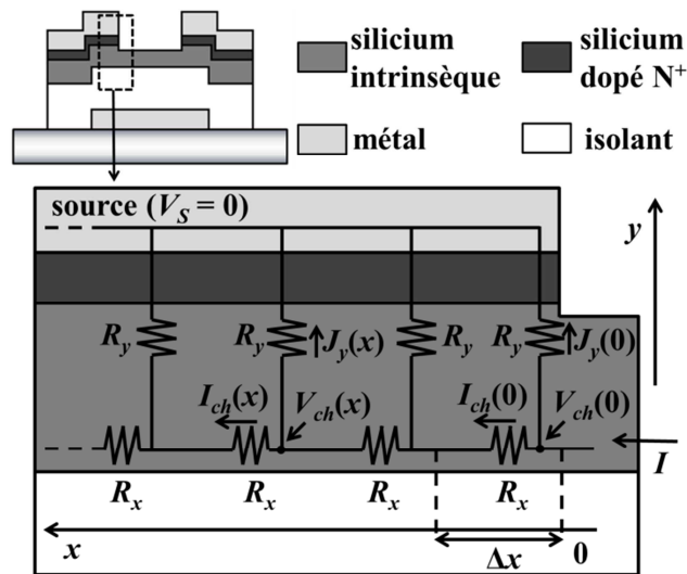
Figure 3.3-1 Circuit équivalent près de la source d'un TFT avec la structure bottom-gate staggered .
