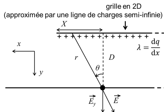
Figure 3.2-5 Schéma de l'effet au bord dans la structure TGC.
