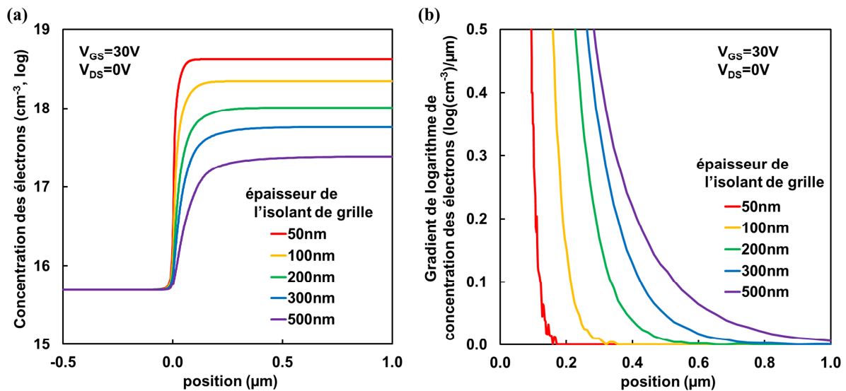
Figure 3.2-8 (a) Simulation ATLAS de la concentration des électrons induits par la tension de grille dans la structure TGC avec des différentes épaisseurs de l'isolant de grille et (b) son gradient.
