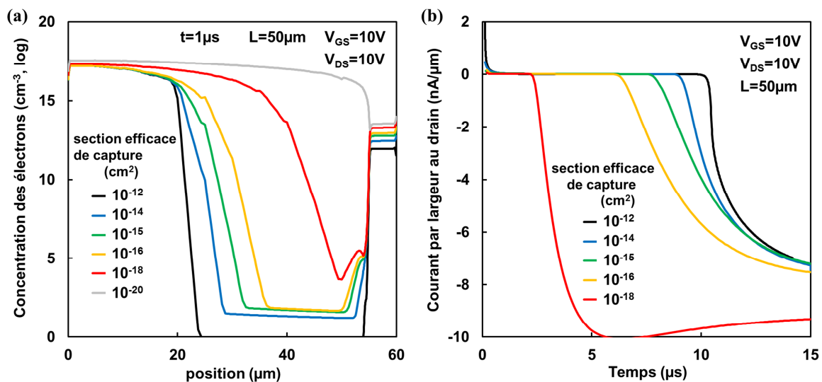
Figure 4.5-12 Simulation ATLAS de la transition de l'état éteint ( V_{GS} = 0\text{V} ) à l'état allumé ( V_{GS} = 10\text{V} ) en mode saturé ( V_{DS} = 10\text{V} ), en faisant varier la section efficace de capture : (a) la concentration des électrons dans le canal (lue à 1nm de distance à partir de l'interface avec l'isolant de grille) à l'instant t = 1\mu\text{s} , (b) le courant au drain en fonction du temps.
