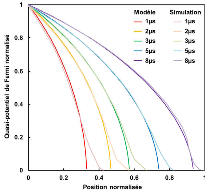
Figure 4.5-5 Simulation de la distribution du quasi-potentiel de Fermi à plusieurs instants d'un TFT à base de silicium avec des défauts et la distribution prévue par notre modèle (avec \gamma = 0,79 ).
