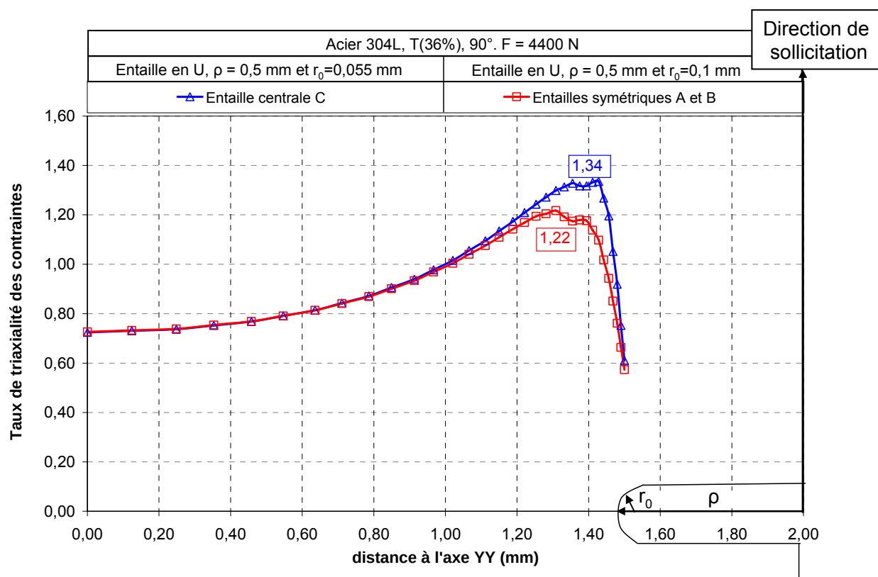
Figure A.3-2 : Profil du taux de triaxialité en fond d'entaille pour l'acier 304L T(36%), 90° sous une force appliquée de 4400 N
