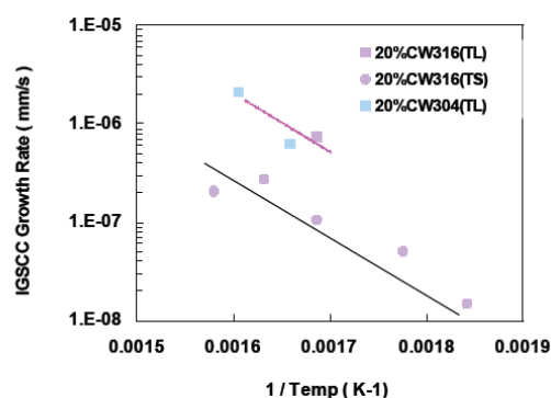
Figure 2-39 : Evolution de la vitesse de propagation intergranulaire en milieu primaire de REP en fonction de la température. Aciers 304 et 316 écrouis par laminage L(20%). Essais sous charge constante K = 30 MPa.m (Arioka 2007)
