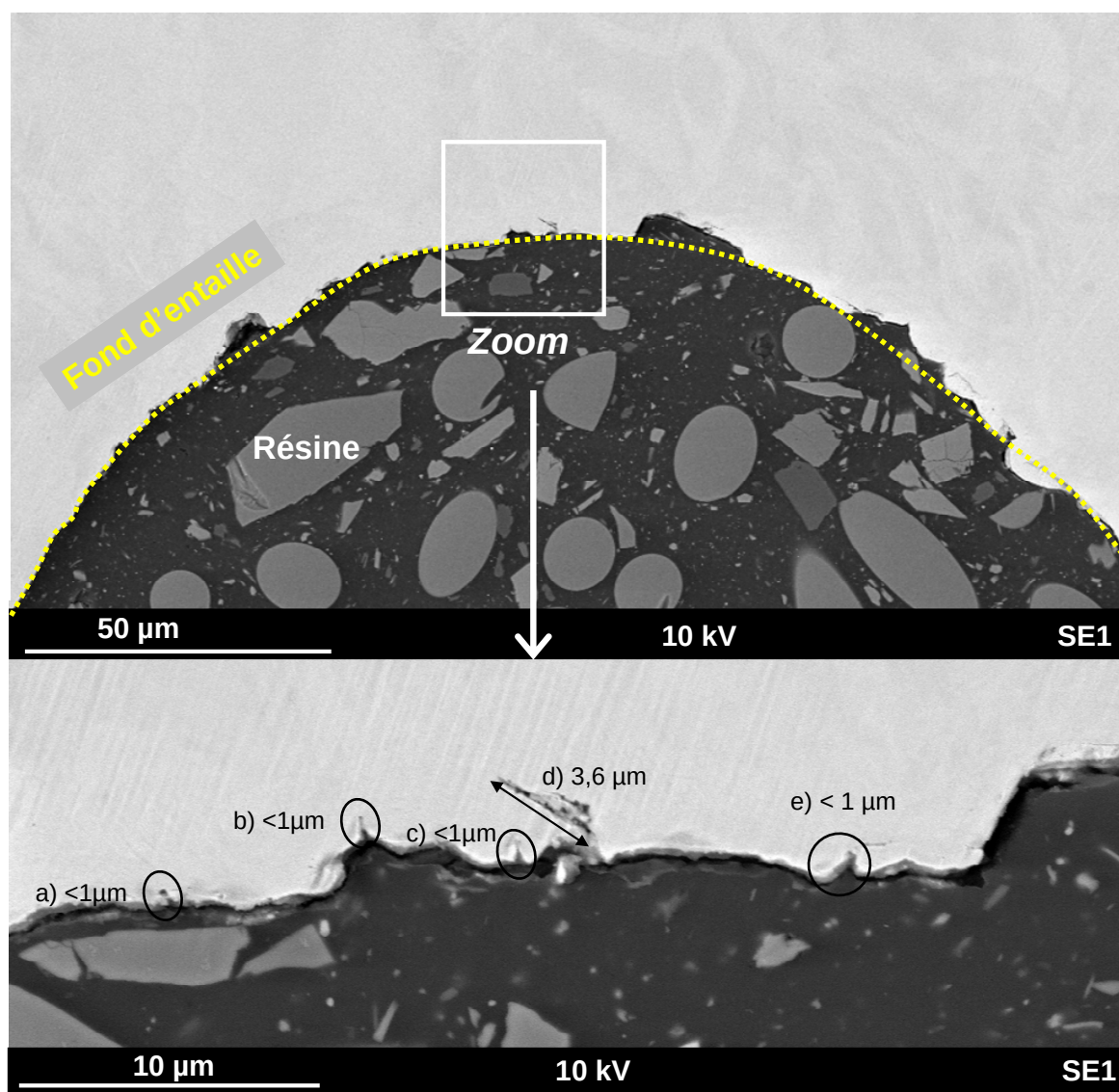
Figure 4-20 : Observations MEB d'un fond d'entaille en U (électro-érosion, pas de passage de fil) après essai de CSC. Détail du fond d'entaille : nombreux défauts. Absence de fissuration avérée
