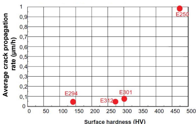
Figure 2-46 : Evolution de la vitesse moyenne de propagation des fissures de CSC selon la dureté initiale en surface - Acier 304L éroui par grenaillage, essai de traction lente 1,5 \cdot 10^{-7} \text{s}^{-1} , 360°C (Raquet 2005)
