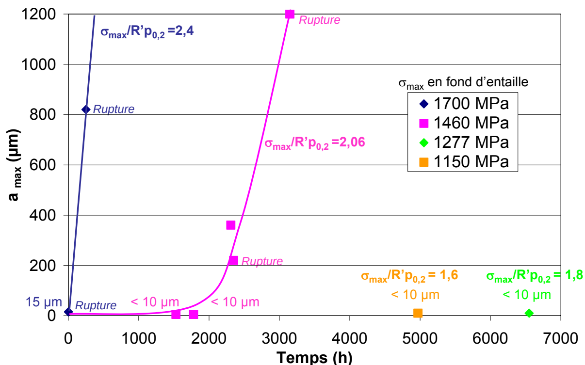
Figure 2-64 : Profondeur maximale de fissuration a_{\max} obtenue après essais d'amorçage de la CSC sur éprouvettes entaillées. Acier 316L L(40%), chargement trapèze. R = 0,85 , f = 3.10^{-4} Hz, 340^{\circ}\text{C} (Herms 2011a)
