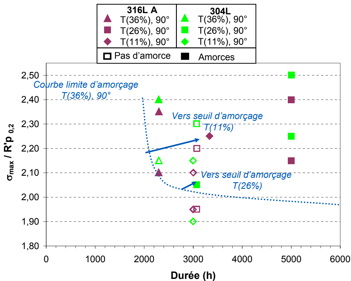
Figure 5-34 : Domaine d'amorçage à 360°C dans l'espace chargement relatif / durée en fonction de la pré-déformation
