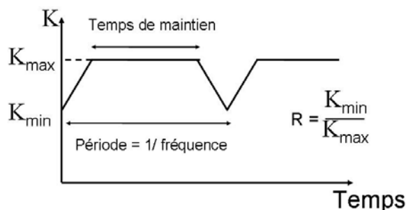
Figure 2-26 : Description d'un chargement cyclique de forme trapèze
