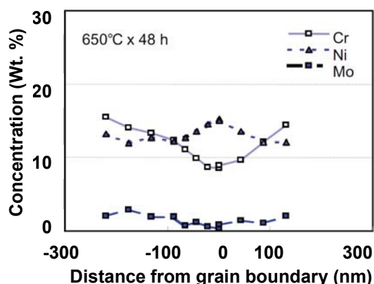
Figure 2-41 : Evolution de la teneur massique en Cr, Ni, et Mo autour d'un joint de grains (Arioka 2005)
