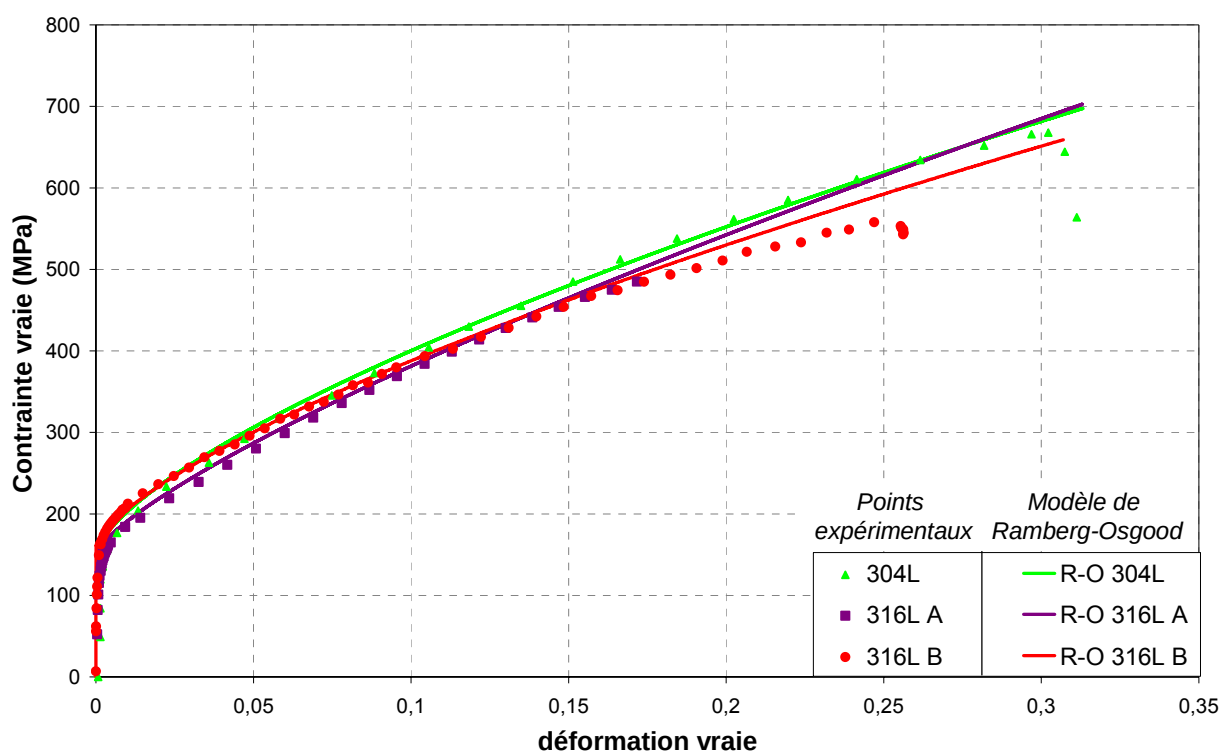
Figure 3-6 : Courbes simulées obtenues à l'aide d'un modèle de Ramberg-Osgood (R-O) à 360°C des aciers 304L, 316L A et B - Etat hypere trempé
