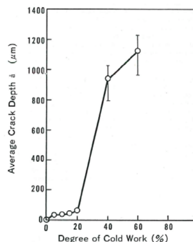
Figure 2-21 : Influence de l'écrouissage sur la sensibilité à la CSC d'un acier 304L ( Md_{30} = 7^\circ\text{C} ), essais CBB pendant 500 h, 8 ppm d'oxygène dissous (Kuniya 1988)
