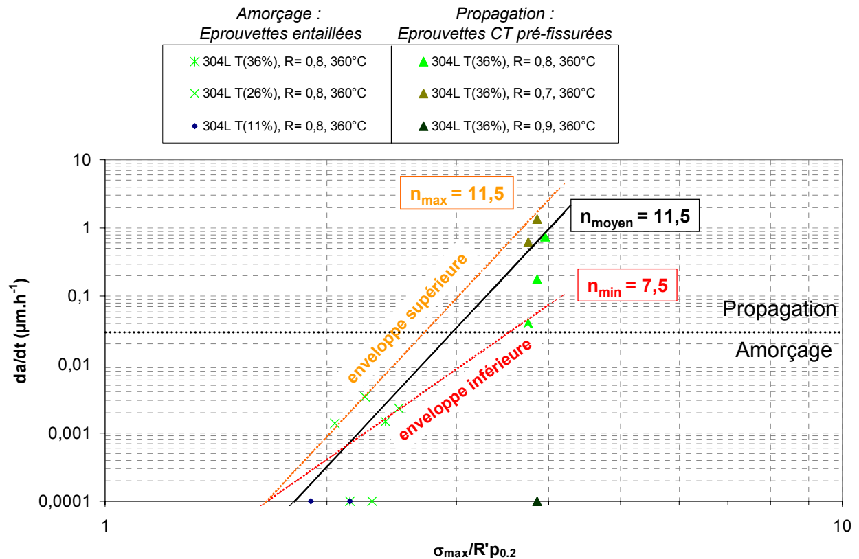
Figure 6-43 : Effet du chargement sur les cinétiques de propagation lente et de propagation rapide. Acier 304 L. Les vitesses de propagation nulles ont été décalées à 0,0001 \mu\text{m.h}^{-1}
