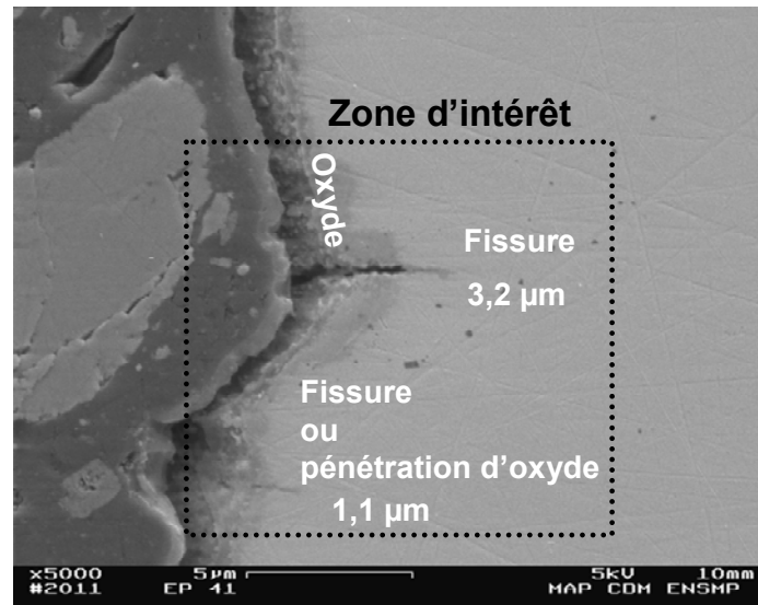
Figure 5-6 : Amorces présentes dans la zone de prélèvement de la lame mince. Epreuve 1510TE7, entaille B, acier 304L, T(26%), 5000 h, \sigma_{\max}/R'p_{0.2} , 360°C = 2,25
