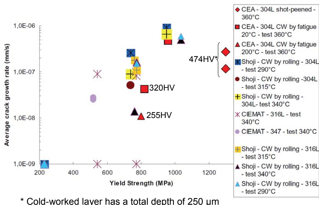
Figure 2-45 : Compilation de résultats de propagation par CSC des aciers inoxydables du CEA (Raquet 2005) avec Castano (Castano 2003) et Shoji (Shoji 2003)
