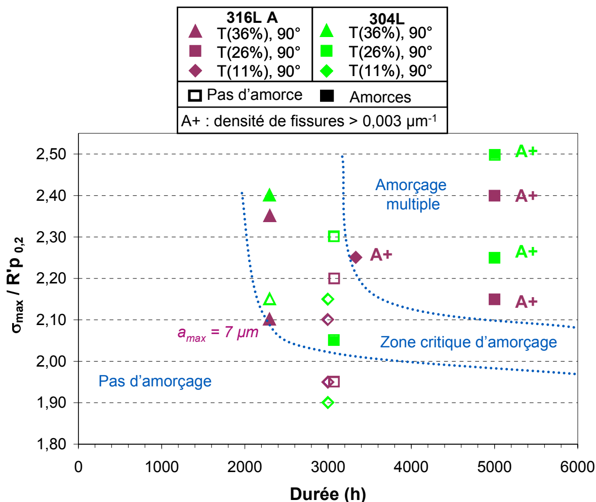
Figure 5-35 : Courbe limite d'amorçage et d'amorçage multiple à 360°C. Analyse en densité linéique
