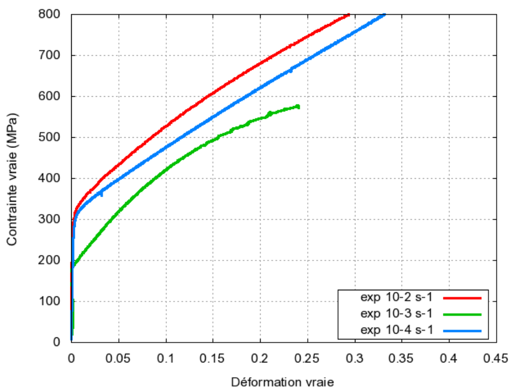
Figure 3-20 : Effet de la vitesse de déformation à l'ambiante sur l'acier 316L A à l'état de réception. Base expérimentale
