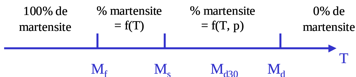
Figure 2-4 : Stades de la transformation martensitique en fonction de la température T et de la déformation plastique p
