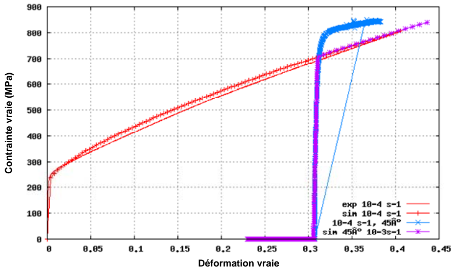
Figure A.2-8 : Comparaison des courbes contrainte-déformation expérimentales et simulées avec écroutissage cinématique, 45°, acier 304L
