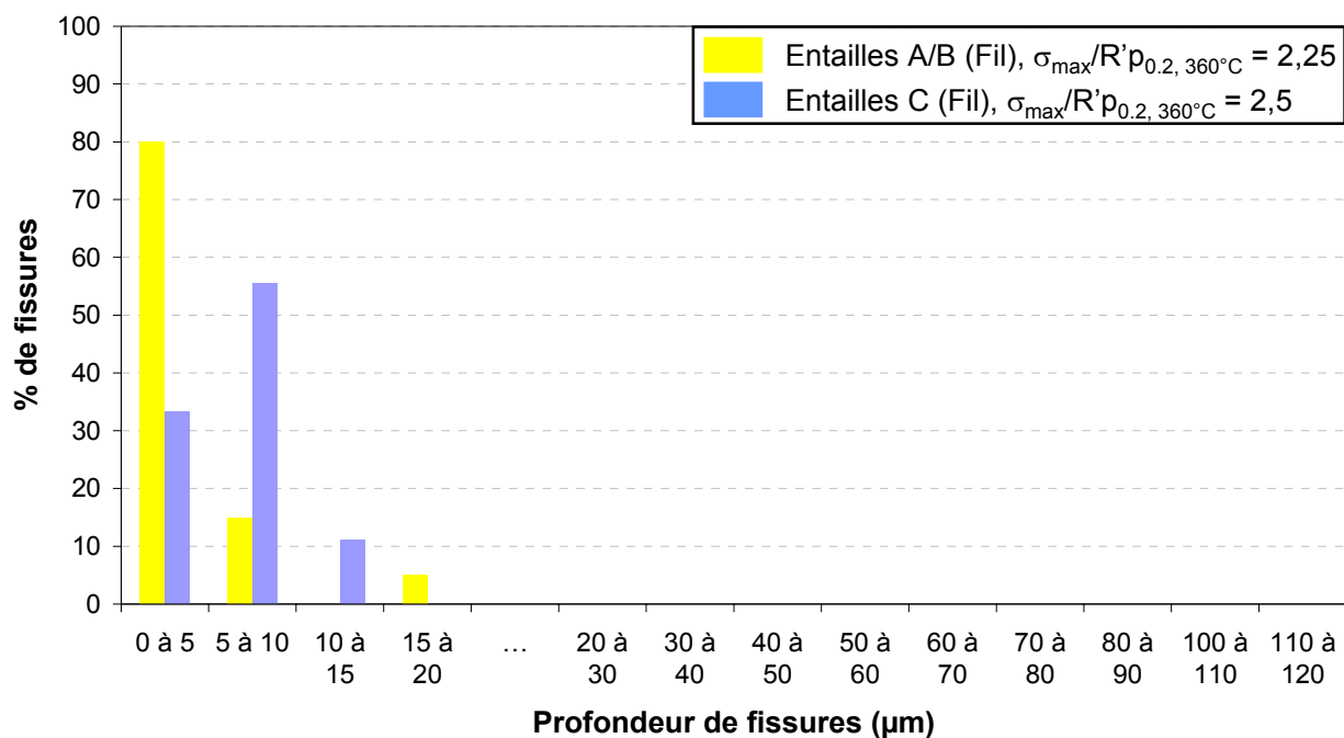
Figure 5-33 : Histogramme des profondeurs de fissures observées sur coupe métallographique. Epruvettes 1510TE7 et 25, acier 304L, T(26%), 90°, 5000 h
