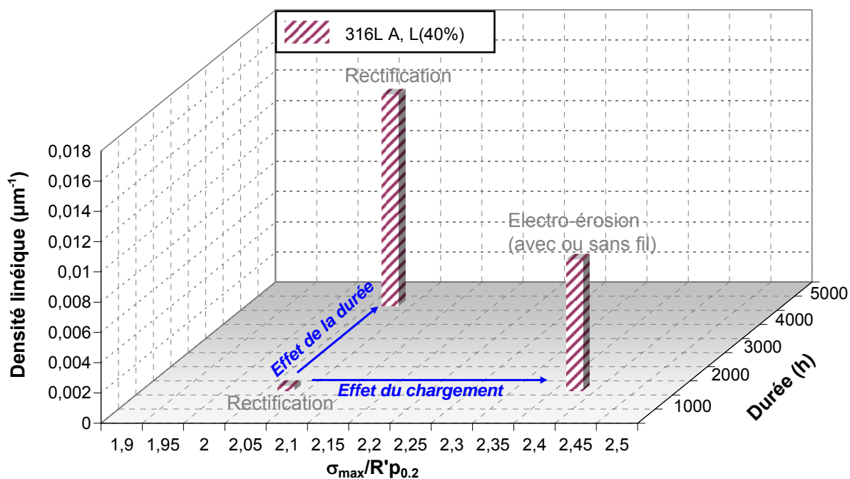
Figure 5-46 : Effet du chargement et de la durée sur la densité linéique des amorces. Acier 316L A, L(40%)
