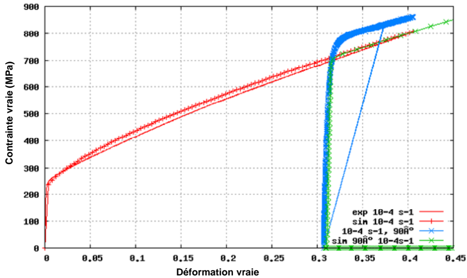
Figure A.2-7 : Comparaison des courbes contrainte-déformation expérimentales et simulées avec écroutissage cinématique, 90°, acier 304L
