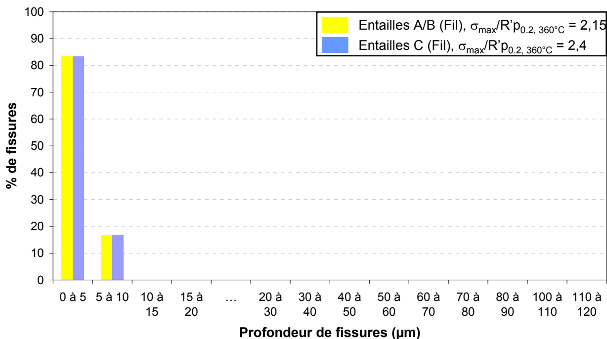
Figure 5-32 : Histogramme des profondeurs de fissures observées sur coupe métallographique. Epruvettes 1510TT7 et 25, acier 316L A, T(26%), 90°, 5000 h
