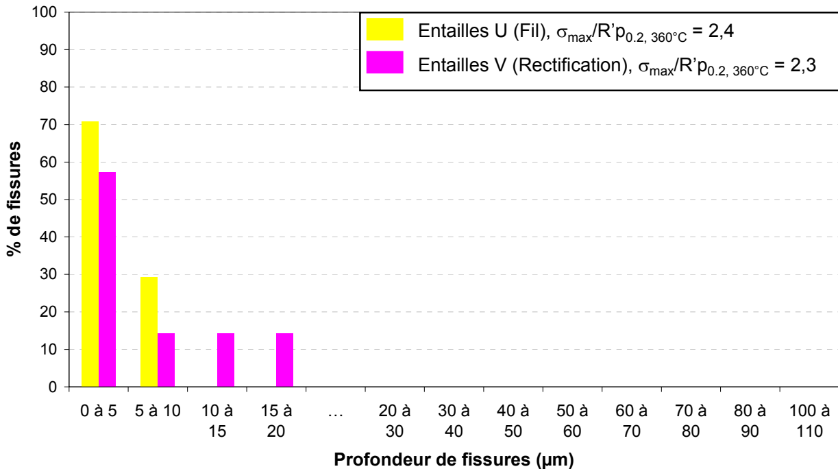
Figure 5-57 : Distribution des profondeurs de fissures observées sur coupe métallographique. Eprouvette 1617T36T3-4, acier 316L A, T(36%), 3000 h
