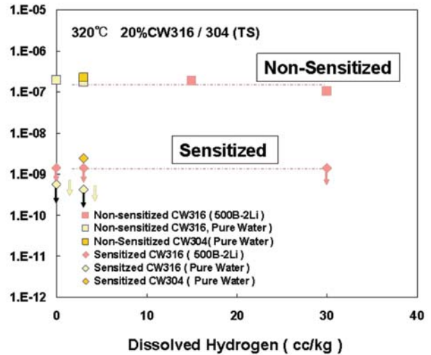
b) Essais sous charge constante K= 30 MPa.\sqrt{m} Aciers 304 et 316 sensibilisés ou non écrouis par laminage L(20%), 320°C (Arioka 2005)
