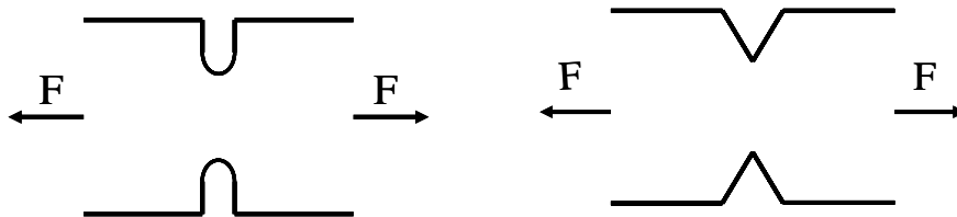
Figure 4-3 : Formes des entailles (U ou V) des éprouvettes TRC
