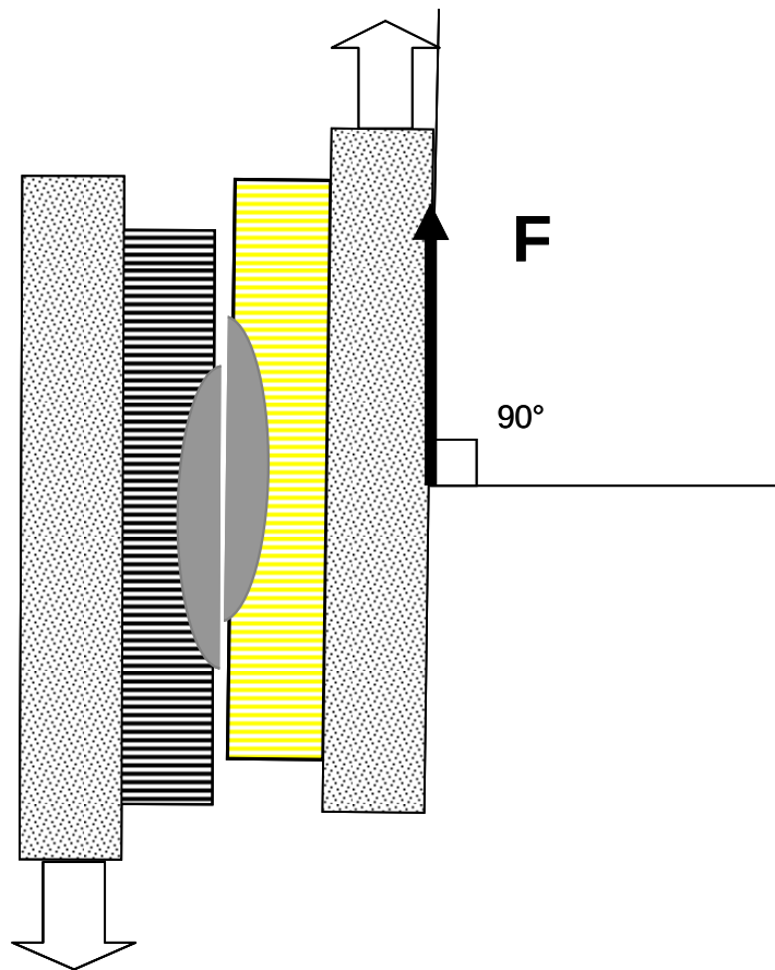
Figure 5-21. Représentation schématique de l'essai de cisaillement (30°).
