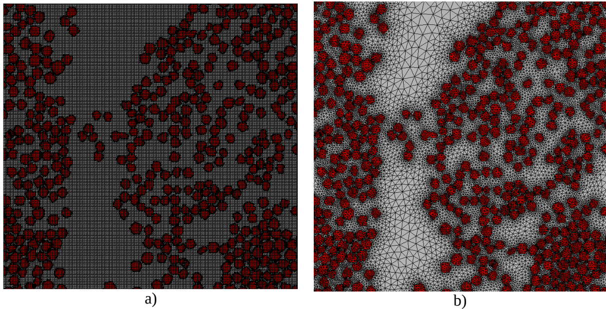
Figure 3-17. Maillages de la microstructure pour les calculs par éléments finis.
