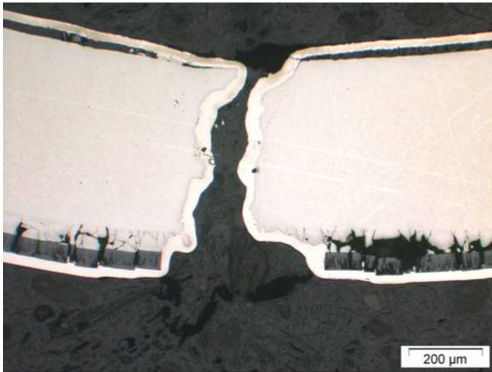
Figure 4-19 : Fissure de l'ex-β de la gaine 6_1100_A_2 rompue à \epsilon_{00}=0,072 .
