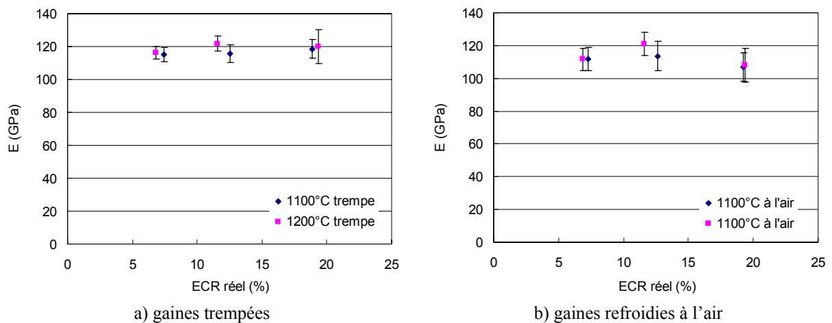
Figure 2-24 : Evolution du module d'Young E de la matrice de la couche ex- \beta en fonction de l'ECR réel.
