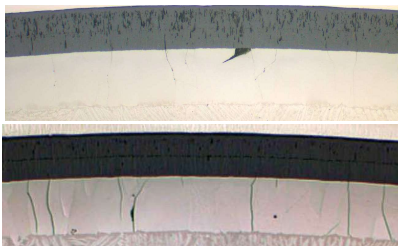
Figure 4-22 : Couches \alpha(O) et ZrO_2 de la gaine 10_1200_A_F après l'essai EDC.
