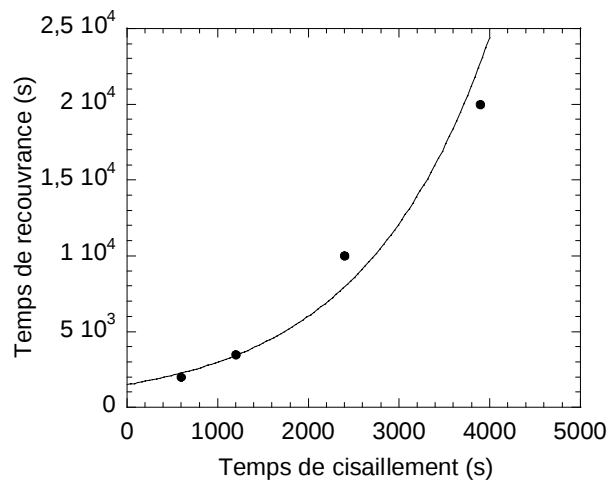
Fig. 4.26. Temps de recouvrement des modules pour la fréquence de 10 rad/s en fonction du temps de cisaillement pour un taux de cisaillement de 0,16 \text{ s}^{-1}
