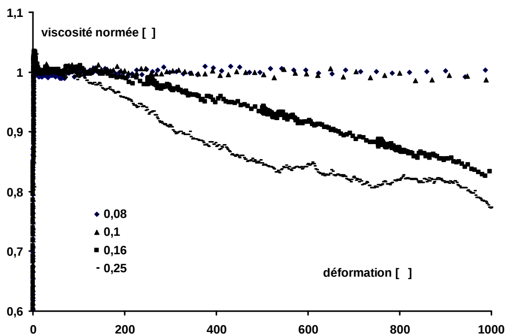
Fig. 4.13. Evolution de la viscosité normée \eta(t)/\eta_0 en fonction de la déformation (Polymère B, \diamond 0,08 s^{-1} ; \blacktriangle 0,1 s^{-1} ; \blacksquare 0,16 s^{-1} et \blacktriangle 0,25 s^{-1} , 160°C)
