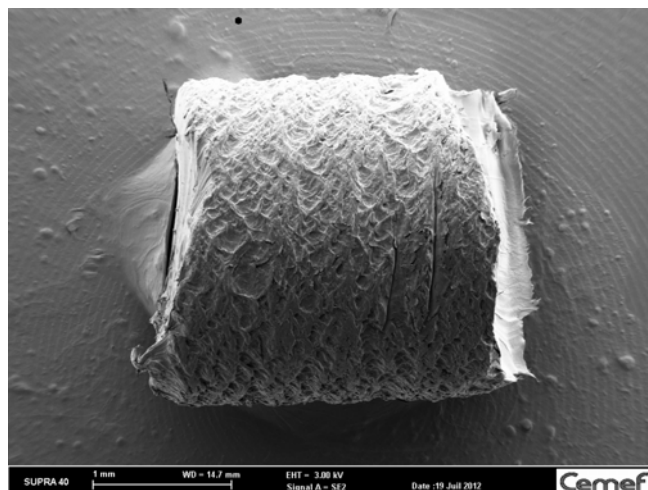
Figure 5.8. Aspect de l'extrudats pré-cisaillés pendant 7200 s à 2,5 tr/min (Polymère D, 160°C)
