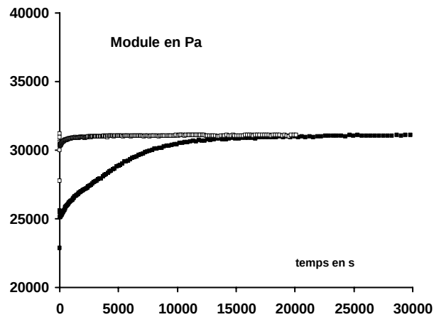
Fig. 4.25. Temps de recouvrement du module visqueux pour la fréquence de 10 rad/s pour le taux de cisaillement de 0,16 \text{ s}^{-1} pendant deux temps, 600 ( \square ) et 3900 s ( \blacksquare )
