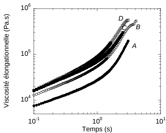
Figure 3.30. Viscosité élongationnelle en fonction du temps pour les quatre polymères à 1 \text{ s}^{-1} (140°C)
