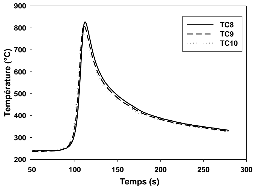
Figure 3-48 : cycles thermiques relevés par les thermocouples, pour des températures maximales inférieures à Ac_{1f} .
