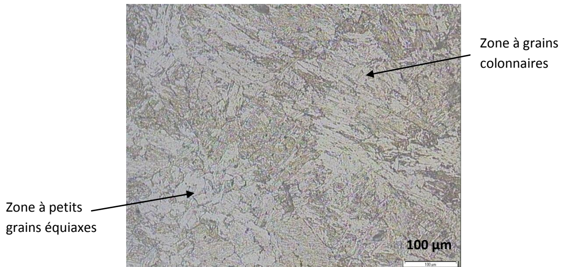
Figure 3-69 : micrographie optique de la zone fondue. Transition entre zones à grains colonnaires et équiaux (Attaque Villela).
