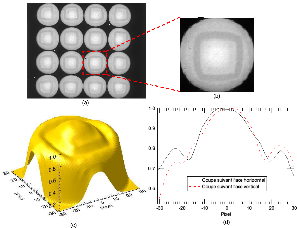
FIGURE 5.10 – (a) Image brute d'un corps noir plan à la température de 20 °C, placé contre le hublot de la caméra, sans correction des pixels morts, (b) Extraction de l'imagette correspondant à la voie 11, corrigée des pixels morts et de taille 62 \times 62 pixels, (c) Image 3D normalisée du fond uniforme acquis par la voie 11, (d) Coupes suivant les axes horizontal et vertical de l'imagette.
