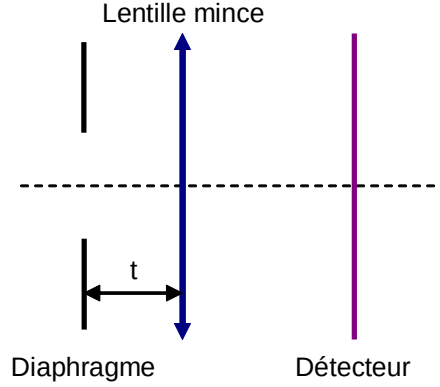
FIGURE 1.5 – Illustration d'un système simple composé d'une lentille mince, d'un diaphragme (qui est la pupille d'entrée) et d'un détecteur, t est la distance entre la pupille d'entrée et la lentille.
