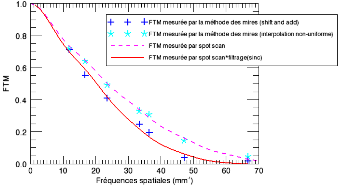
FIGURE 5.16 – Courbes de FTM sur l’axe optique de la caméra sur puce associée aux deux algorithmes de dépliement de spectre, de type shift and add d’une part et par interpolation non-uniforme d’autre part. Nous avons comparé les mesures effectuées par la méthode des mire, par spot scan , et par spot scan multiplié par un terme de filtrage en sinus cardinal.
