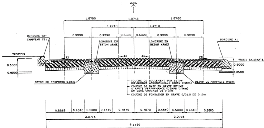
Figure 47: Coupe type du TVR de Caen (Source : l'AOT de Caen)
