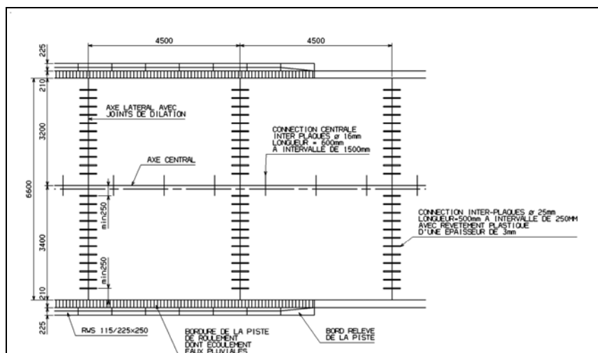
Figure 62: Implantation des plots magnétiques de la voie du PHILEAS sur un ouvrage en BA (Source : APTS)
