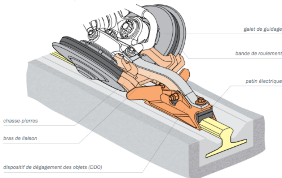
Figure 43: Détail du guidage du Translohr (Source : Lohr-Industrie)
