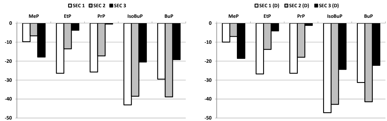
A. Abatement sur la base des concentrations totales (D+P) B. Abatement pour la phase dissoute (D)
