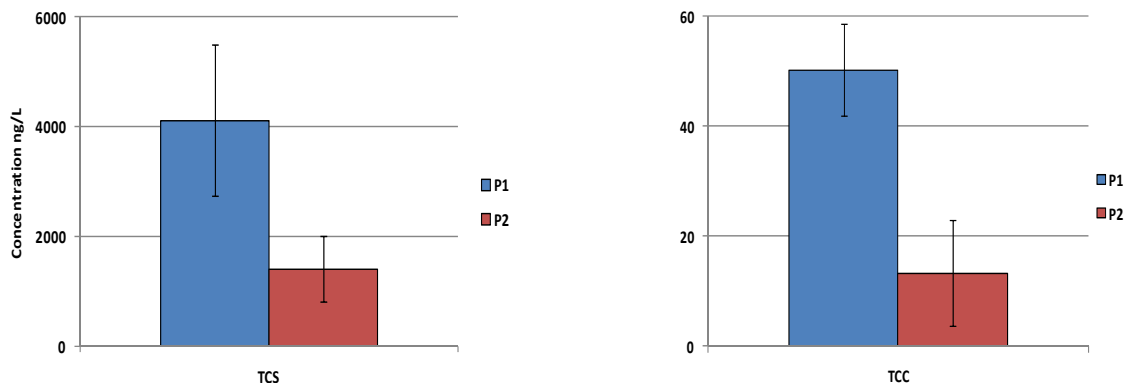
Figure 63 : Concentration (ng/L) du TCS et du TCC (phase particulaire) en P1 et P2
