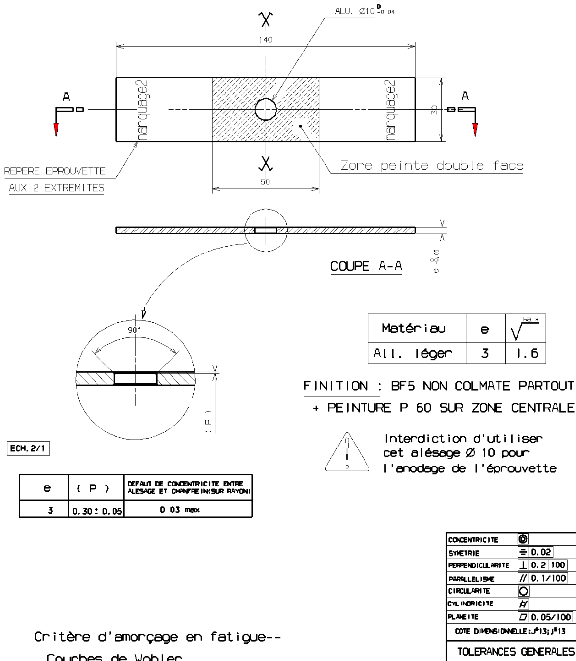
FIGURE 2.18 – Plan de définition des éprouvettes de fatigue trouées T10 (Kt=2,3)
