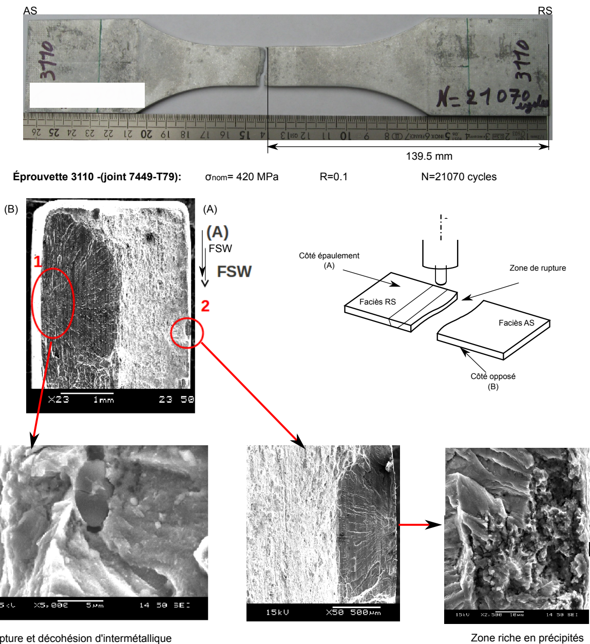
FIGURE 4.27 – Observations MEB du faciès de rupture d'un joint soudé par FSW en alliage 7449-T79
