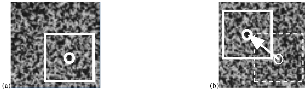
FIGURE 1.25 – Principe de calcul de déplacement ; (a) :Imagette de référence non déformée et (b) : Imagette déformée
