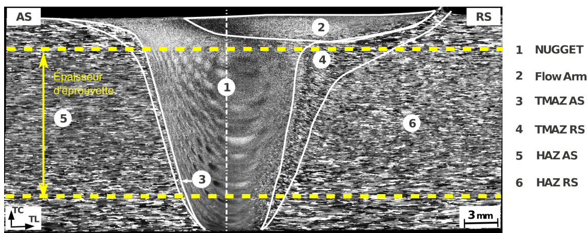
FIGURE 3.15 – Définition, à partir de la microstructure, des zones constituant les joints FSW dans l'épaisseur des éprouvettes de traction monotone quasi-statique
