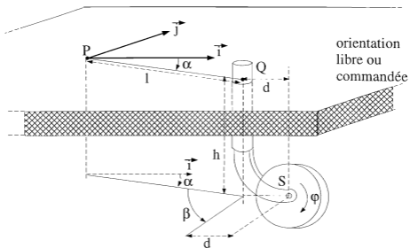
Figure 2.5: Roue désaxée
