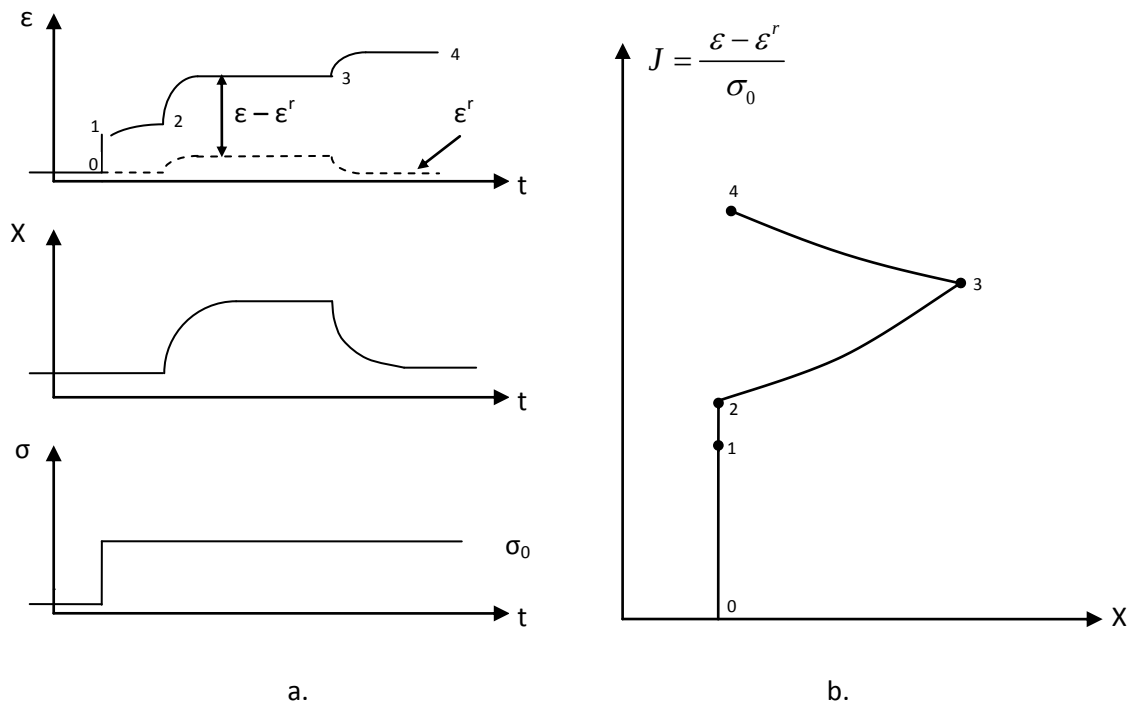
Figure 1.11. Construction d'une trajectoire mécanosorptive. a. Représentation temporelle : déformation totale ( \varepsilon ) et déformation liée au retrait ( \varepsilon^r ), taux d'humidité ( X ) et contrainte \sigma en fonction du temps ( t ). b. Trajectoire associée : complaisance J (déformation diminuée du retrait rapportée à la contrainte appliquée \sigma_0 ) en fonction du taux d'humidité X (d'après Gril, 1988).
