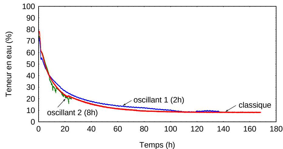
Cinétique de séchage – dosse 10 mm
