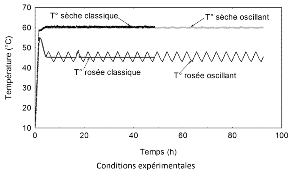
Figure D.2c. Conditions de séchage et cinétiques de séchage – campagne n°A.2. [Séchage classique : T° sèche = 60,3°C, X_{eq} = 7,0% ; séchage oscillant : T° sèche = 60°C, X_{eq} = 7,3%, \Delta X_{eq} = 1,8%, période = 4 heures].
