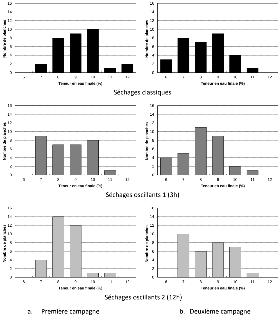
Figure 2.13. Distribution de la teneur en eau finale.
