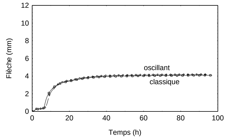
Flexion trois points – quartier (10mm)
