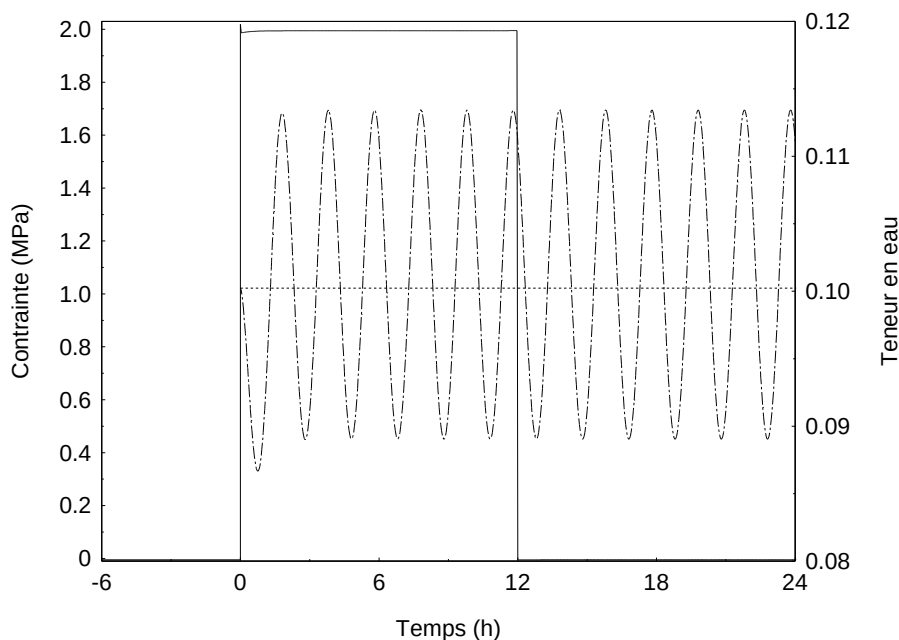
Figure 3.15. Conainte et teneur en eau fonction du temps [ \Delta X_{eq} 2,4%, période : 2h]
