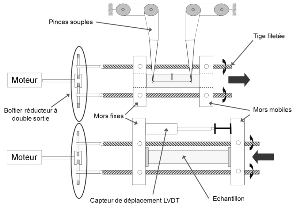
Figure G.3. Dispositif expérimentale pour mesurer la déformation à l'aide d'un capteur de contact type LVDT.
