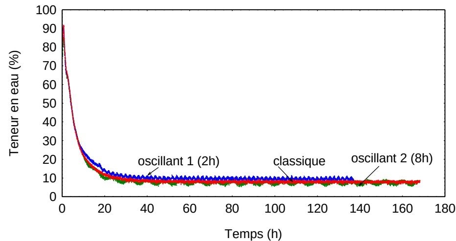
Cinétique de séchage – dosse 5 mm
