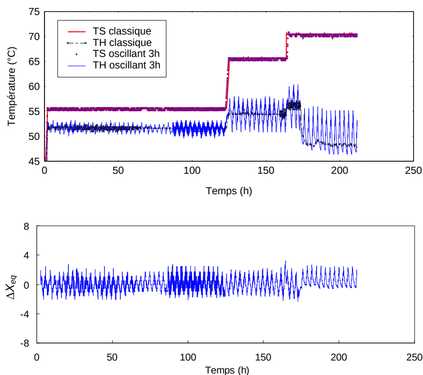
Figure 2.4. Tables des séchages classique et oscillant 1 (période de 3h) – campagne 2. En haut : température sèche et humide mesurées. En bas : Oscillation de X_{eq} calculée à partir de la température sèche et humide mesurées.
