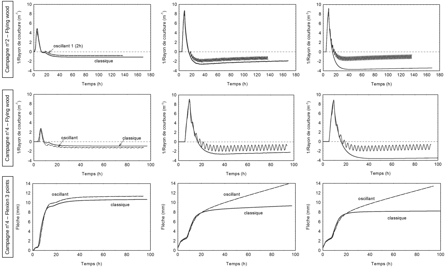
Figure b. Confrontation expérimentale – simulation avec m_s = 100 \text{ GPa}^{-1} , E_{ms} = 60 \text{ MPa} , \varepsilon_{ir} = 50 \text{ GPa}^{-1} . A gauche : résultats expérimentaux ; au centre : simulation (données climatiques expérimentales) ; à droite : simulation (données climatiques lissées).
