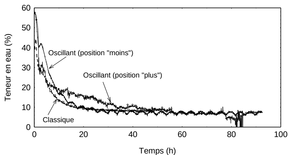
Cinétique de séchage – dosse 5 mm
