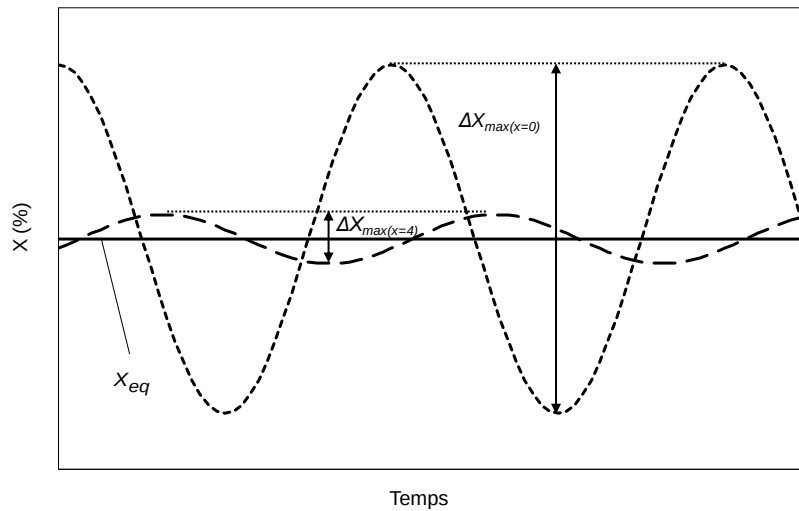
Figure 3.1. Schéma de l'évolution sinusoïdal de la teneur en eau pour x = 0 (surface) et x = 4 \text{ mm} .
