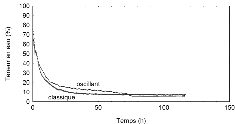
Cinétique de séchage – quartier
