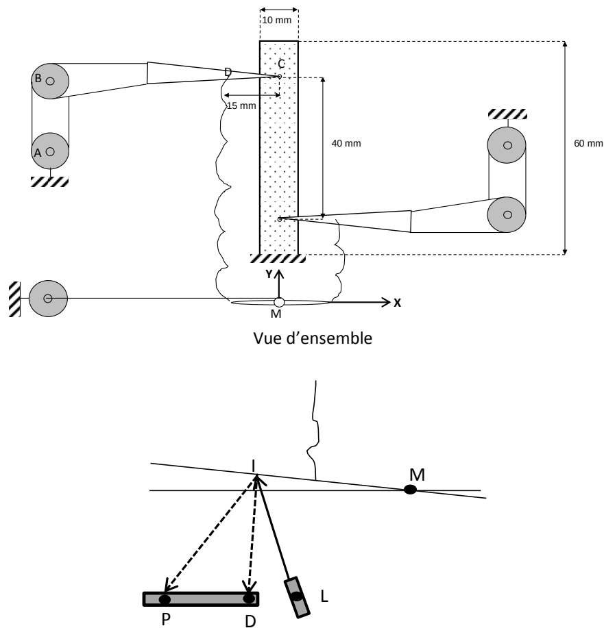
Rotation du miroir (M) et changement de position du rayon réfléchi dans le capteur numérique
