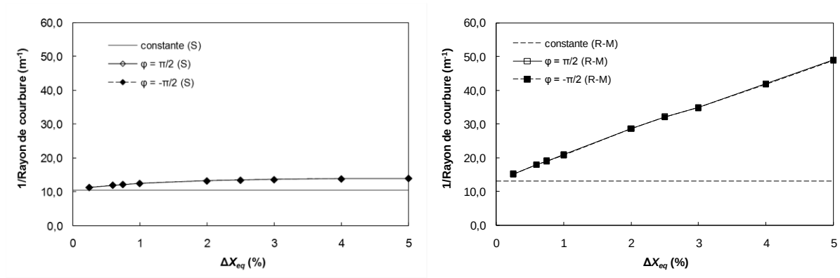
Figure B.15. Effet de l'amplitude dans le rayon de courbure finale en fonction du déphasage (angle \varphi ) selon le modèle de Salin (S) à gauche et de Ranta-Maunus (R-M) à droite. [Période : 3h]
