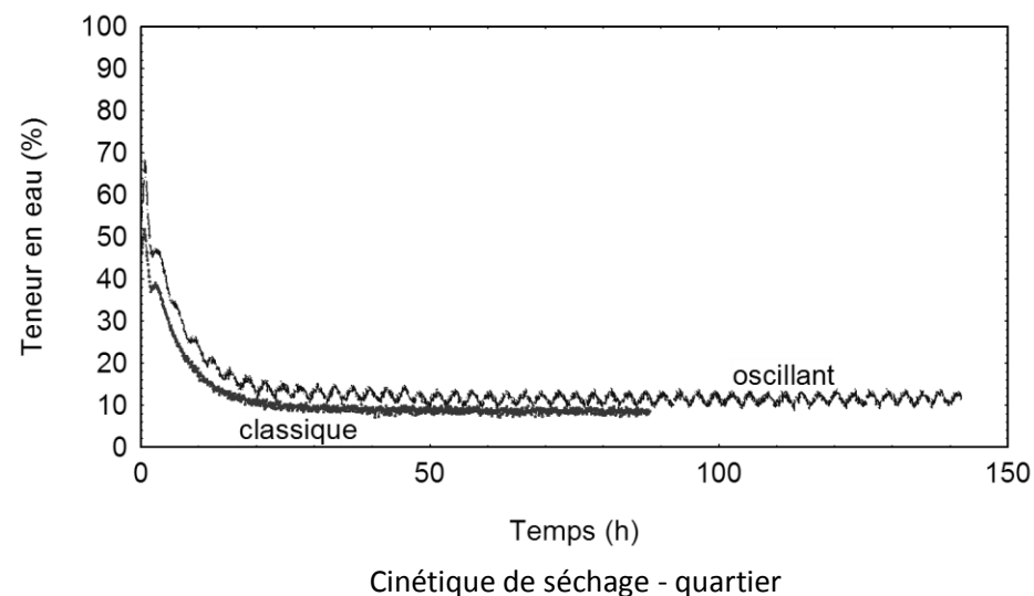
Figure D.1a. Conditions de séchage et cinétiques de séchage – campagne n°1. [Séchage classique : T° sèche = 59°C, X_{eq} = 8,8% ; séchage oscillant : T° sèche = 59°C, X_{eq} = 9,2%, \Delta X_{eq} = 3,2%, période = 3 heures].
