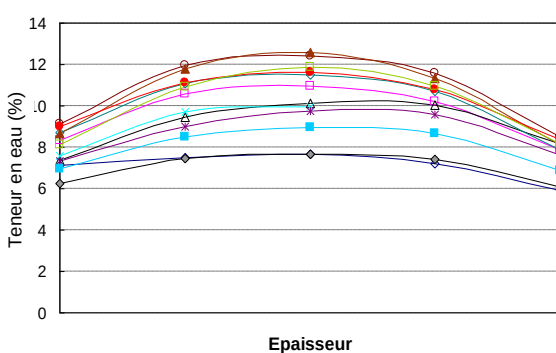
Séchages oscillants 2 (12h)
