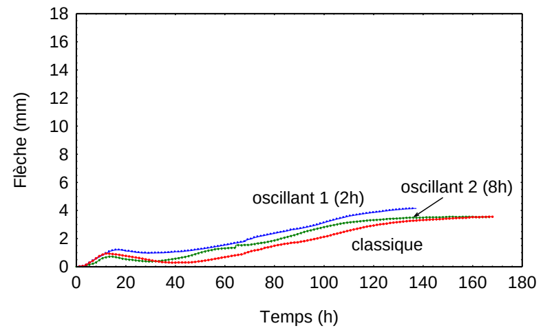
Poutre cantilever – dosse (20 mm)
