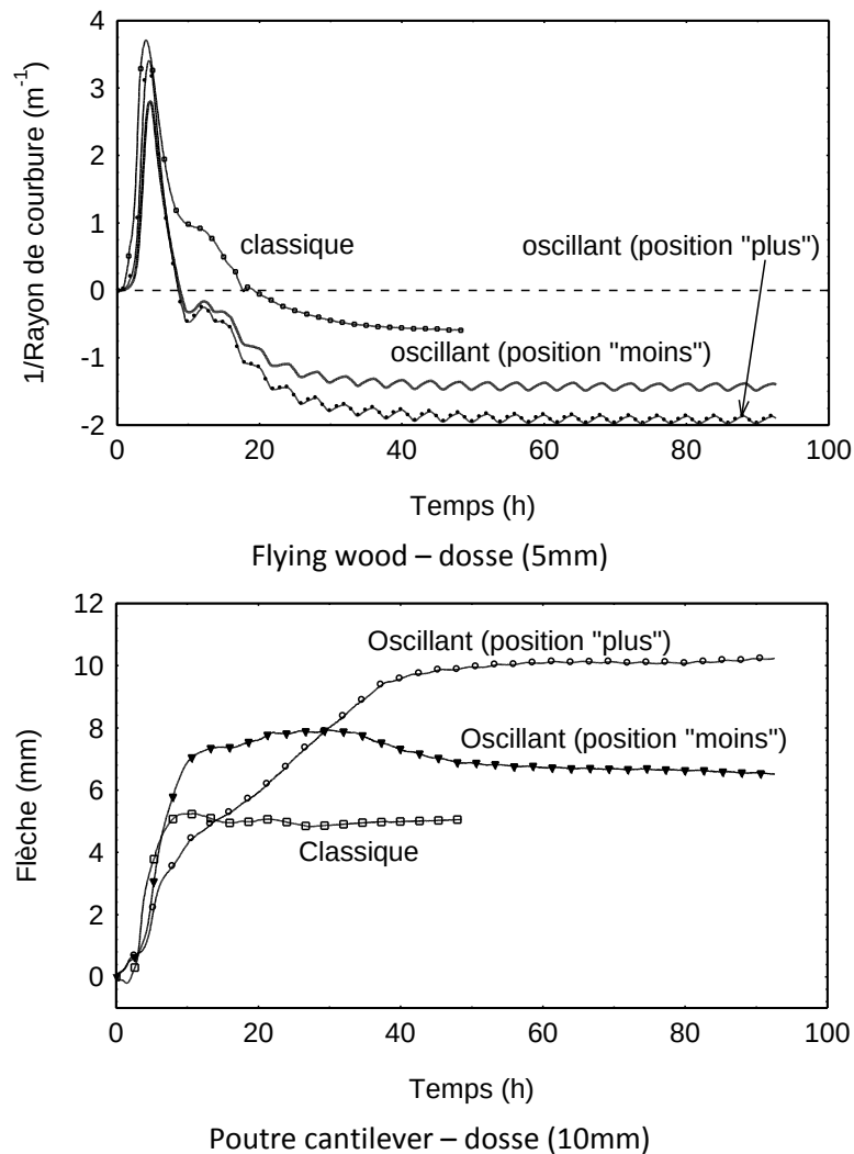
Figure D.3b. Réponse mécanique aux oscillations de la teneur en eau – effet de la courbure de cernes pour un échantillon sur dosse. [Séchage classique : T^\circ \text{ sèche} = 60,3^\circ\text{C} , X_{eq} = 7,0\% ; séchage oscillant : T^\circ \text{ sèche} = 60,1^\circ\text{C} , X_{eq} = 7,4\% , \Delta X_{eq} = 1,5\% , période = 4 heures].
