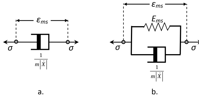
Figure 3.14. Modèle rhéologiques représentant la déformation mécanosorptive : a) Modèle de Ranta – Maunus ; b) Modèle de Salin.
