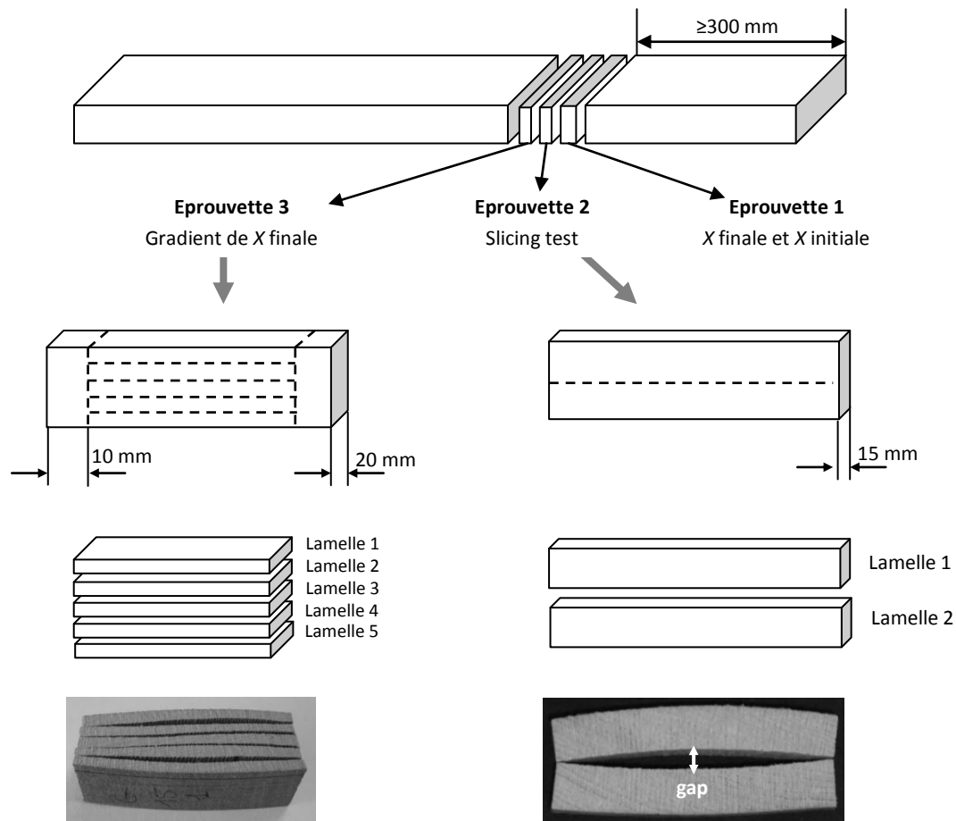
Figure 2.10. Plan de découpe à la fin du séchage pour la mesure des teneur en eau (X) finale et initiale, le slicing test et le gradient de teneur en eau finale. Les traits pointillés représentent les traits de coupe. En dessous, à gauche, lamelles pour le gradient après 24 heures dans l'étuve à 103°C ; à droite, lamelles pour le slicing test après 48 heures, on y aperçoit le gap.
