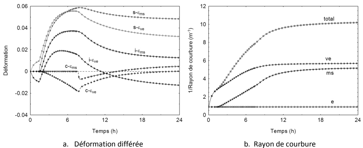
Figure B.11. Déformation mécanosorptive ( \epsilon_{ms} ) et viscoélastique ( \epsilon_{ve} ) à la surface supérieure (s), à la surface inférieure (i) et au cœur (c) et rayon de courbure.
