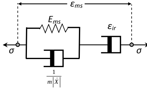
Figure E.1. Modèle de comportement mécanosorptif avec un élément de Kelvin (partie recouvrable) et un amortisseur (partie irréversible) en série.
