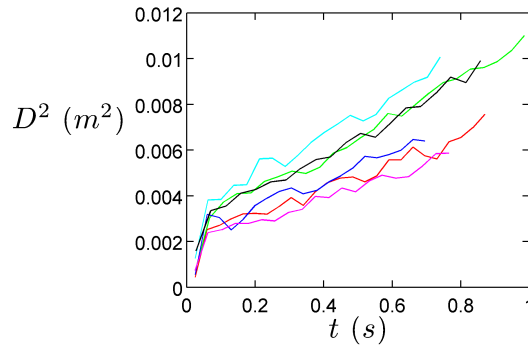
FIGURE 6.9 – Evolution du diamètre au carré de différentes bulles toroïdales entre leur formation et le contact avec la surface, le volume des bulles varie entre 5 et 15 cm 3 .
