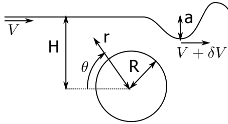
FIGURE 8.16 – Notations utilisées pour le modèle.
