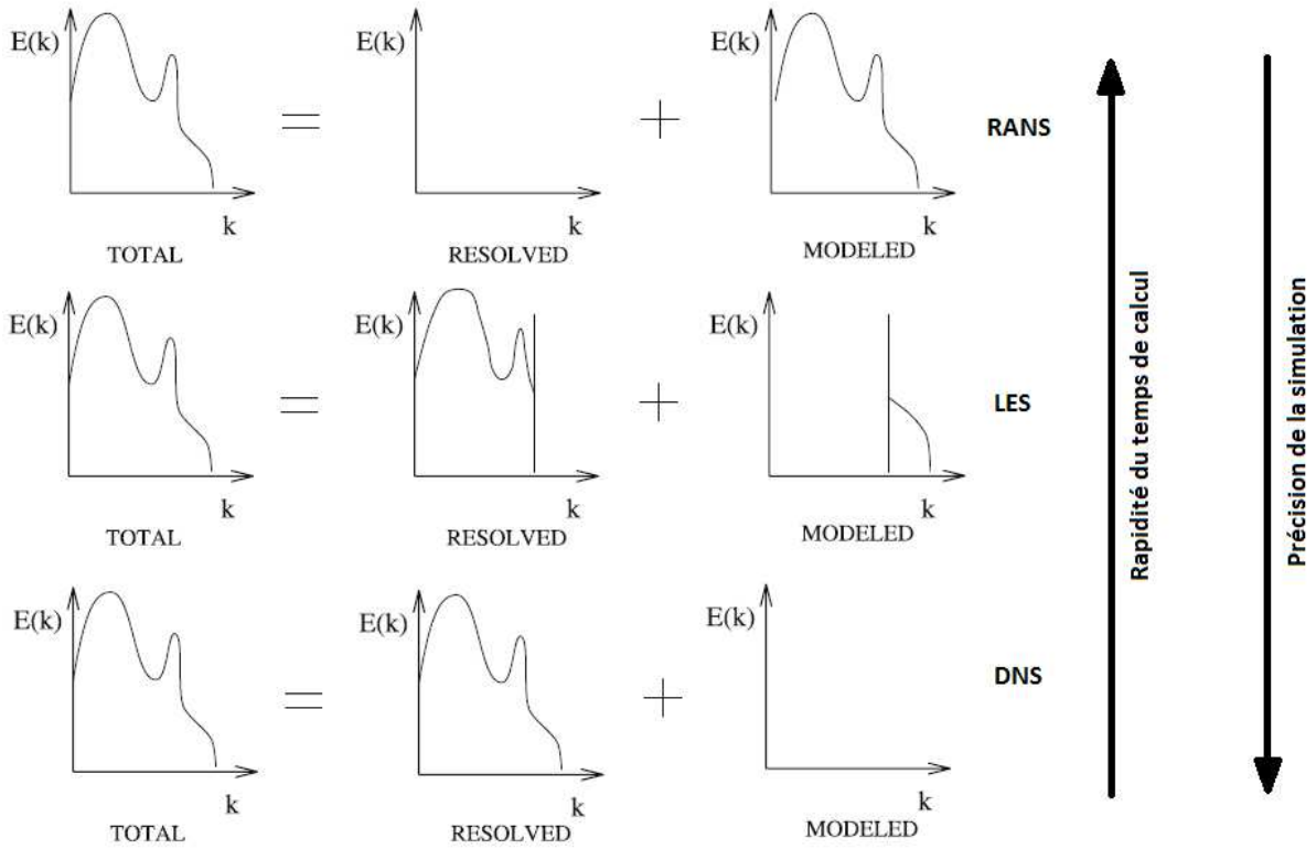
FIGURE 3.2 – Schématisation de la partie explicitement résolue et de la partie modélisée du spectre de l'énergie pour différent types de simulations : RANS, LES et DNS. De plus, est ajouté, pour chaque méthode, le rapport entre précision et temps de calcul [Sagaut, 2005].
