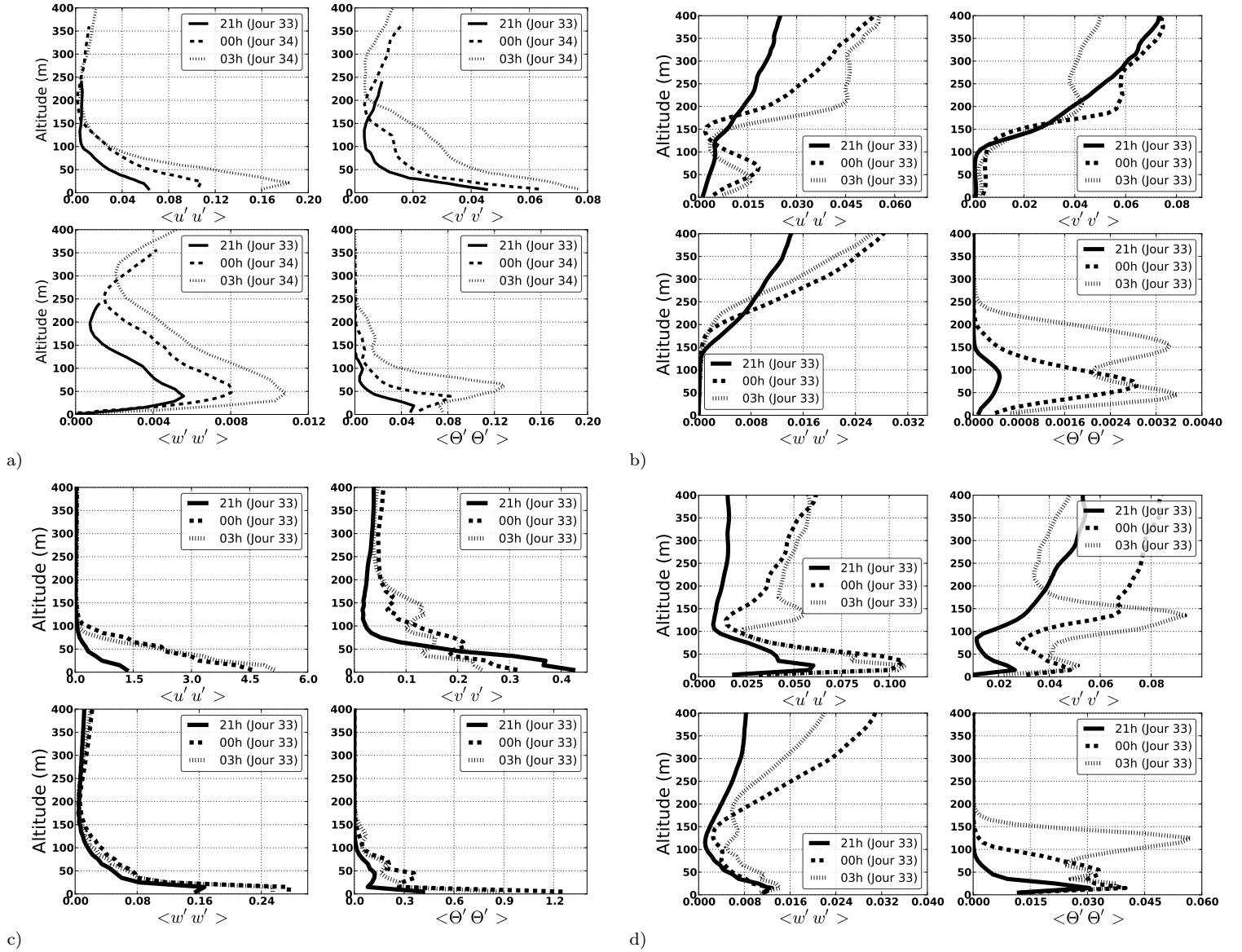
FIGURE 6.13 – Variances \overline{u'^2} , \overline{v'^2} , \overline{w'^2} et \overline{\Theta'^2} en fonction de l'altitude, la nuit, à 21h le jour 33, 00h et 03h le jour 34. Les résultats de (a) [Basu et al., 2008] avec le modèle sous-maille LASDD, (b) du modèle de Smagorinsky, (c) du modèle Germano-Lilly et (d) du modèle Wong-Lilly.
