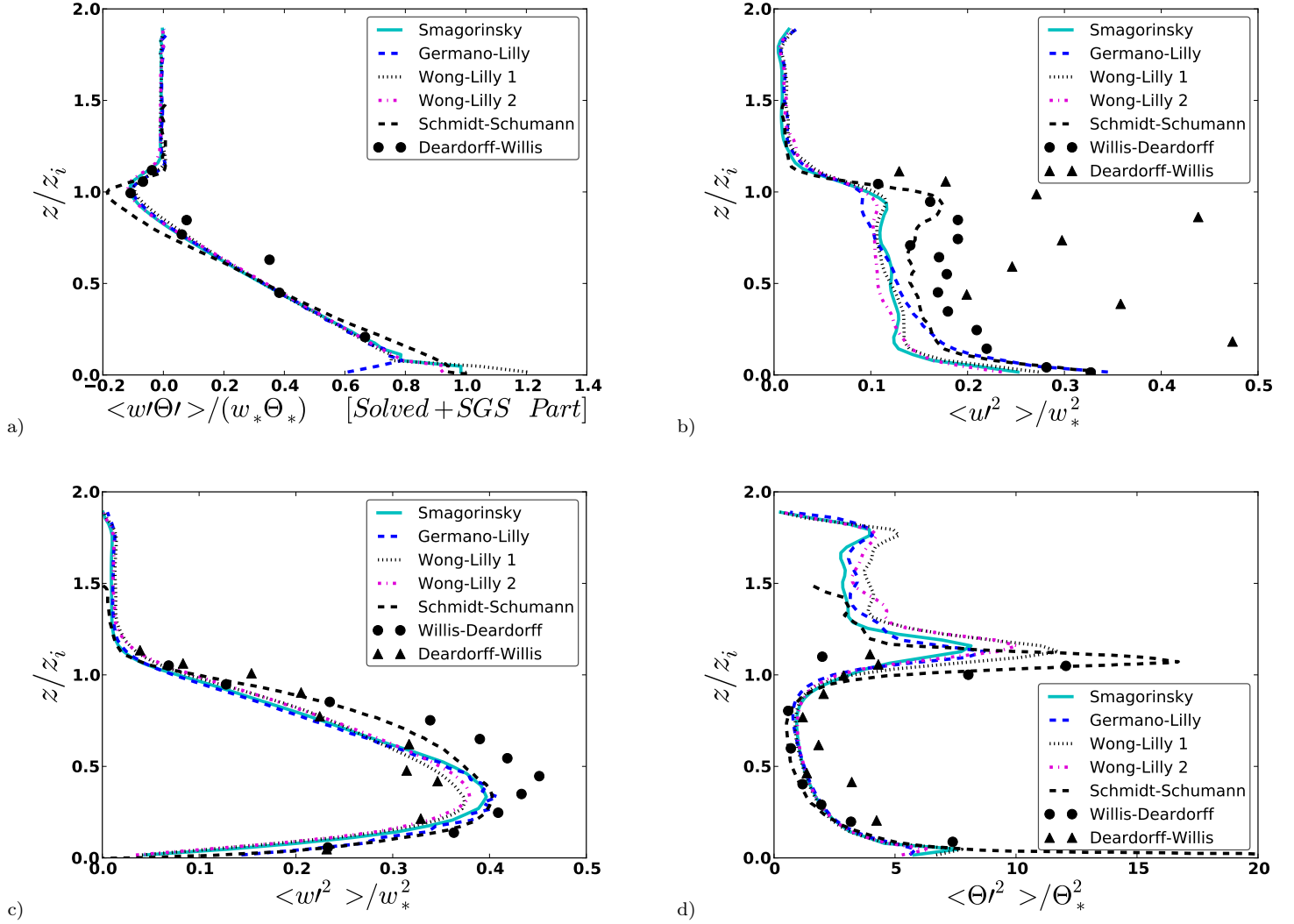
FIGURE 5.12 – Flux thermiques et variances normalisées (a) \langle w'\Theta' \rangle / (w_* \Theta_*) , (b) \langle u'^2 \rangle / w_*^2 , (c) \langle w'^2 \rangle / w_*^2 et (d) \langle \Theta'^2 \rangle / \Theta_*^2 en fonction de z/z_i . Les correspondances des lignes et des symboles sont similaires à la figure 5.10, excepté les pointillés-tiretés roses qui représentent le modèle de Wong-Lilly sans calcul dynamique du nombre de Prandtl turbulent [Wong-Lilly 2].
