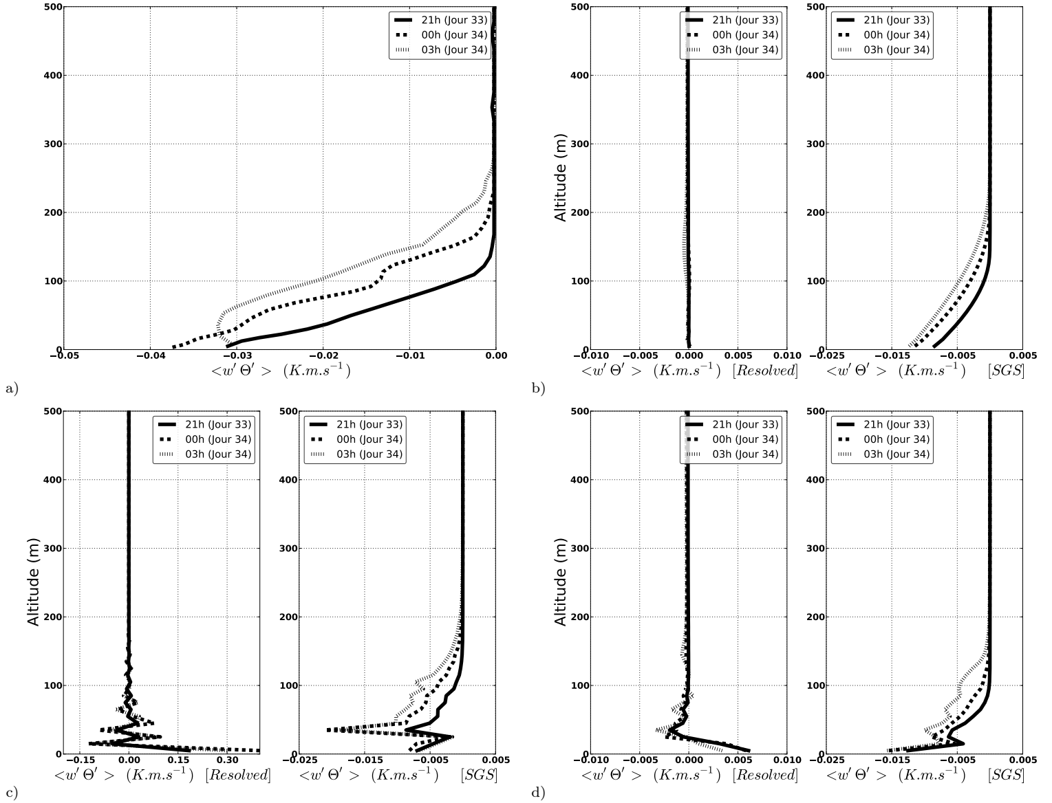
FIGURE 6.11 – Profils des flux thermiques verticaux \langle \overline{w'\Theta'} \rangle en fonction de l'altitude, la nuit, à 21h le jour 33, 00h et 03h le jour 34. (a) Le flux thermique total pour le modèle LASDD de [Basu et al., 2008]. Les résultats des flux thermiques résolus [Resolved] et sous-maille [SGS] pour les modèles de (b) Smagorinsky, (c) Germano-Lilly et (d) Wong-Lilly.
