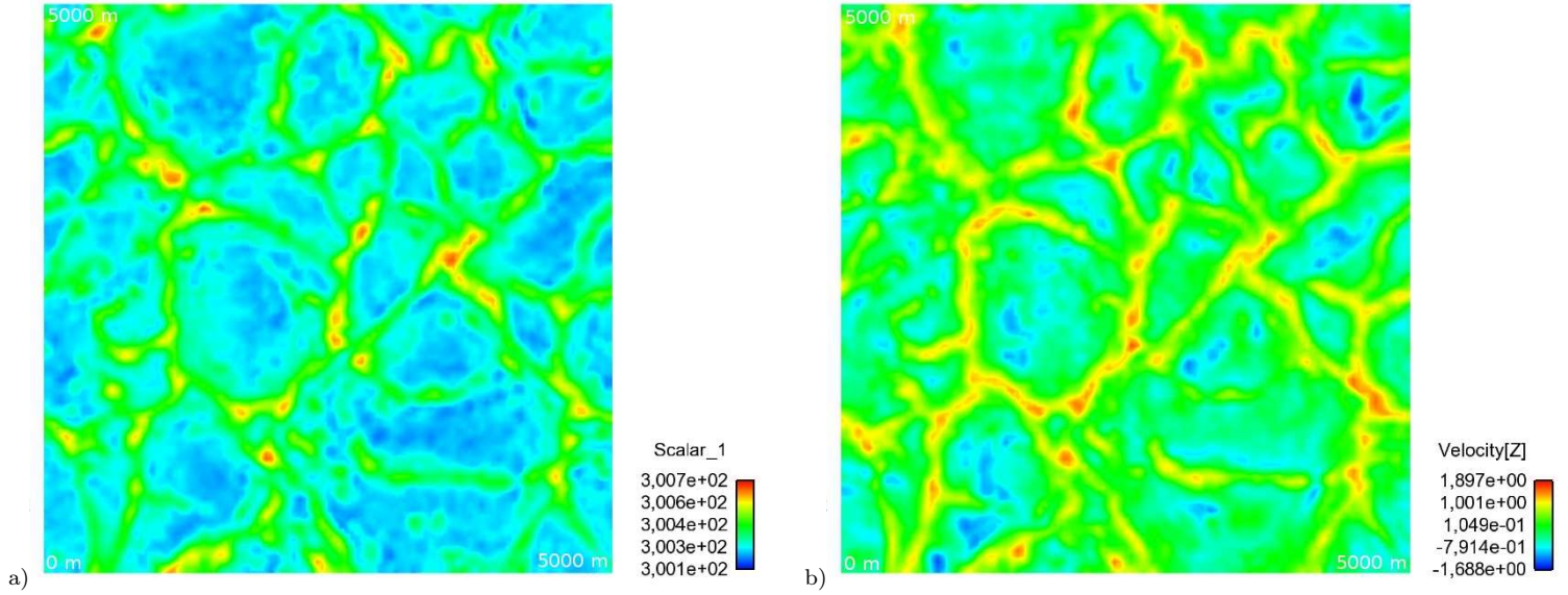
FIGURE 5.13 – Coupe du domaine à z = 100 m des champs 3D résolus de (a) température potentielle \bar{\Theta} (Scalar_1) et (b) vitesse verticale \bar{w} (Velocity[z]).
