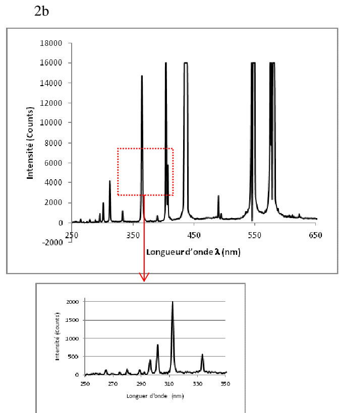
Figure II-2 : a- Distribution spectrale de la lampe HPL-N et b- Spectre UV-Visible de la lampe HPL-N mesuré par un spectrophotomètre à fibre optique.
