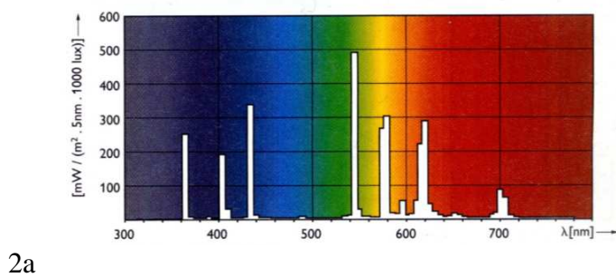
Figure II-2 : a- Distribution spectrale de la lampe HPL-N et b- Spectre UV-Visible de la lampe HPL-N mesuré par un spectrophotomètre à fibre optique.
