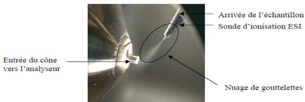
Figure II-4 Source d'électronébulisation (a) principe de fonctionnement (d'après Kebarle, 2000 [10] ) (b) photographie de la source ESI
