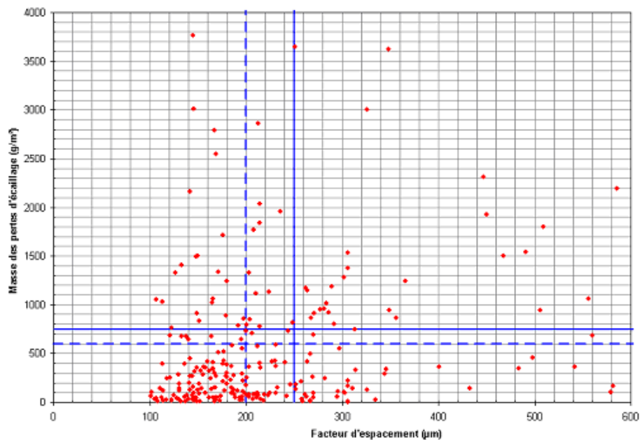
Figure 1.44 Relation entre le facteur d'espacement (seuils de 200 et 250 \mu\text{m} ) et l'écaillage (seuils de 600 et 750 \text{g}/\text{m}^2 ) d'après [Prost et Orcel, 2003], les seuils sont issus de [Recommandations gel, 2003]
