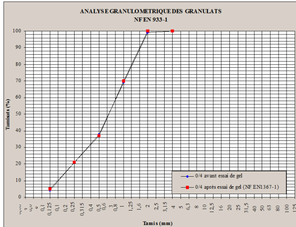
Figure 2.35 Évolution de la granulométrie du sable normalisé (CEN) après 10 cycles de gel-dégel dans l'eau
