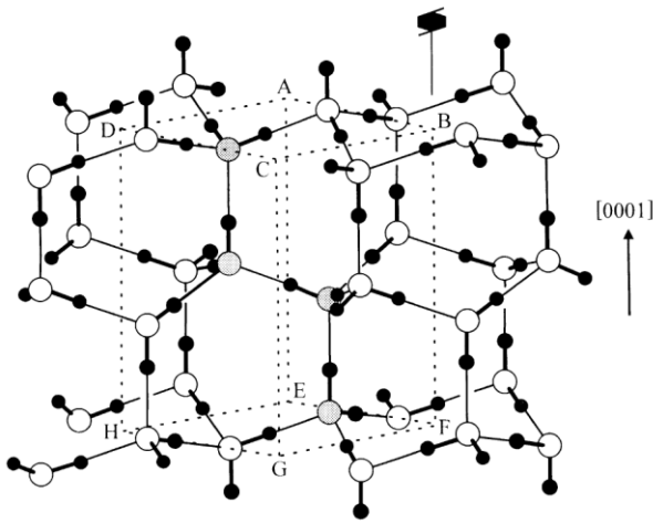
Figure 1.13 Structure cristalline hexagonale de la glace 1h d'après [Petrenko, 1999]
