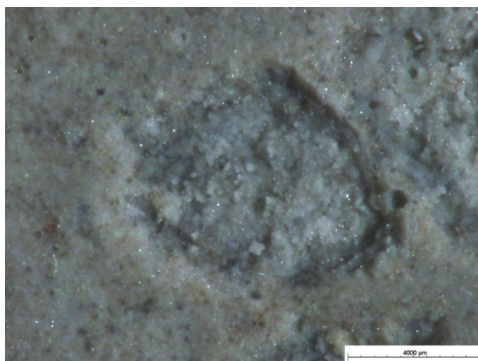
Figure 3.11 Dégradation localisée (diamètre d'un ordre de grandeur de 0,5 mm) à la surface d'un corps d'épreuve 16x14x3,5 (en cm) en mortier
