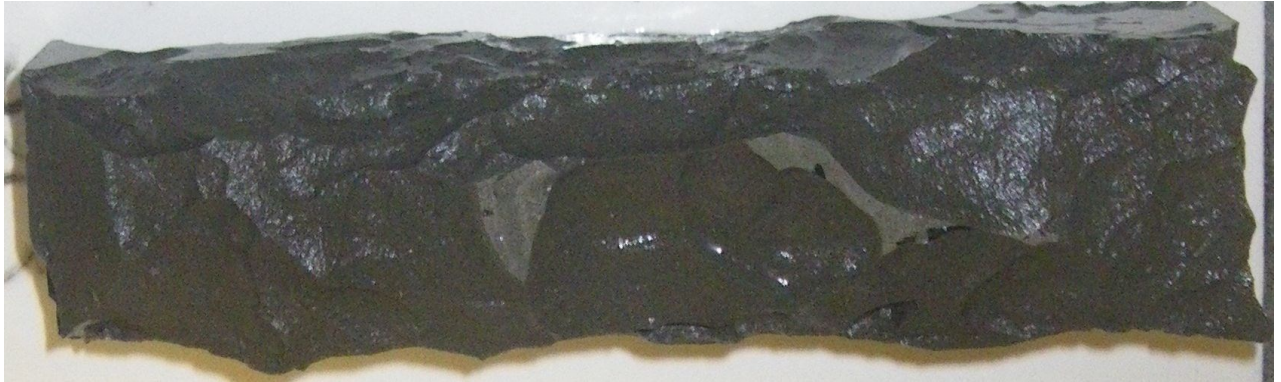
Figure 2.118 Coulis sans adjuvant ni ajout, C.p.1.(3)-0,44-0-0-0, partiellement immergé dans 3% de NaCl après 13 cycles de type écaillage (1 cycle/jour)
