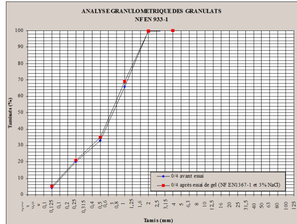
Figure 2.36 Évolution de la granulométrie du sable normalisé CEN après 10 cycles de gel-dégel dans une solution à 3% de NaCl
