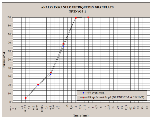
Figure 2.36 Évolution de la granulométrie du sable normalisé CEN après 10 cycles de gel-dégel dans une solution à 3% de NaCl
