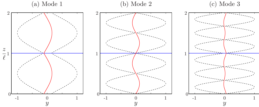
FIGURE 2.9 – Partie réelle (rouge) et enveloppe (pointillés noirs) des modes linéaires les plus instables pour \xi = 3.65 , et trois longueurs réduites différentes : (a) \ell = 0.55 , (b) \ell = 1 et (c) \ell = 1.50 . Sur chacune des figures, la ligne horizontale bleue indique la localisation d'un récupérateur d'énergie.
