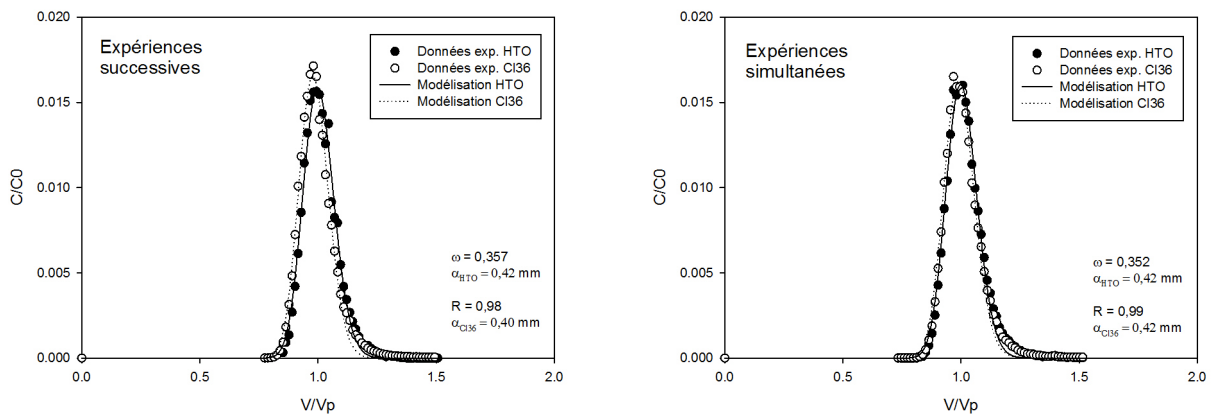
FIGURE C.11 – Comparaison entre les traçages successifs et simultanés de HTO et ^{36}\text{Cl} dans une colonne de sédiment désargilé reconstitué avec du sable humide.
