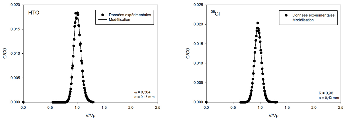
FIGURE C.2 – Percée de HTO et 36 Cl dans une colonne de sédiment complet reconstitué à sec.
