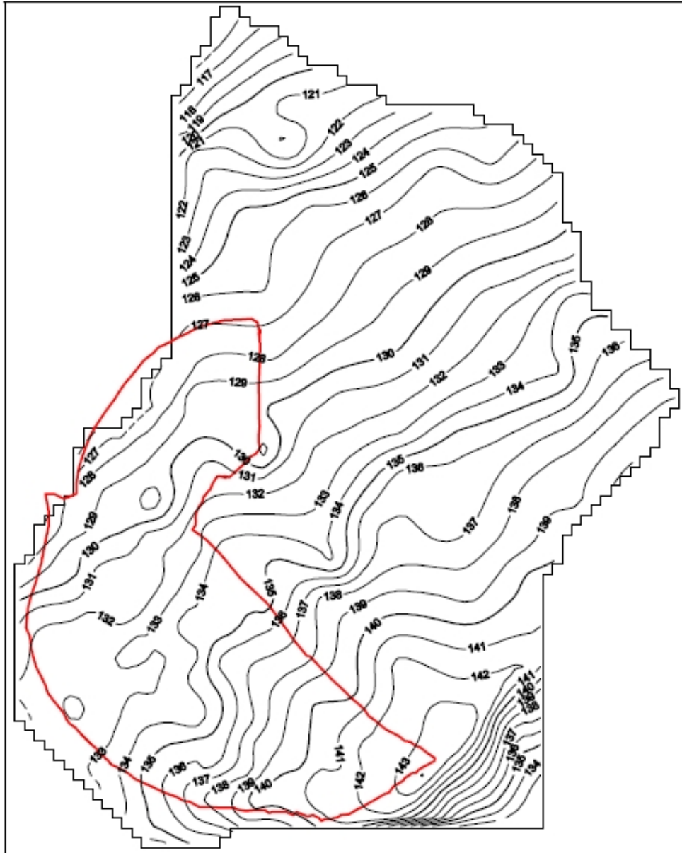
FIGURE 1.34 – Isohypses du substratum du modèle 1997 (in Andra (2004), Volume II, Chapitre 1).
