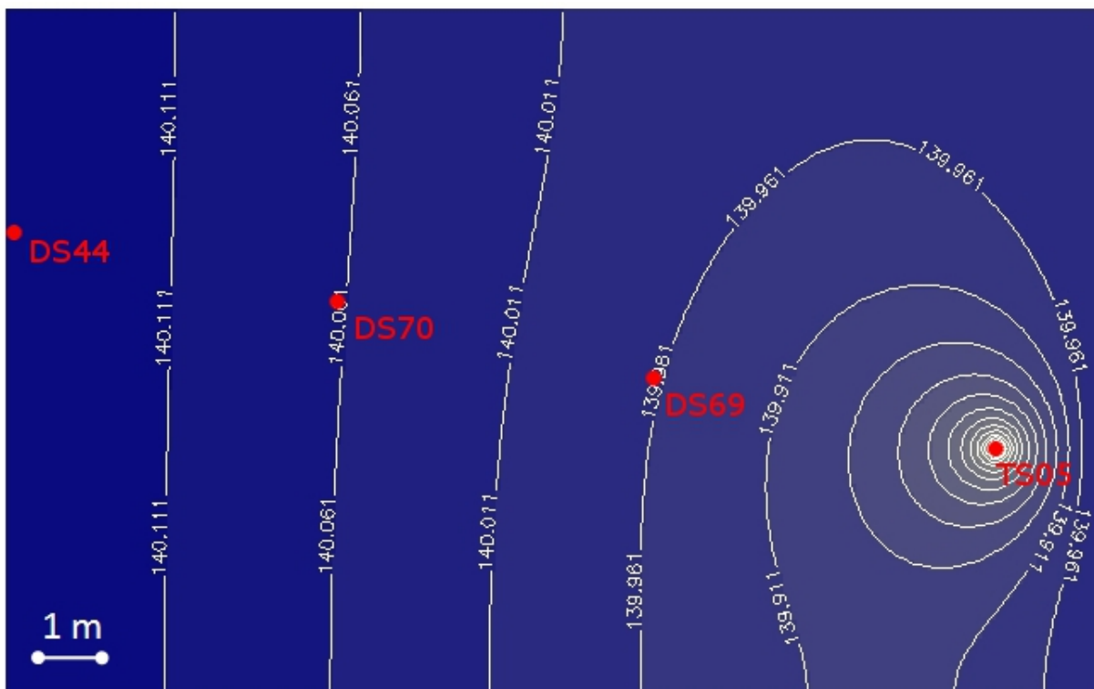
FIGURE 5.4 – Carte piézométrique du modèle.
