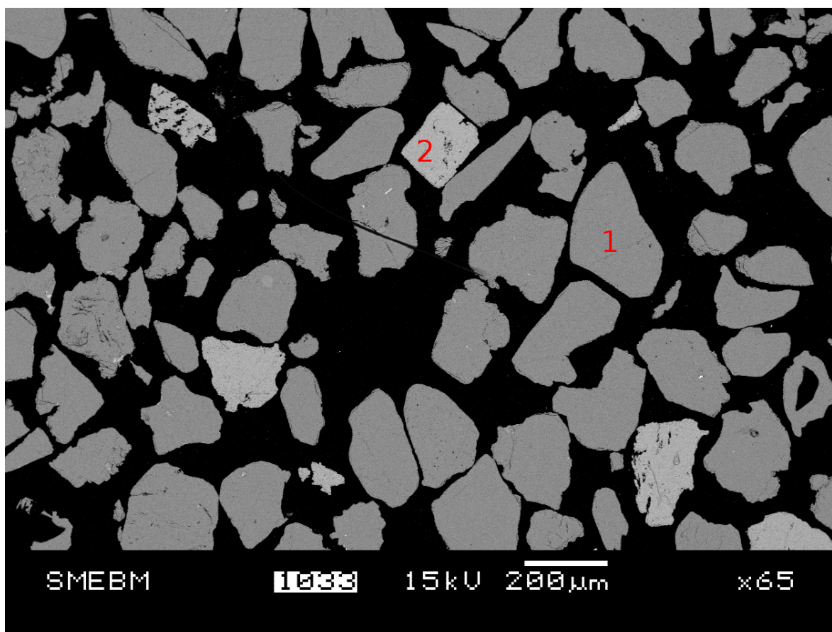
FIGURE 2.17 – Cliché MEB de la fraction majoritaire du sédiment aptien.
