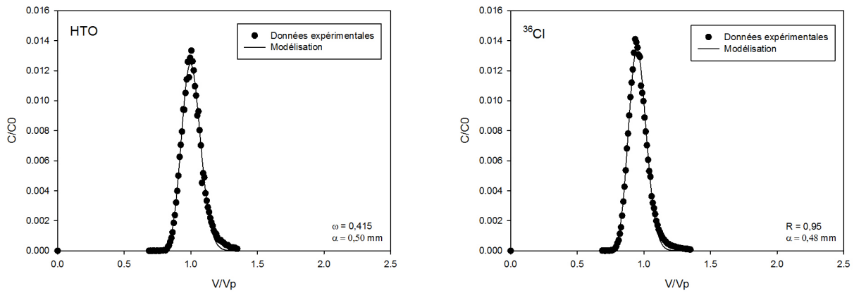
FIGURE C.1 – Percée de HTO et 36 Cl dans une colonne de sédiment désargilé reconstitué à sec.
