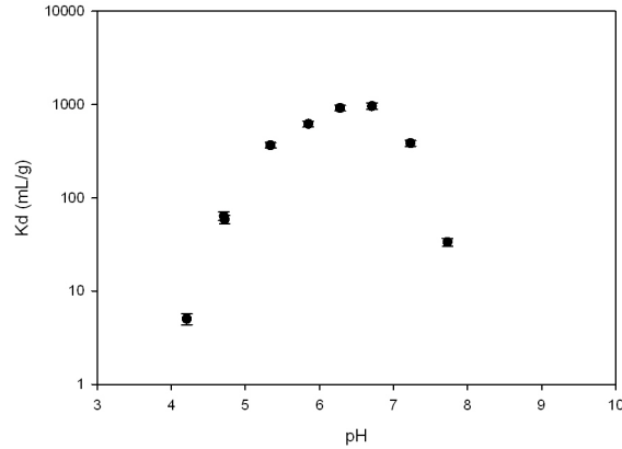
FIGURE 4.11 – Etude du K_d(\text{U(VI)}\text{-Sédiment désargilé}) en fonction du pH à [U] = 2.10^{-7} \text{ mol/L} , pCO_2 = p_{atm} , [NaCl] = 6,4.10^{-3} \text{ mol/L} , S/L = 10 \text{ g/L} .
