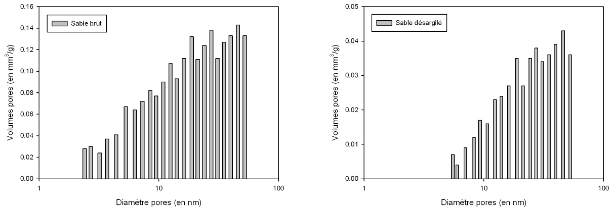
FIGURE 3.21 – Distribution de la taille des pores pour des échantillons de sable brut et désargilé.
