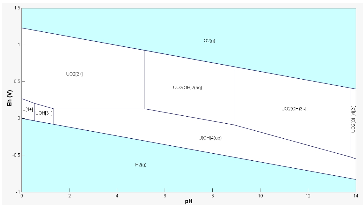
FIGURE 4.2 – Diagramme de Pourbaix de l'Uranium à 10^{-9} mol/L.
