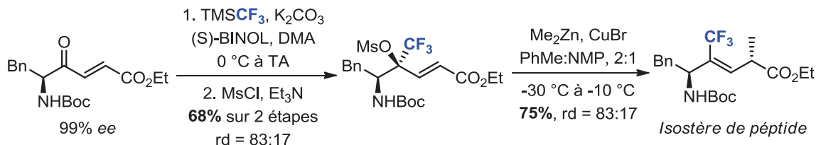
Schéma VI-3 – Application de la trifluorométhylation de cétones à la synthèse de vinyles- \text{CF}_3
