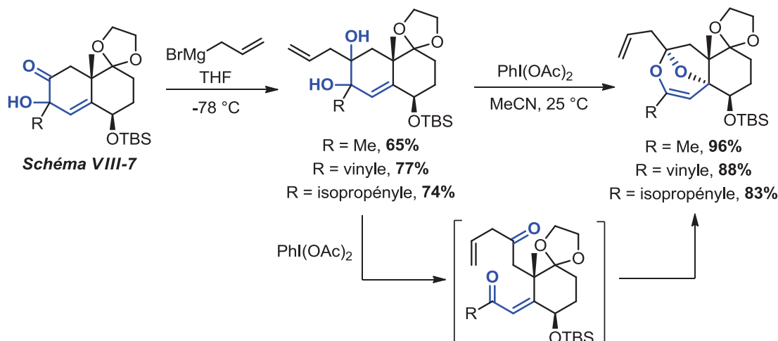
Schéma VIII-20 – Addition d'un organométallique sur la cétone d' \alpha -céto carbinol vinyliques et exploitation des diols-1,2 obtenus
