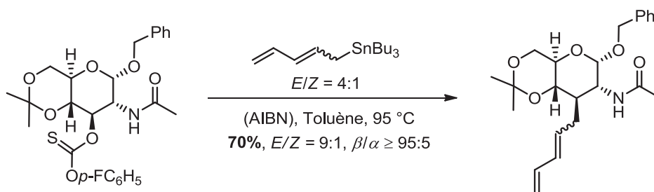
Schéma III-10 – Installation d'une chaîne pentadiényle sur un dérivé de sucre
