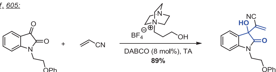
Schéma VIII-5 – Exemples de réactions de Baylis-Hillman
