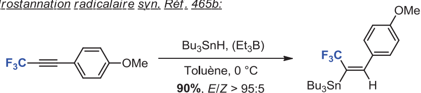
Schéma VI-6 – Hydro-métallation d'alcynes trifluorométhylés
