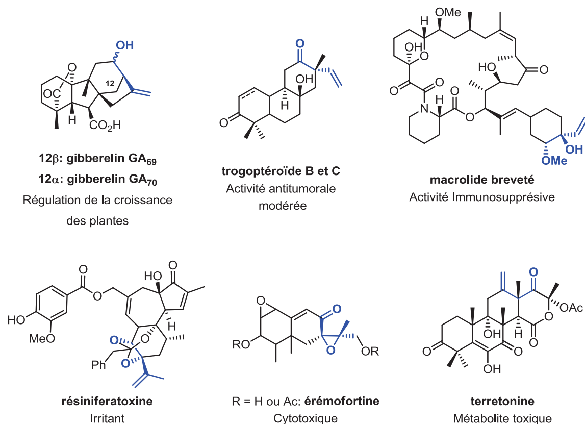
Schéma VIII-3 – Exemples de produits naturels contenant un motif qui pourrait être installé via un \alpha -céto carbinol vinylique a
