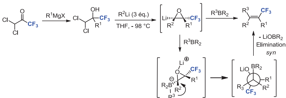
Schéma VI-4 – Synthèse de vinyles- \text{CF}_3 tétrasubstitués de géométrie contrôlée
