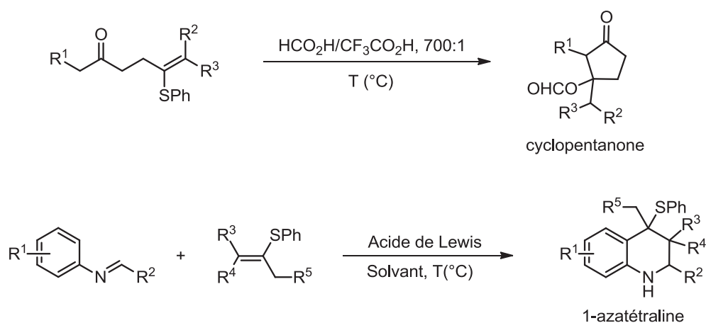
Schéma V-33 – Valorisations potentielles des sulfures vinyliques
