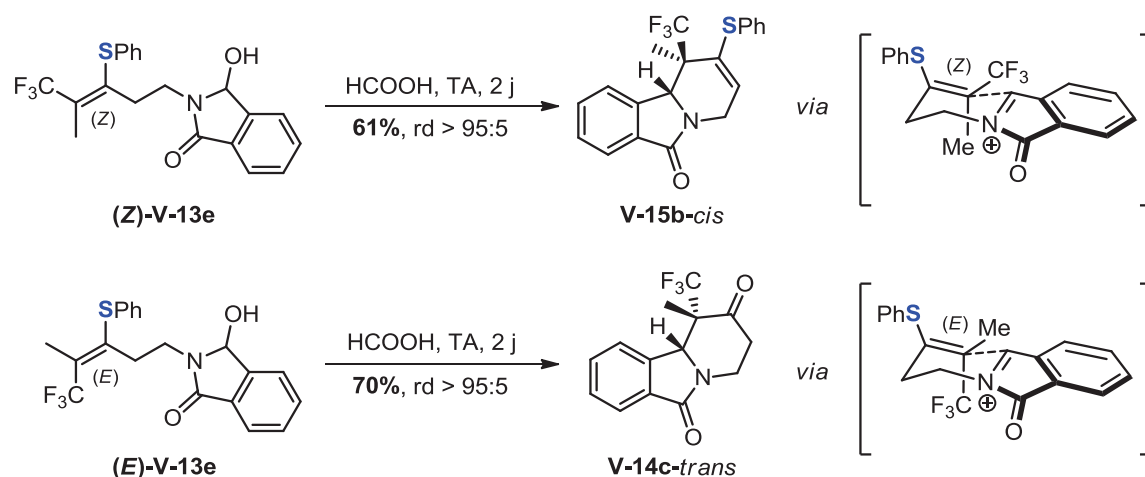
Schéma V-32 – Stéréospécificité de la réaction de cyclisation
