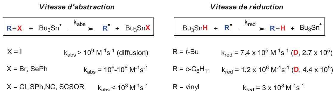
Schéma I-13 – Constantes d'abstraction par le radical Bu_3Sn^\bullet et de réduction par l'hydruure Bu_3SnH
