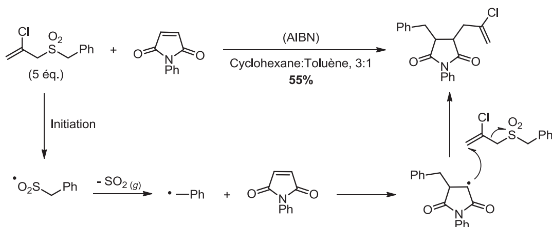
Schéma III-21 – Piègage du radical intermédiaire par le N-phénylmaléimide
