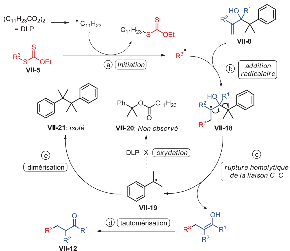
Schéma VII-29 – Mécanisme de la réaction d'addition-élimination
