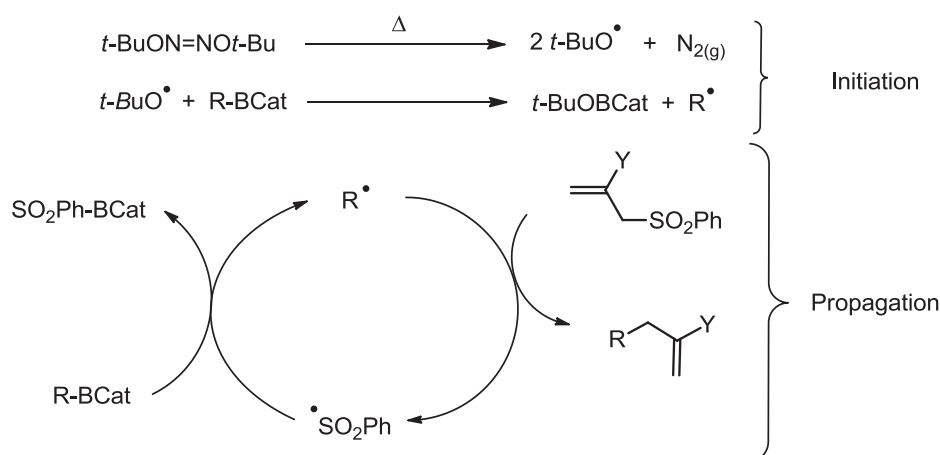
Schéma III-27 – Exemples et mécanisme de la méthode au catécholborane de Renaud
