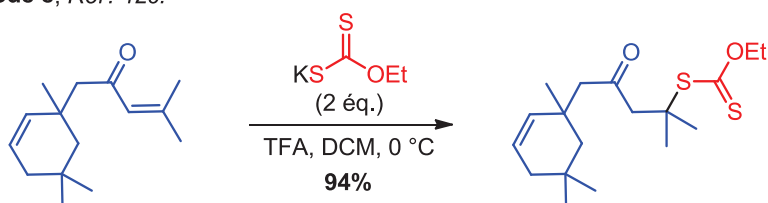
Schéma II-15 – Quelques exemples de préparation de xanthates
