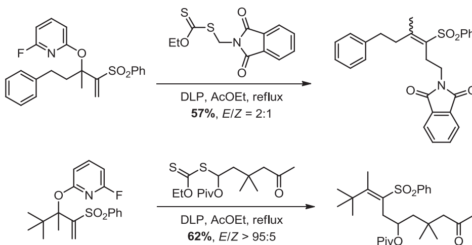
Schéma III-48 – Synthèse de vinyliques tétra-substitués
