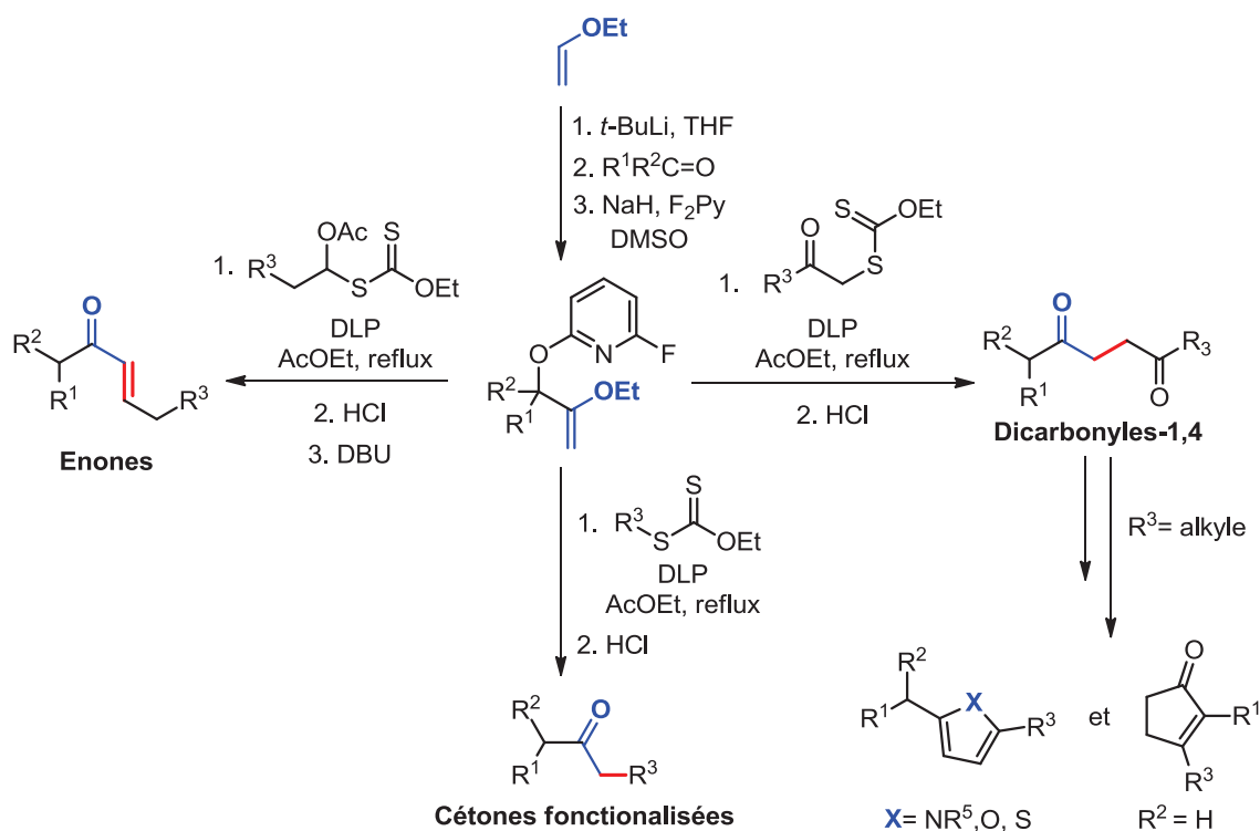
Schéma IV-15 – Bilan de la méthode : synthèse de cétones, de dicétones-1,4 et d'étones; accès à des carbo-/hétéro-cycles à 5 chaînons
