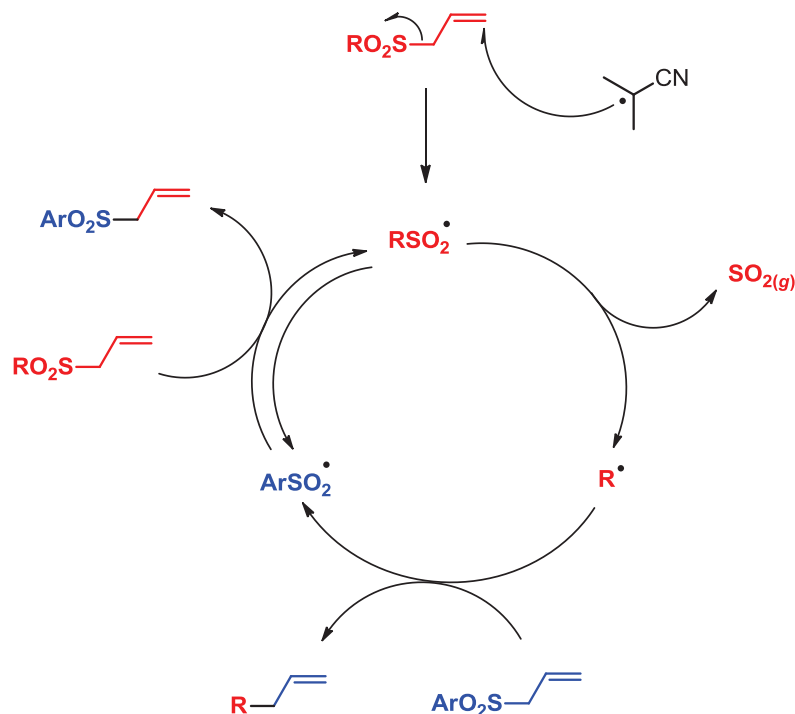
Schéma III-20 – Mécanisme de l'allylation par extrusion de dioxyde de soufre
