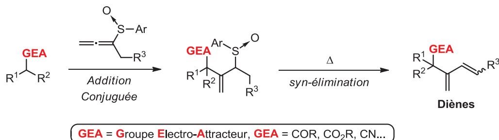
Schéma VIII-36 – Applications potentielles de l'addition conjuguée sur des alcynyles et des allényles sulfoxydes
