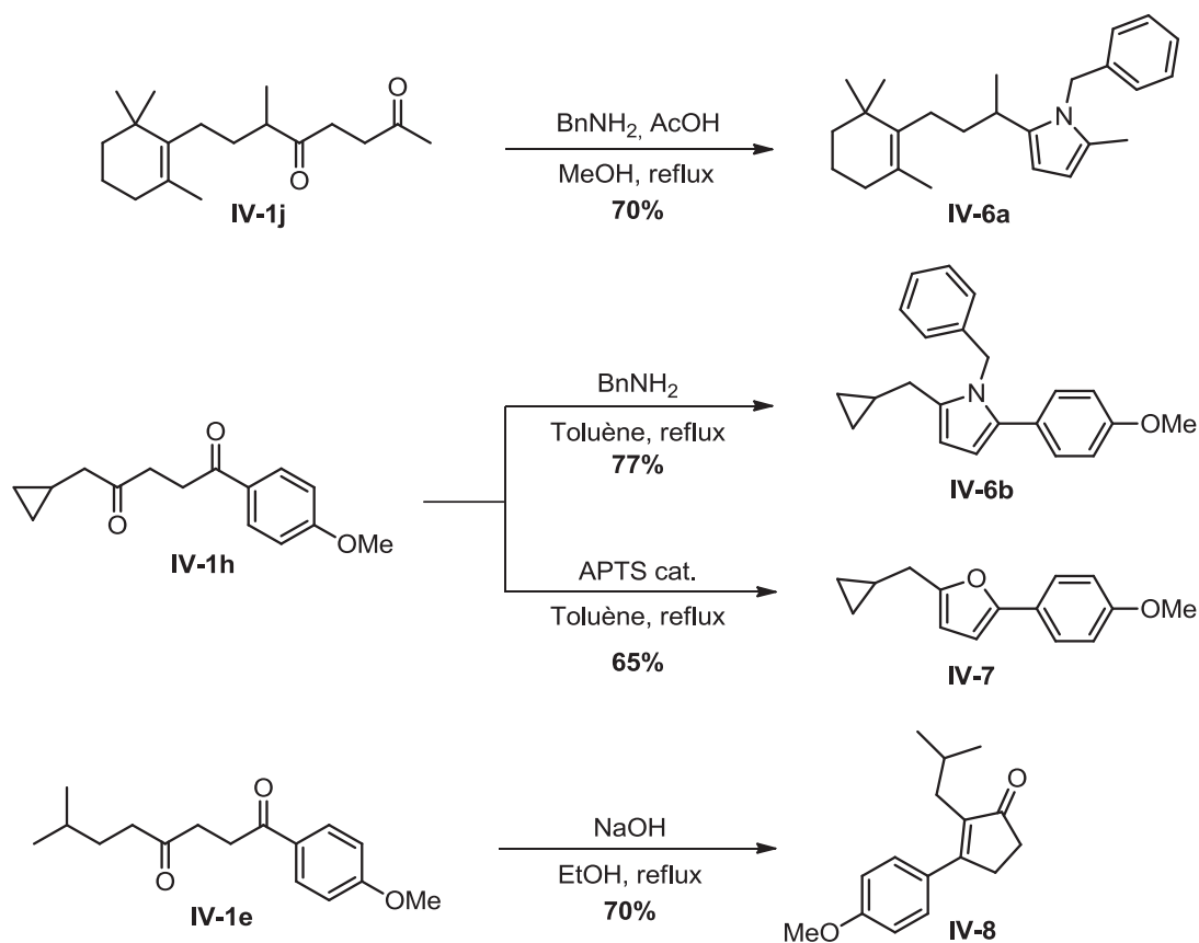
Schéma IV-11 – Préparation de cycles à 5-chaînons
