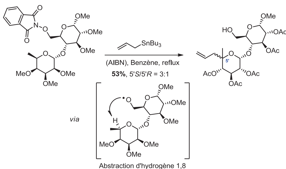
Schéma III-8 – Allylation d'un carbohydrate par cascade radicalaire
