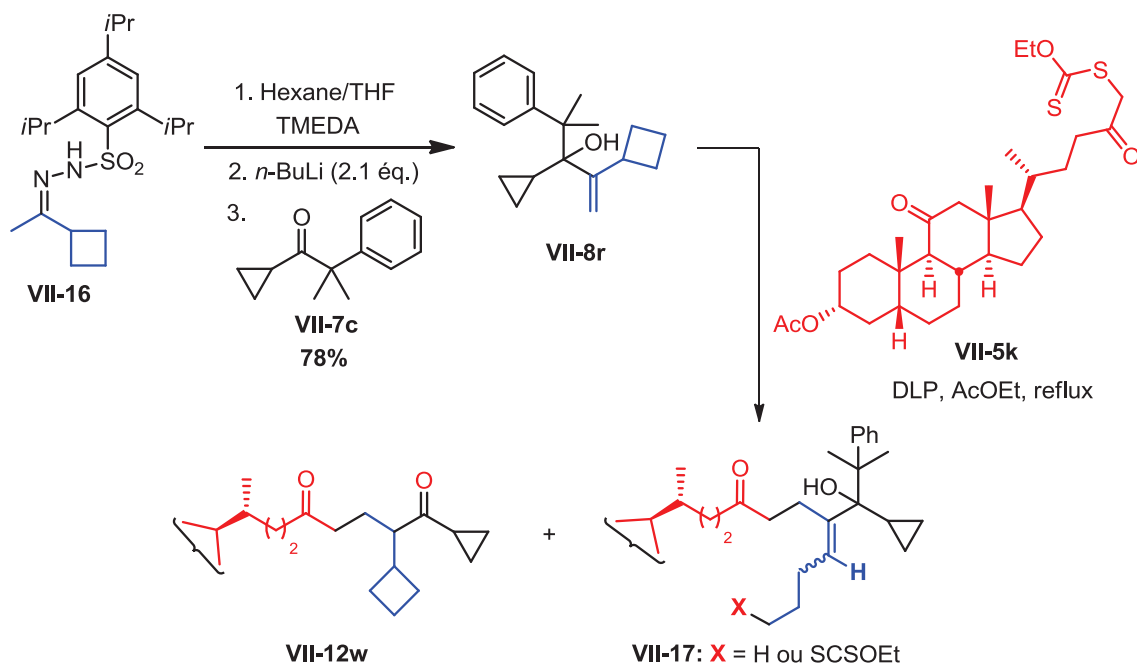
Sch\u00e9ma VII-28 – Comp\u00e9tition entre l'\u00e9limination et l'ouverture du cyclobutane
