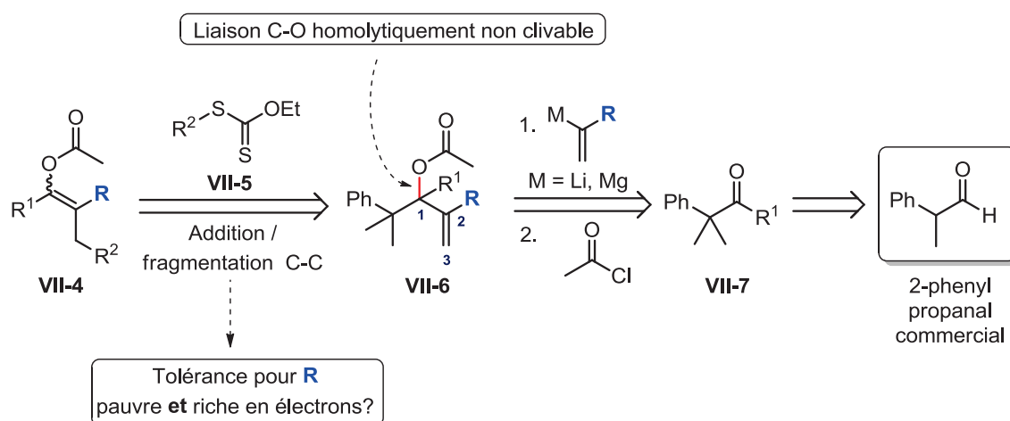
Schéma VII-10 – Stratégie d'obtention d'esters d'énol
