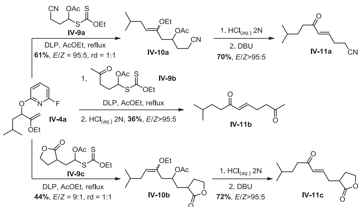
Schéma IV-14 – Synthèse d'ènones de géométrie ( E )
