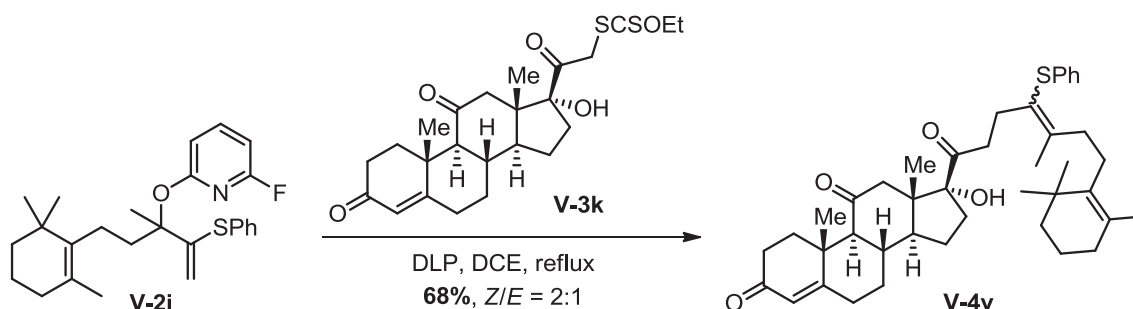
Schéma V-15 – Synthèse d'un sulfure vinylique tétra-substitué complexe
