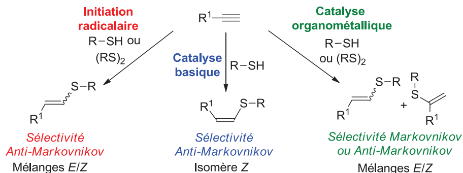
Schéma V-4 – Bilan de la méthode d'hydrothiolation
