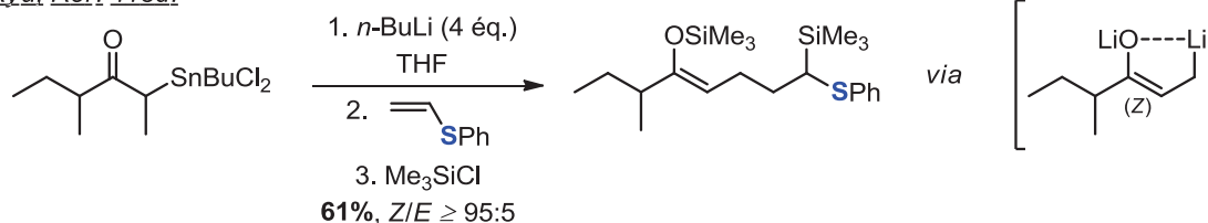
Schéma V-24 – Exemples de carbométallation de sulfures vinyliques
