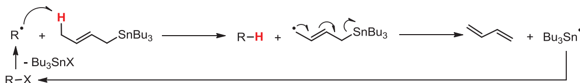
Schéma III-14 – Arrachement d'hydrogène sur le crotyltributylétain
