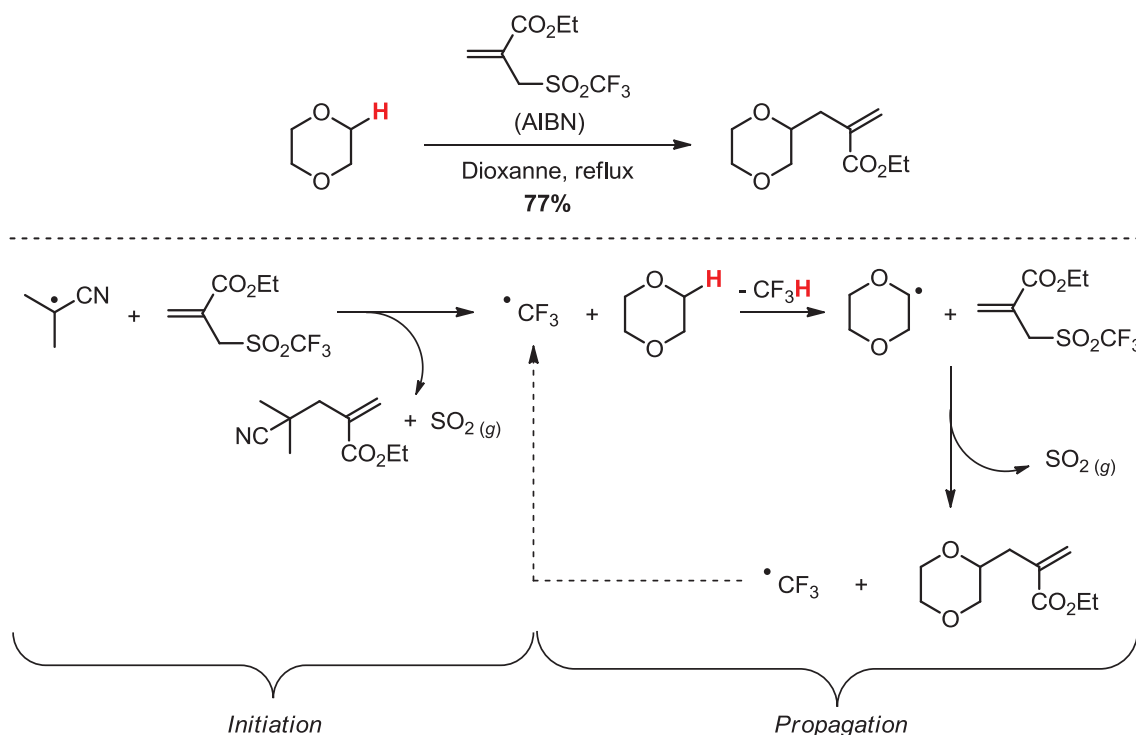
Schéma III-26 – Allylation utilisant les trifluorures de Fuchs
