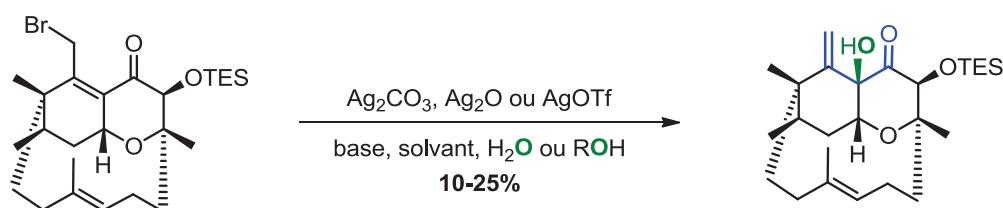
Schéma VIII-15 – Déplacement d'un bromure allylique
