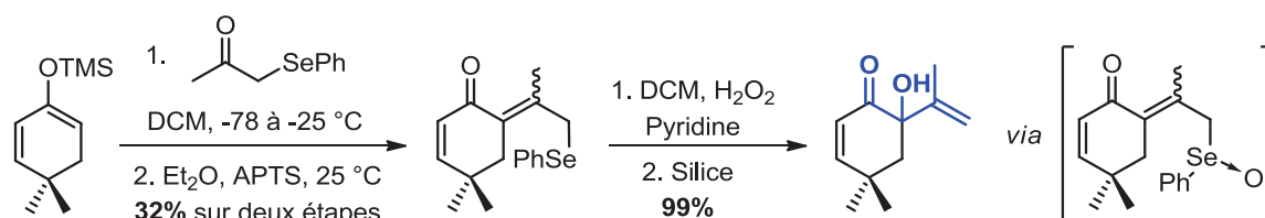
Schéma VIII-18 – Réarrangement sigmatropique d'un sélénoxyde allylique
