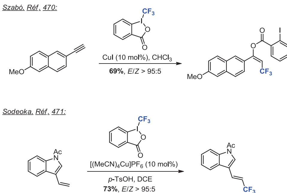
Schéma VI-8 – Oxy-trifluorométhylation d'alcyne et d'alcène
