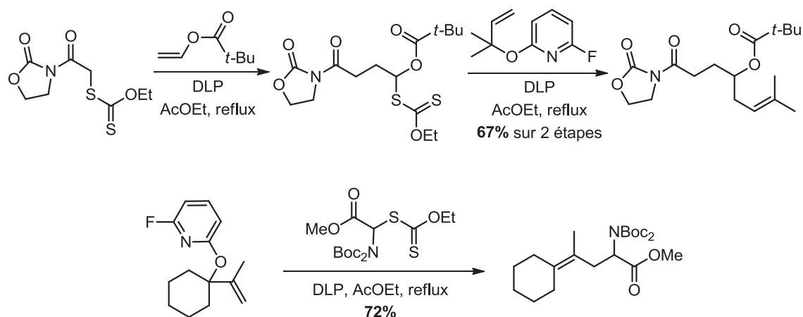
Schéma III-44 – Exemples d'allylations radicalaires
