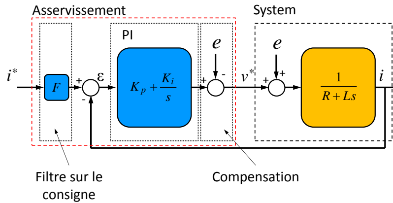
Figure 129 Diagramme de l'asservissement de courant
