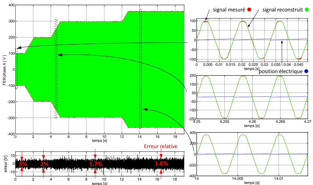
Figure 115 Relevés de fem à vide, mesurée et reconstruite
