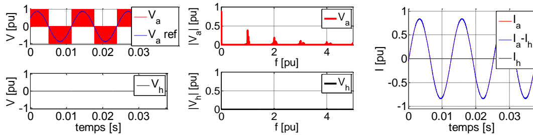
Figure 27 Modulation vectorielle « Z SVM » utilisant un modèle d'onduleur avec commutation idéale
