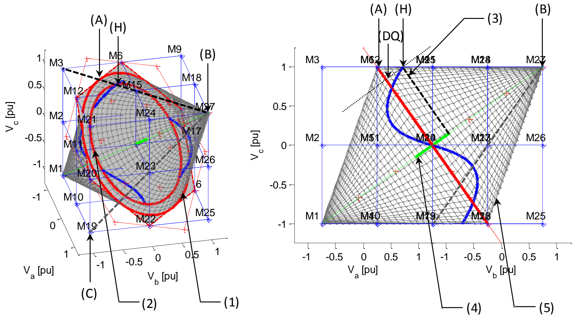
Figure 149 Zoom sur l'espace accessible de la machine fictive principale en fonction de la composante homopolaire de tension
