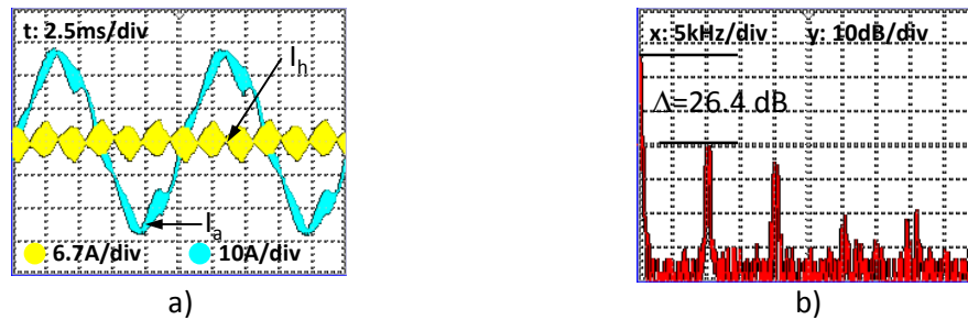
Figure 99 a) Courant de phase et courant homopolaire pour la stratégie « 3 Niveaux Simple Modulation » ; b) Analyse spectrale du courant de phase avec atténuation de 26.4 dB à 10 kHz par rapport au fondamental
