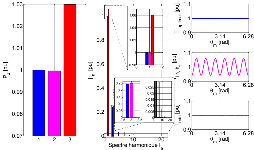
Figure 47 Pertes Joule, analyse spectrale du courant de phase et couple obtenu pour k_{FEM3}/k_{FEM1}=0.25 et pour trois stratégies de commande : pertes Joule optimales à couple constant (courbes bleues) ; pertes Joule minimales en autorisant uniquement les harmoniques un et trois de courant (courbes magenta) et la stratégie à courant sinusoïdal (courbes rouges)
