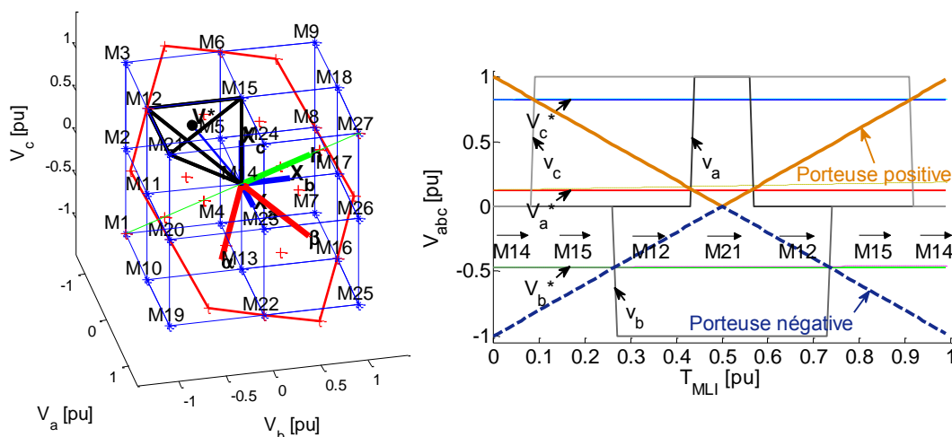
Figure 16 Modulation de type « 3 Niveaux Simple Modulation » – vecteurs activés pendant une période MLI (voir zoom en annexe 6.10)
