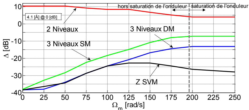
Figure 103 Atténuation du courant homopolaire à la fréquence MLI par rapport au fondamental égal à 4.1 [A] (0.2 pu en régime nominal)
