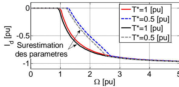
Figure 70 Effet sur le courant I_d par la prise en compte des phénomènes dynamiques
