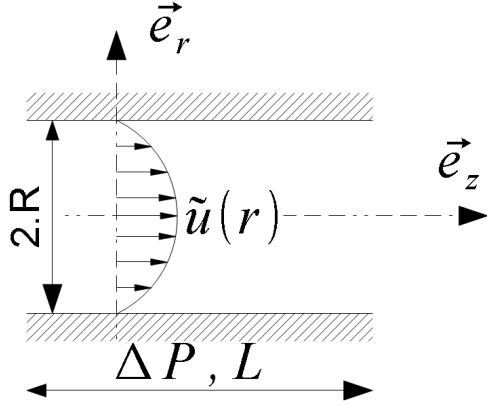
FIGURE 3.1 – Représentation géométrique de l'écoulement et du système de coordonnées cylindriques
