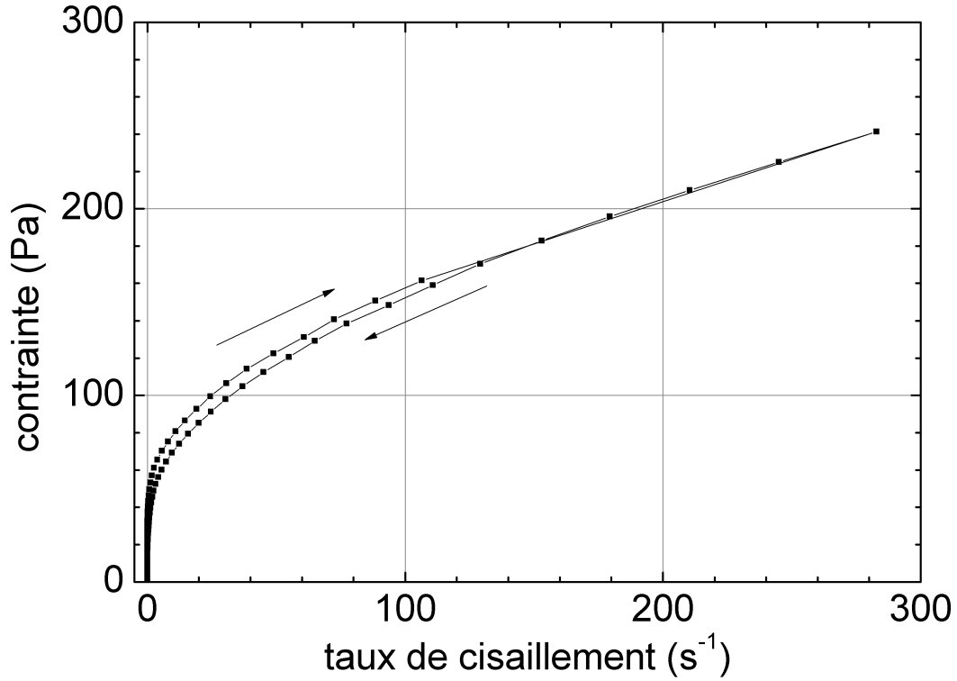
FIGURE 2.20 – Rhéogramme de l'émulsion avec mesure de thixotropie
