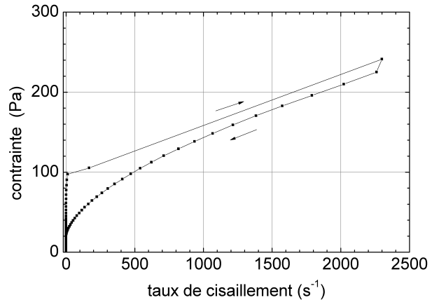
FIGURE 2.14 – Boucle thixotrope pour une solution de bentonite à 9% en masse à 25°C
