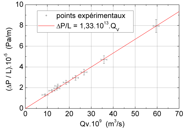
(b) Injection dans deux capillaires en parallèle, de diamètres 289 et 680\mu m
