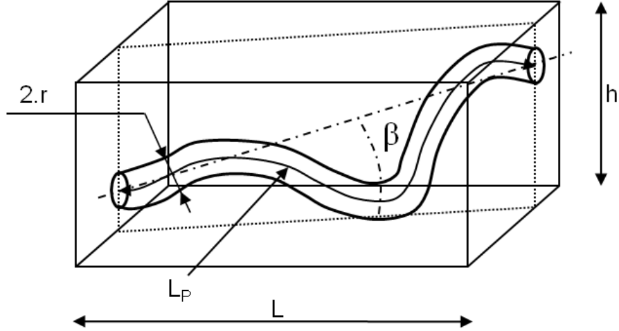
FIGURE 1.4 – Définition des paramètres géométriques de la tortuosité et de l'orientation d'un pore.
