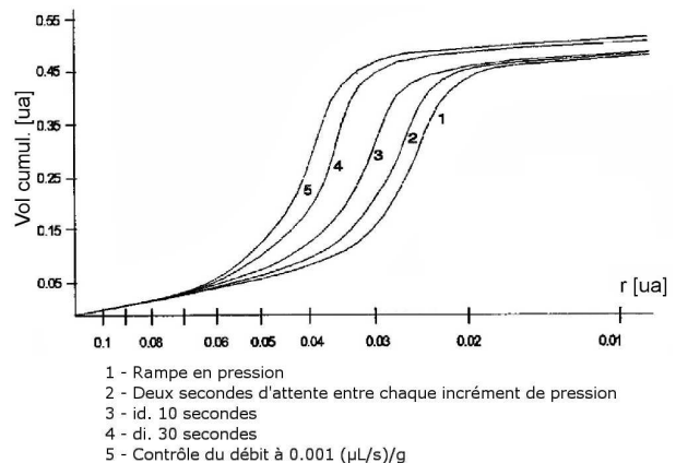
FIGURE 1.13 – Influence du protocole d'injection sur la taille des pores et le volume poreux cumulé [32]
