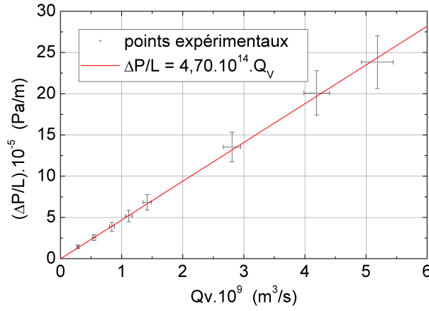
(a) Injection dans un seul capillaire de diamètre 289\mu m
