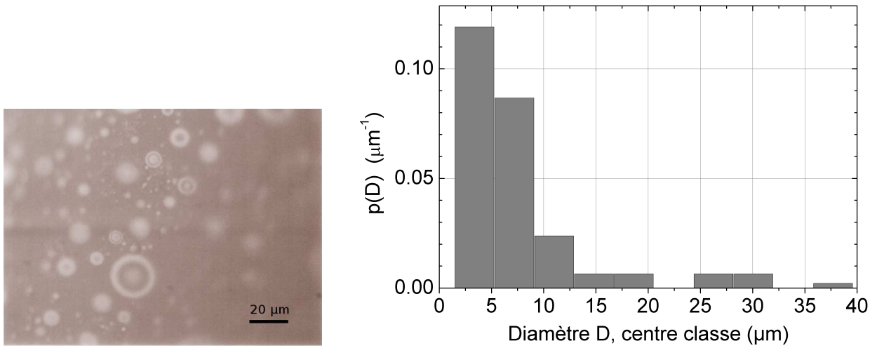
(a) Portion de la micrographie des micelles (b) Représentation en histogramme de la distribution de taille des micelles
