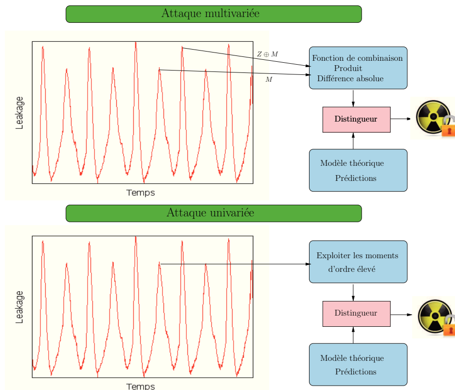
Figure 2: Illustration des attaques d'ordre élevé.
