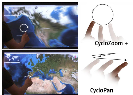
FIGURE 2.26: CycloZoom et CycloStar : deux techniques permettant respectivement de zoomer et panner sur une surface tactile.
