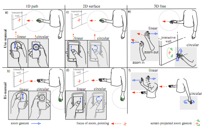
FIGURE 2.27: Représentation des différents gestes proposés par Nancel pour interagir sur très grand écran, (incluant des gestes basés sur des mouvements oscillatoires).
