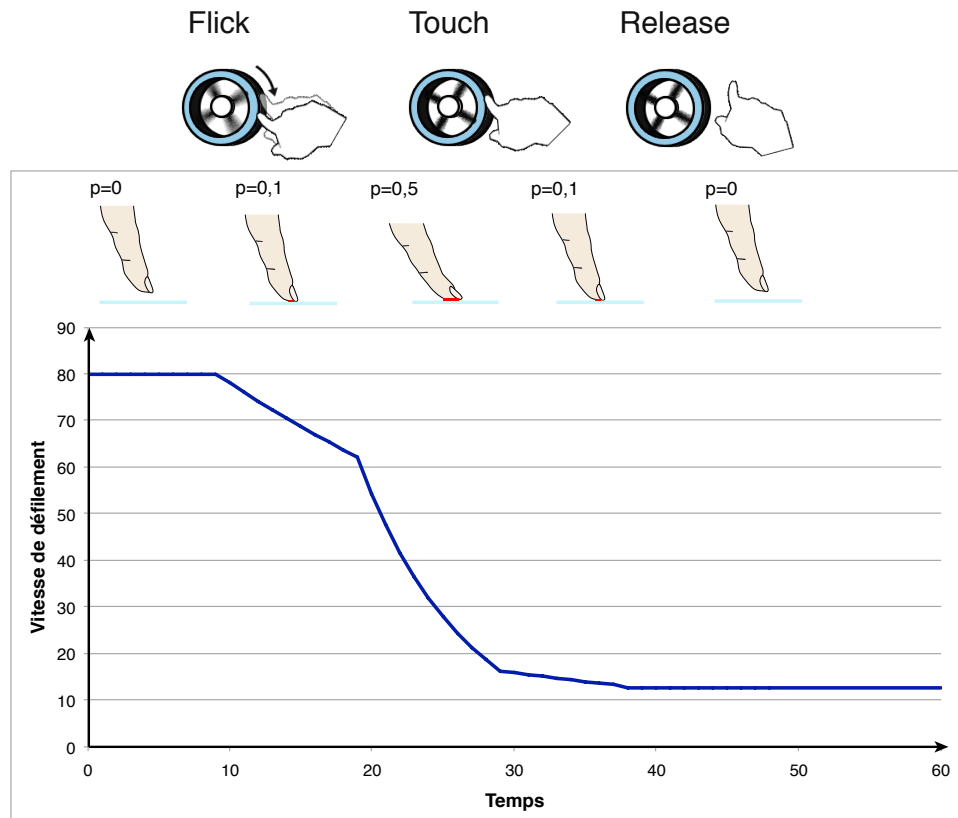
FIGURE 3.11: Comportement de la technique Flick-and-Brake avec la métaphore du mouvement inertiel.
