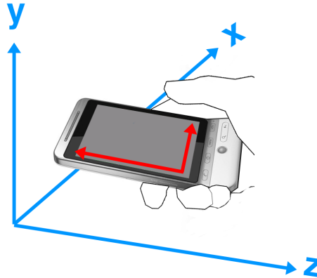
FIGURE 1.2: En bleu le référentiel terrestre et en rouge le référentiel du mobile
