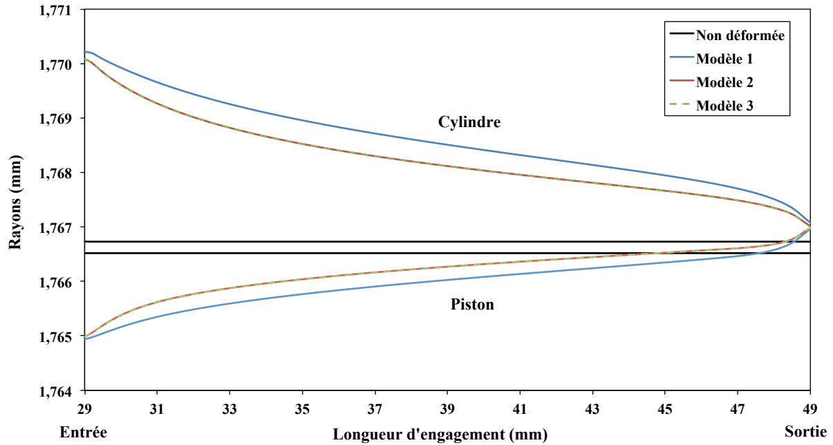
FIGURE 3.39: Jeu dans l'ensemble piston-cylindre 1 GPa N°2, en libre déformation, pour une pression maximale 1 GPa, pour les trois modèles de calcul.
