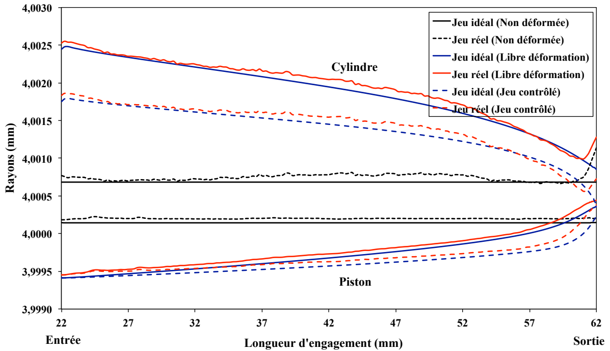
FIGURE 4.18: Déformation obtenu pour le jeu idéal et le jeu réel, pour une pression 200 MPa, sur l'ensemble piston-cylindre 200 MPa N o 4, en libre déformation et en jeu contrôlé.
