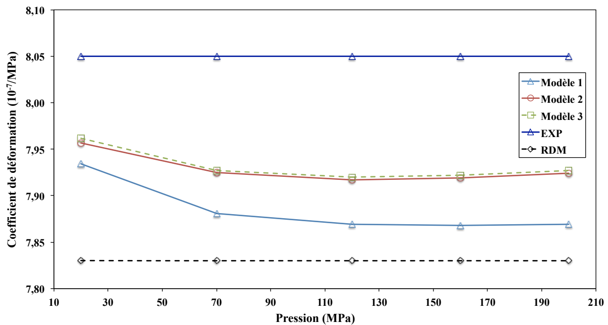
FIGURE 4.1: Comparaison des résultats du coefficient de déformation ( \lambda ) en fonction de la pression, entre l'expérimentation (EXP), les trois modèles et le calcul théorique de la résistance des matériaux (RDM), sur l'ensemble piston-cylindre 200 MPa N°4, en libre déformation.
