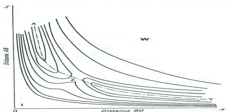
Figure 58 : La dynamique de « l'atome-foule » vue par la chimie quantique selon Bachelard 769 .
