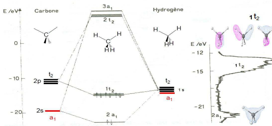
Figure 74 : Diagramme de corrélation du méthane et spectre photoélectronique 980 .
