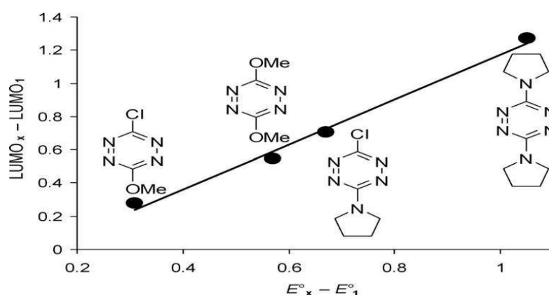
Figure 9 : Corrélation entre propriétés collectives. Les différences sont faites par rapport aux grandeurs associées à la dichloro-s-tétrazine prise pour référence ( LUMO_1 et E_1^0 ) 96 . L'indicateur de fiabilité de la linéarisation obtenue est élevé (voir publication d'origine).
