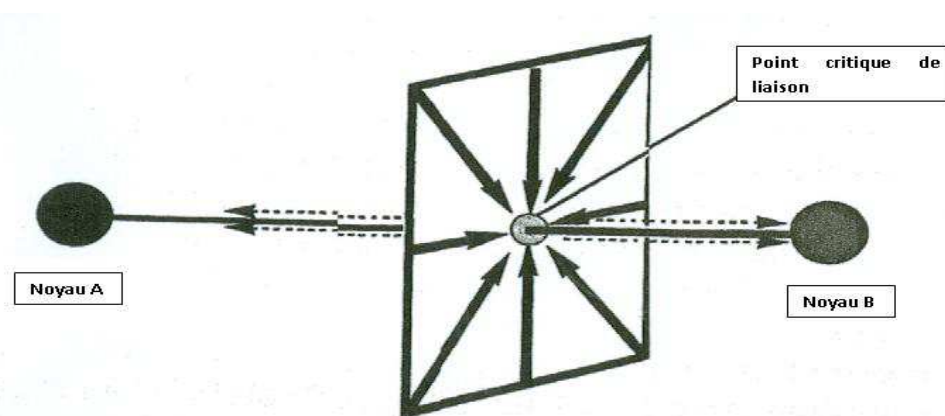
Figure 78 : Ligne d'interaction atomique entre les noyaux A et B 1024 .
