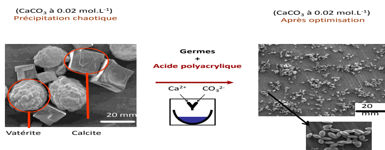
Figure 20 : Effet du procédé sur la précipitation 113 .
