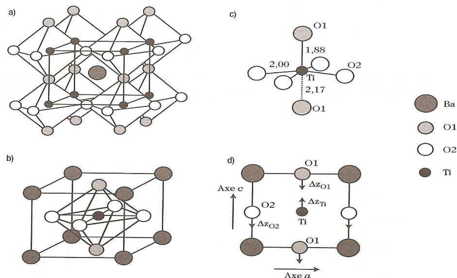
Figure 32 : Structure cristalline pérovskite non déformée, cubique, de \text{BaTiO}_3 au-dessus de la température de CURIE (cas (a) : origine centrée sur un ion \text{Ba}^{2+} ; cas (b) : origine centrée sur un ion \text{Ti}^{4+} ) et représentations schématiques de la déformation tétragonale de celle-ci au-dessous de la température de Curie (cas (c) et (d)) 165 .
