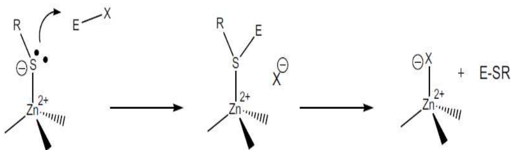
Figure 84 : Réaction d'alkylation du soufre du groupement thiolate relié au zinc 1047 .
