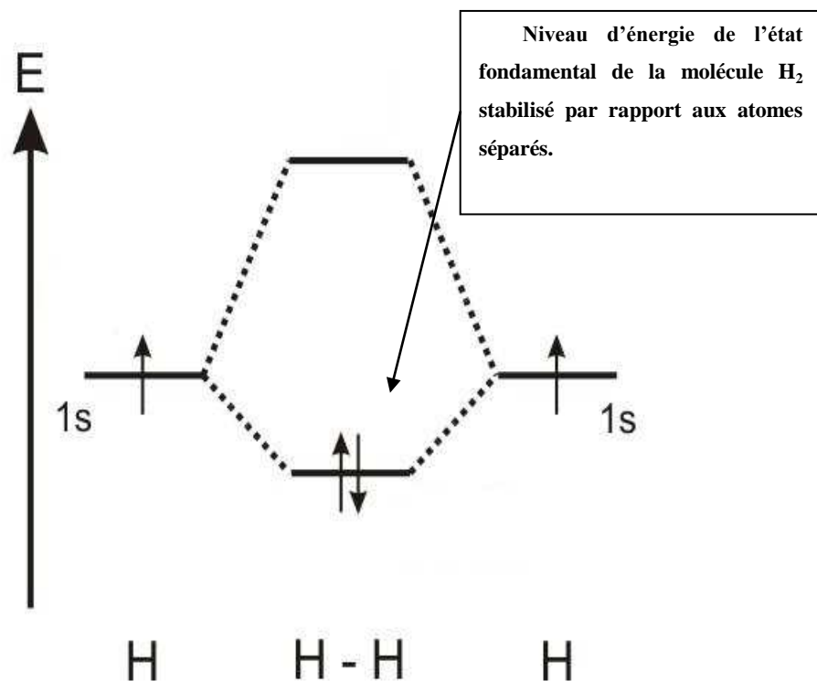
Figure 60 : Liaison chimique et énergie de l'entité dans le cas du dihydrogène.
