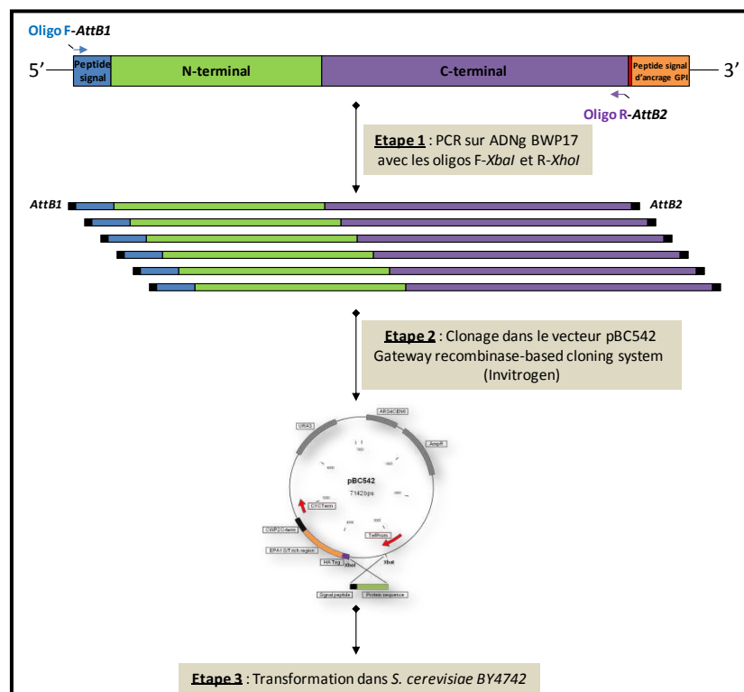
Figure 100 : Clonage des séquences codantes de Rbt1SL, Rbt1FL et Eap1 dans pBC542 en utilisant le système Gateway dans S. cerevisiae BY4742
