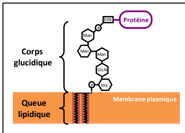
Figure 12 : Structure d'une ancre GPI sans groupements ramifiés EtN : éthanolamine. P : phosphate. Man : mannose. GlcN : glucosamine. Ins : inositol.
