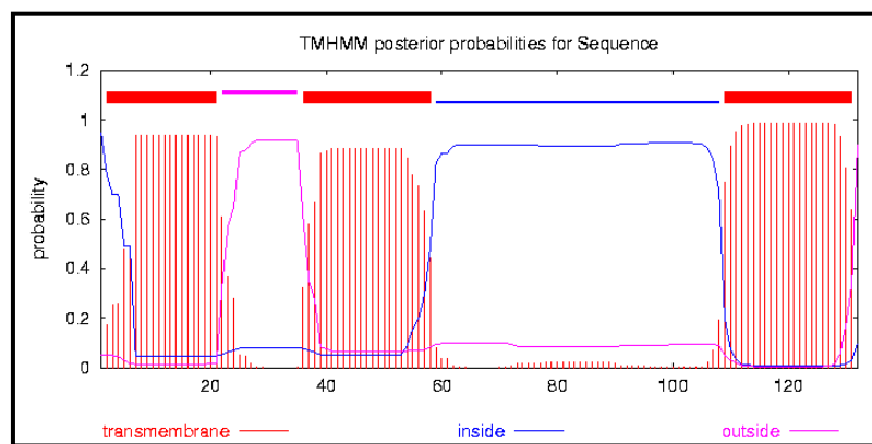
Figure 30 : Schéma de prédiction de domaines transmembranaires de la protéine Pga1
