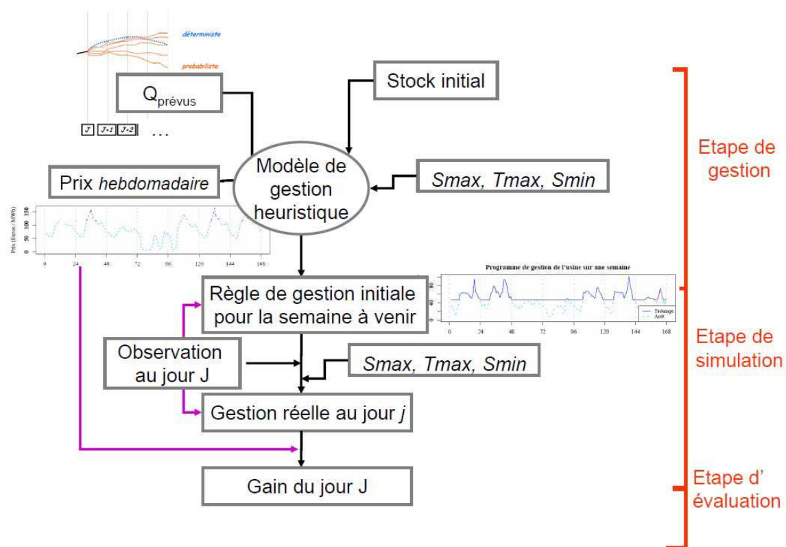
Figure 138: Schématisation de la procédure développée pour l'optimisation heuristique d'une réserve hydroélectrique pour un jour J.
