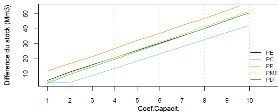
Figure 157: La différence du stock en fonction du coefficient de capacité pour un coefficient de turbinage égal à 3 et pour des prévisions : d'ensemble brutes (PE), climatologiques (PC), parfaites (PP), la moyenne d'ensemble (PME) et la déterministe (PD).
