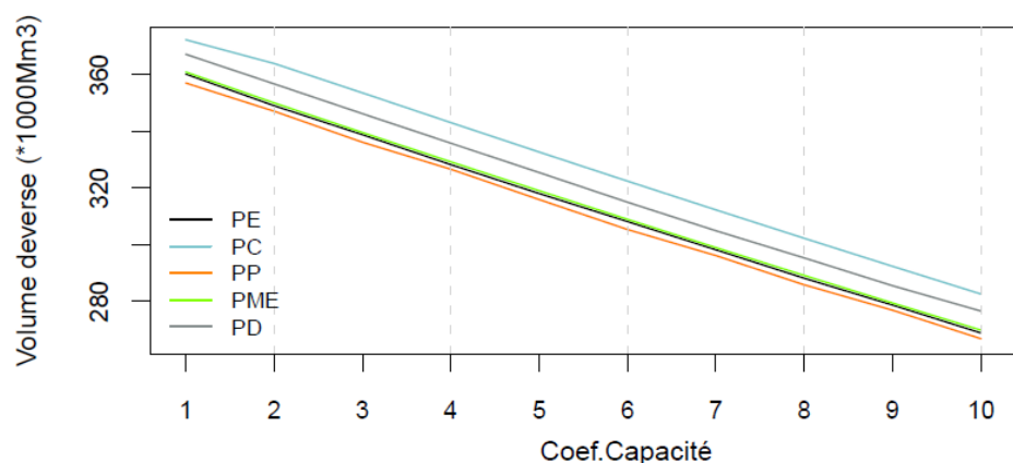
Figure 156: Le volume déversé en fonction du coefficient de capacité pour un coefficient de turbinage égal à 3 et pour des prévisions : d'ensemble brutes (PE), climatologiques (PC), parfaites (PP), la moyenne d'ensemble (PME) et la déterministe (PD).
