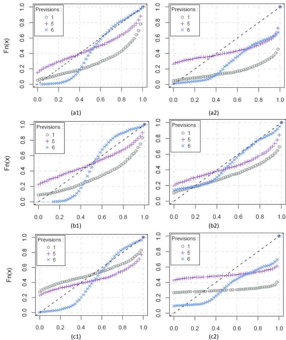
Figure 104 : Diagrammes de probabilité cumulée pour le bassin de (a) la Durance à Serre Ponçon, (b) le Verdon à Castillon et (c) la Romanche à Chambons et pour l'échéance 7 jours. Les graphiques sont calculés à partir des prévisions hydrologiques habillées avec la méthode du meilleur membre et sa modification par Wang et Bishop (2005) et extraites par le modèle hydrologique : (1) MORDOR et (2) GRP.
