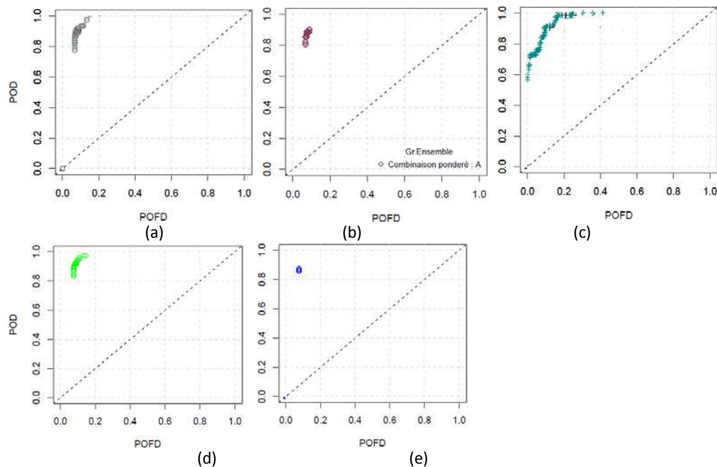
Figure 66 : Courbes ROC pour les prévisions de débit pour le bassin de l'Oise à Sempigny à un horizon de 7 jours tirées du grand ensemble basé sur : (a) l'équiprobabilité de membres, (b) la pondération de la moyenne d'ensemble des différents centres en fonction du score RPS, (c) la pondération en fonction de leur performance selon le RPS. Les prévisions d'ensemble de débit tirées du centre européen et brésilien (d) & (e).
