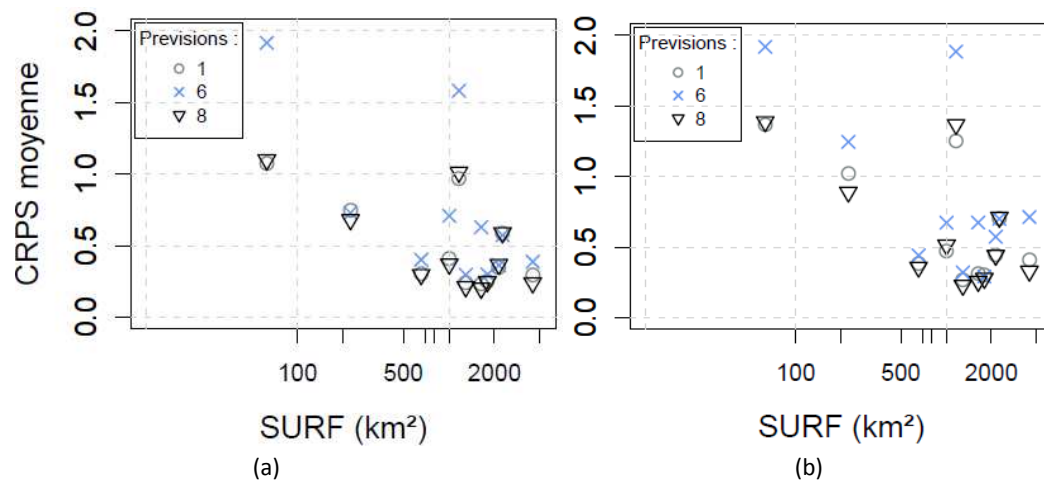
Figure 123 : CRPS moyens de la prévision d'ensemble des débits de bassin brutes fournies par le modèle GRP en fonction de la surface du bassin pour les 11 bassins versants de l'étude et pour les échéances (a) 3 jours et (b) 7 jours. Les graphiques sont calculées à partir des prévisions hydrologiques produites par le modèle MORDOR habillées avec la méthode du meilleur membre modifiée (6) et habillées avec l'erreur de 30% des meilleurs membres (8).
