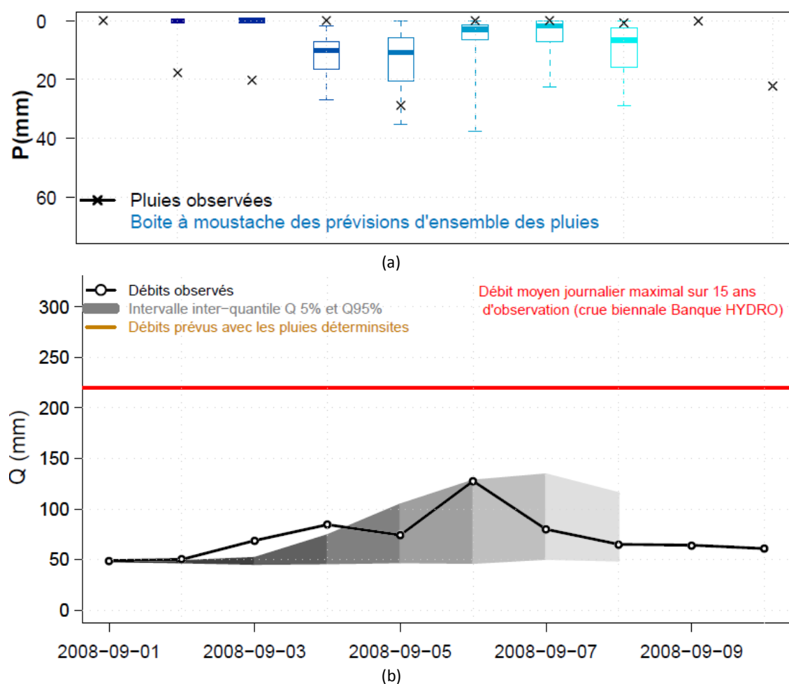
Figure 144 : (a) Boîtes à moustache pour les prévisions d'ensemble de précipitation pour la période de 1 à 9 septembre 2008, (b) l'hydrogramme de débits modélisés par le modèle MORDOR pour la période de 1 à 9 septembre 2008.
