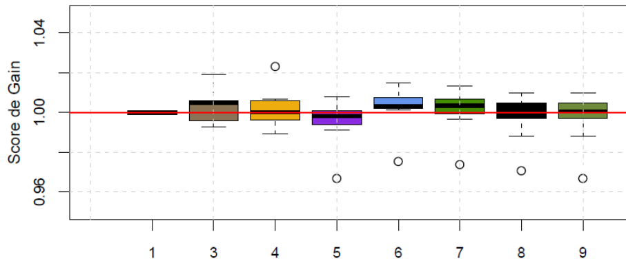
Figure 160: Boîtes à moustaches du score de gain par méthode de post-traitement appliquée. Le graphique présenté correspond à des coefficients de capacité et de turbinage égal à 4 et 3 respectivement.
