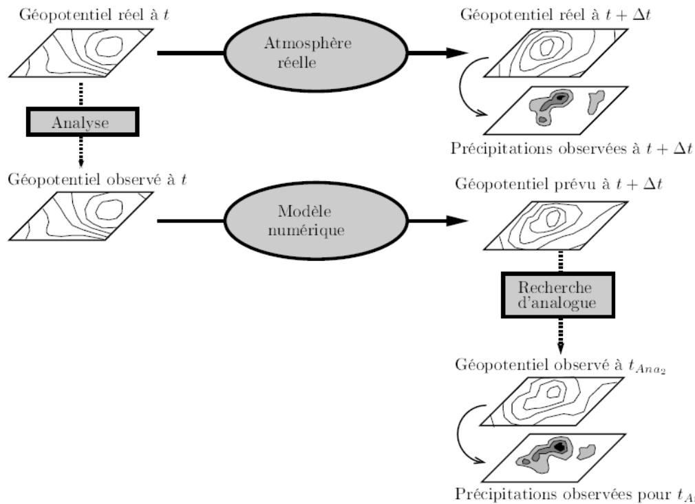
Figure 7 : Description schématique de l'approche de prévisions par analogie (source : Bontron, 2004).
