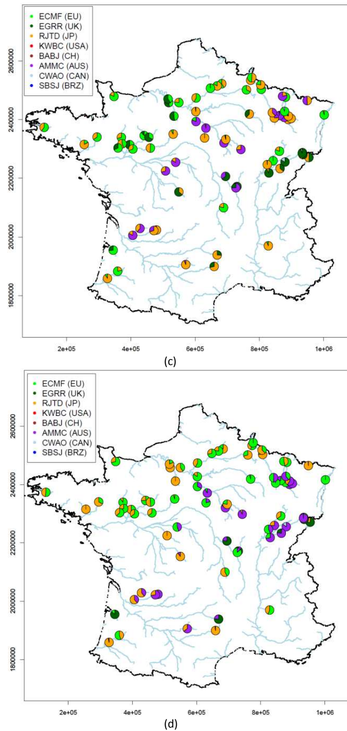
Figure 39 : Carte de localisation des centres qui donnent la meilleure performance selon le critère RPS pour les échéances 3 jours (a), 5 jours (b), 7 jours (c) et 9 jours (d).
