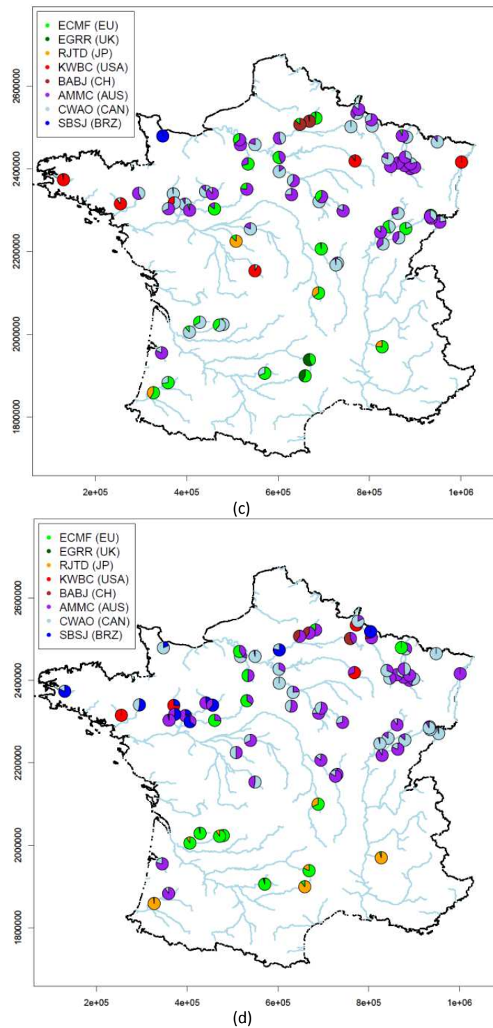
Figure 40 : Carte de localisation des centres qui donnent la meilleure performance selon le critère BSQ90 pour les échéances 3 jours (a), 5 jours (b), 7 jours (c) et 9 jours (d).
