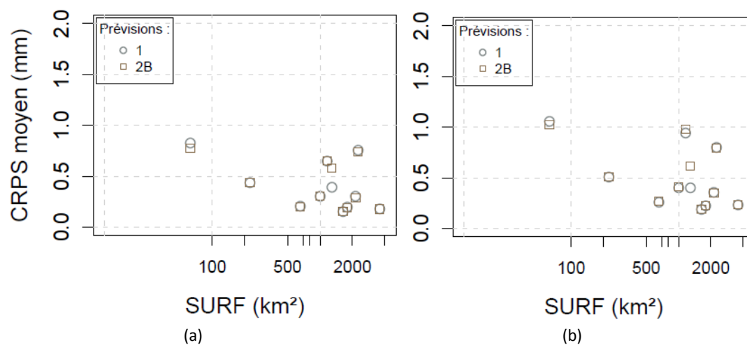
Figure 91 : CRPS moyens de la prévision d'ensemble des débits fournies par le modèle MORDOR en fonction de la surface du bassin pour les 11 bassins versants de l'étude et pour les échéances (a) 3 jours et (b) 7 jours. Les graphiques sont calculés à partir des prévisions de pluies du centre européen brutes (1) et corrigées en utilisant l'information des analogues (2B).
