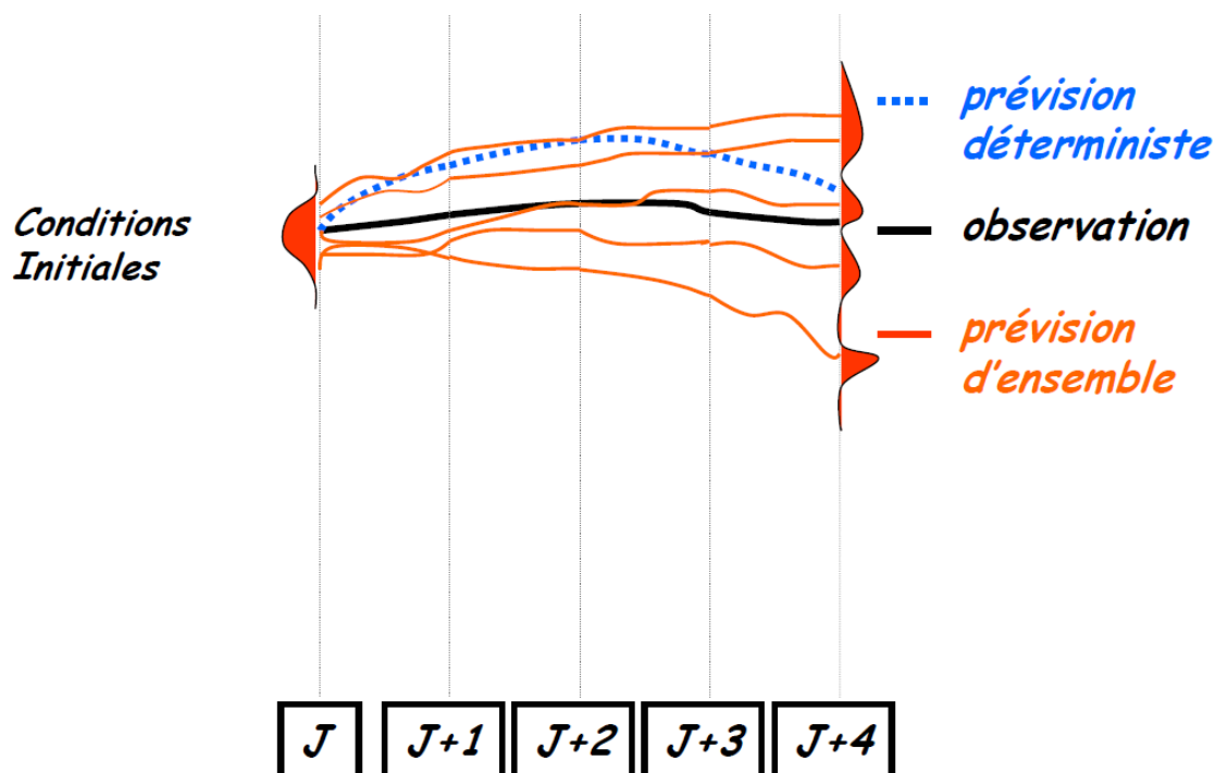
Figure 2: Schéma des prévisions de l'évolution de l'atmosphère pour le cas d'une prévision déterministe et des prévisions d'ensemble et des échéances allant jusqu'à J+4 .
