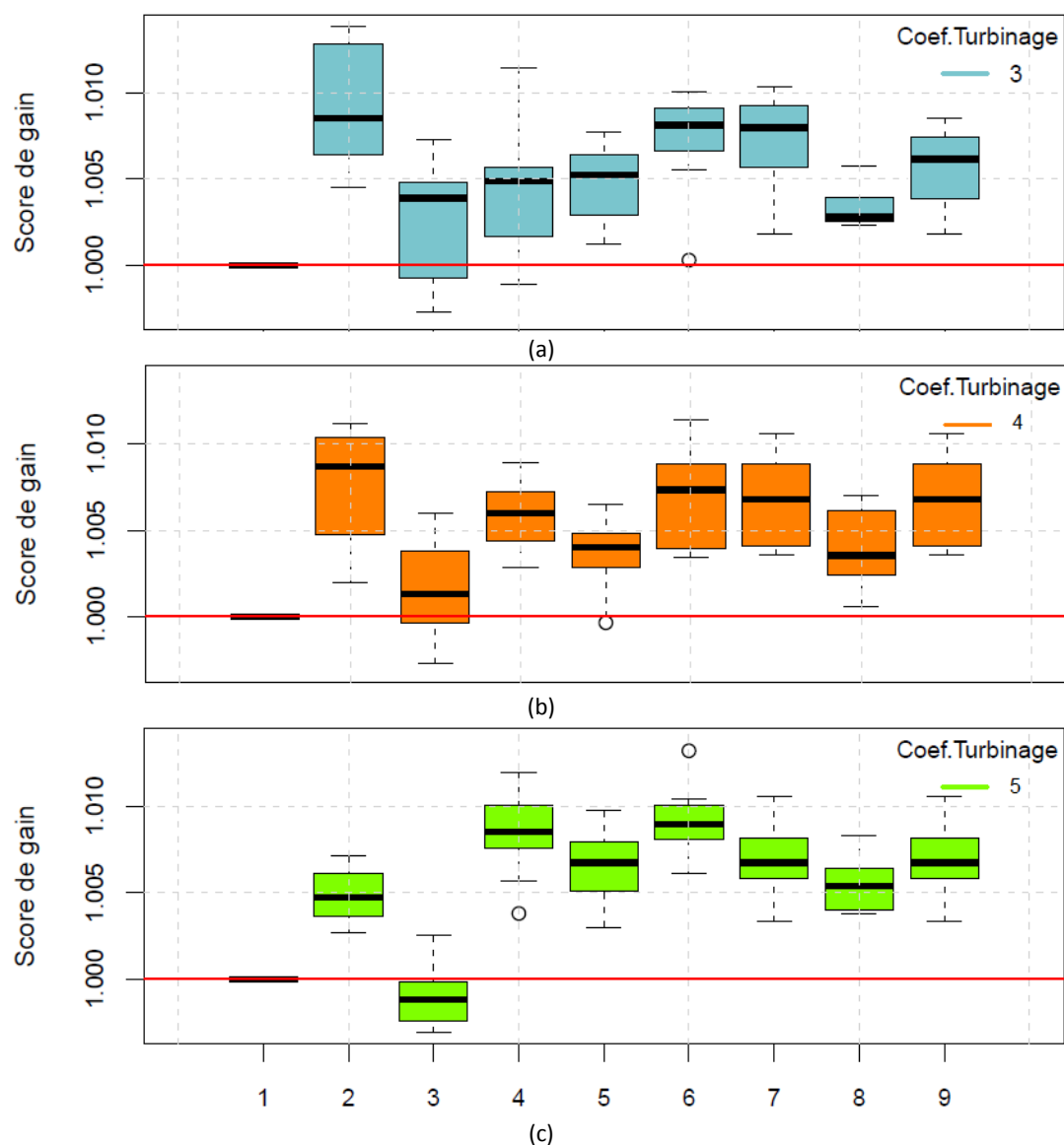
Figure 159: Gain de gestion de turbinage pour les coefficients de turbinage 3(a), 4(b) et 5(c) par type de prévisions : (1) brutes, (2) habillage avec les analogues, (3) habillées avec l'erreur du modèle, (4) habillées avec les analogues et l'erreur du modèle, (5) corrigées avec la BMM (2003), (6) avec la BMM (2005), (7) avec la BMM (2005) modifiée avec la covariance, (8) habillées avec l'erreur de 30% de meilleurs membres et (9) habillées avec la BMM (2006).
