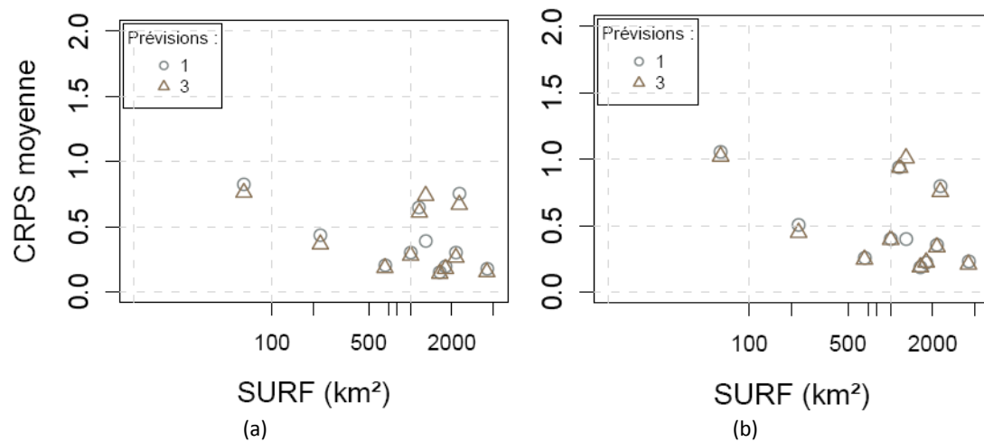
Figure 97 : CRPS moyens de la prévision d'ensemble des débits de bassin brutes fournies par le modèle MORDOR en fonction de la surface du bassin pour les 11 bassins versants de l'étude et pour les échéances (a) 3 jours et (b) 7 jours. Les graphiques sont calculées à partir des prévisions brutes (1) et corrigées avec l'erreur du modèle hydrologique (3).
