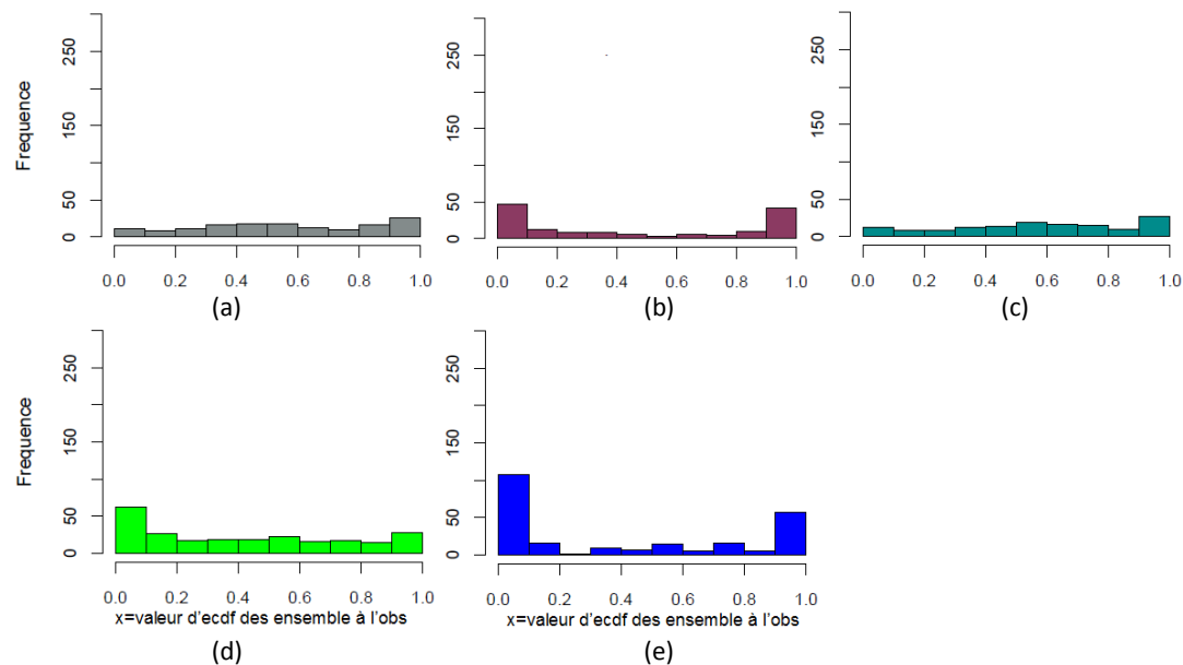
Figure 56 : Histogrammes de PIT pour les prévisions de pluie pour le bassin de l'Oise à Sempigny à un horizon de 7 jours tirées d'un grand ensemble basé sur : (a) l'équiprobabilité de membres, (b) la pondération de la moyenne d'ensemble des différents centres en fonction du score RPS, (c) la pondération en fonction de leur performance selon le RPS. Les prévisions d'ensemble de pluie tirées des centres européen et brésilien évaluées sur les 242 jours sont présentées dans la figure (d) & (e).
