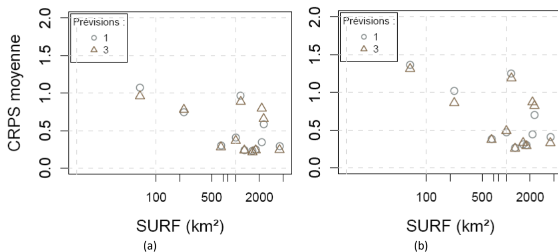
Figure 98 : CRPS moyens de la prévision d'ensemble des débits de bassin brutes fournies par le modèle GRP en fonction de la surface du bassin pour les 11 bassins versants de l'étude et pour les échéances (a) 3 jours et (b) 7 jours. Les graphiques sont calculées à partir des prévisions brutes (1) et corrigées avec l'erreur du modèle hydrologique (3).
