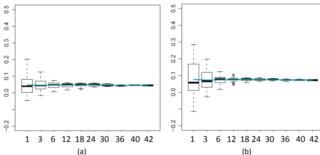
Figure 134 : Boîtes à moustache représentant l'incertitude de l'estimation de la moyenne des erreurs du meilleur membre pour les échéances : (a) 3 et (b) 7 jours. Les boîtes à moustaches sont calculées à partir des prévisions hydrologiques d'ensemble produite par le modèle GRP.
