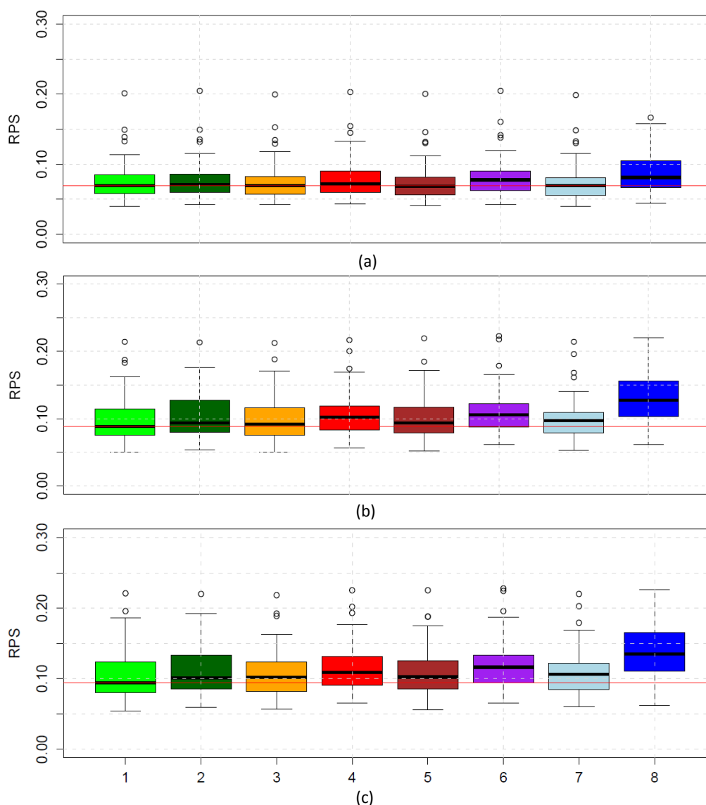
Figure 50 : Boîtes à moustache pour le score de probabilité ordonnée RPS sur les 74 bassins versants étudiés et pour les échéances 3(a), 7(b) et 9(c) jours. Les prévisions de pluie sont issues des centres : (1) ECMF, (2) EGRR, (3) RJTD, (4) KWBC, (5) BABJ, (6) AMMC, (7) CWA0 et (8) SBSJ.
