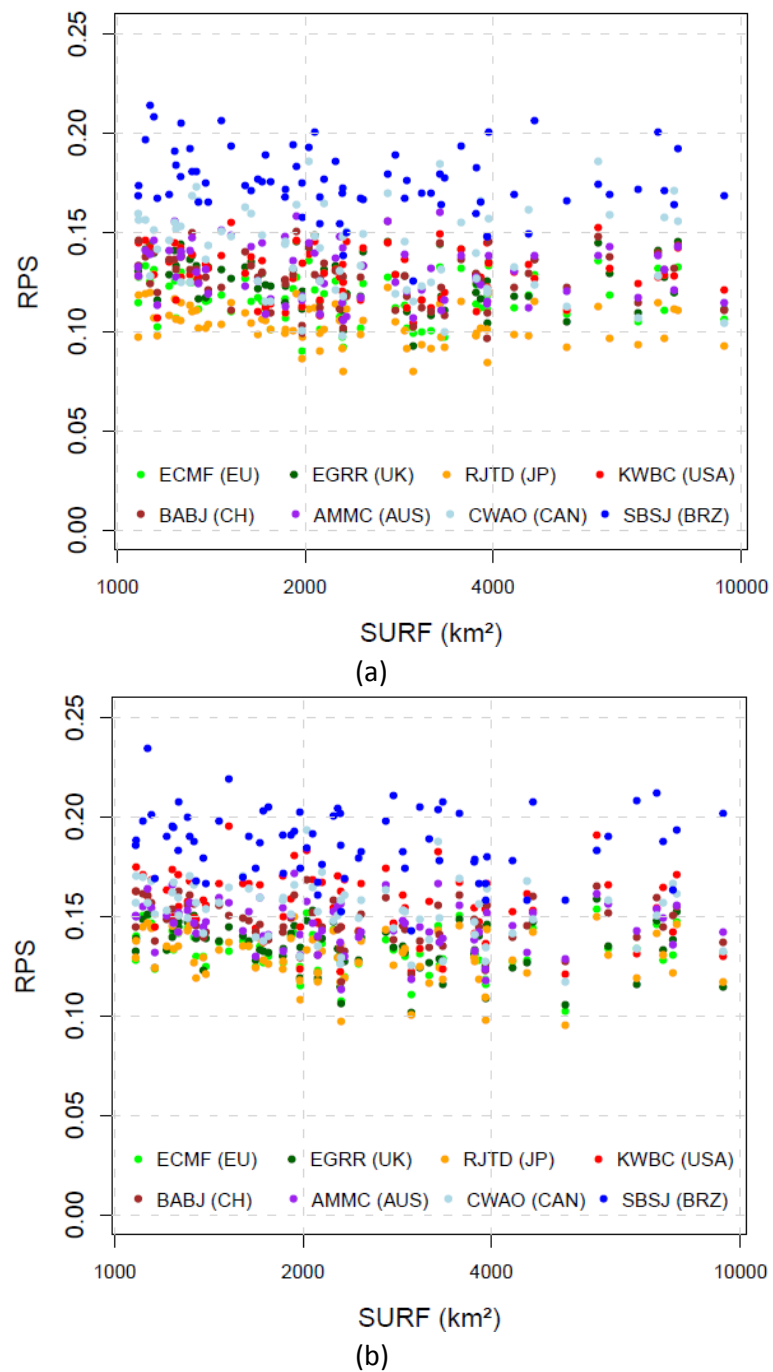
Figure 38 : Graphique du score de probabilité ordonnée RPS en fonction de la surface du bassin versant pour les 74 bassins versants étudiés et pour les échéances 3 (a) et 7 (b) jours. Les prévisions d'ensemble de pluie sont extraites des centres : ECMF (vert clair), EGRR (vert foncé), RJTD (orange), KWBC (rouge), BABJ (marron), AMMC (mauve), CWAQ (ciel) et SBSJ (bleu).
