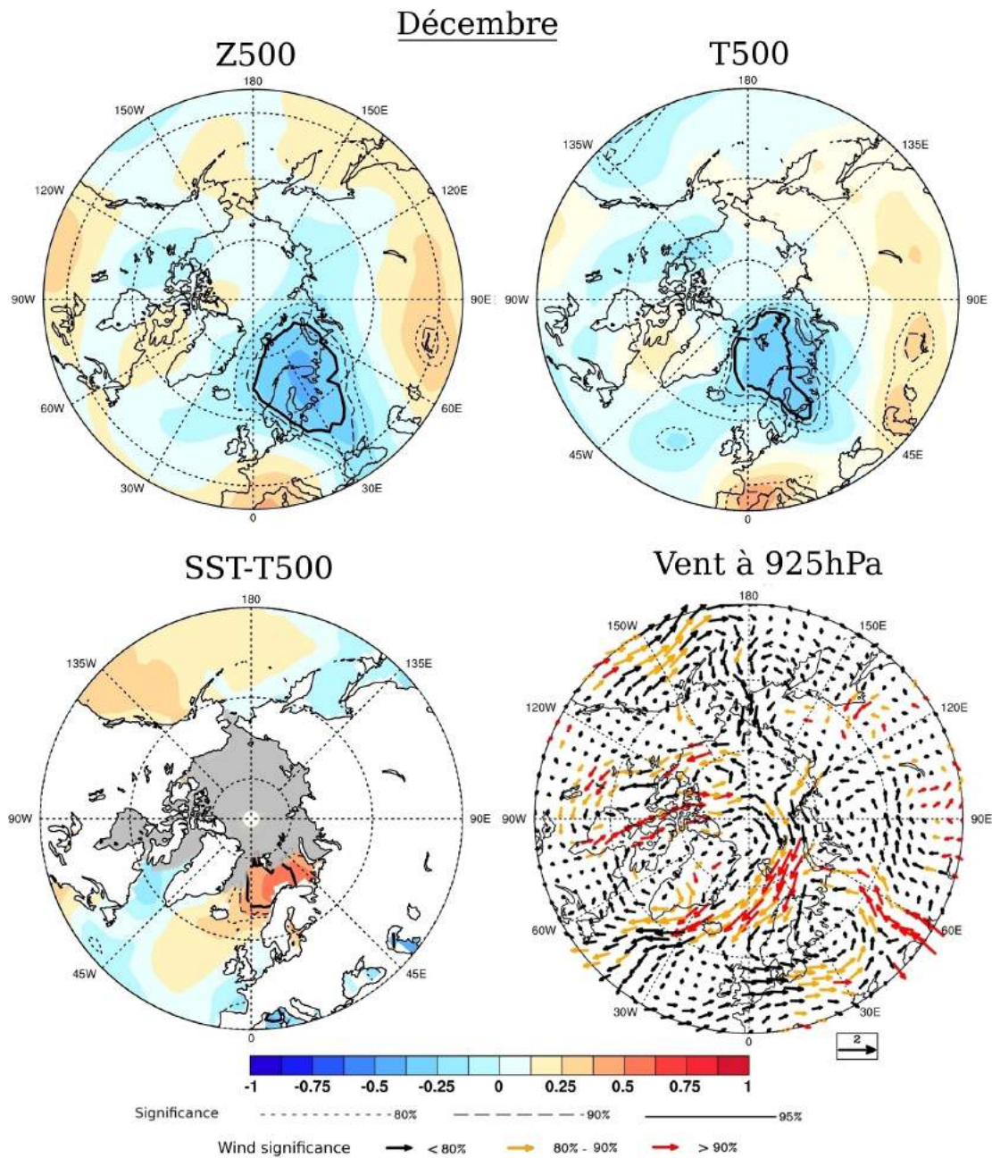
FIG. 5.12 – Corrélation (pour les champs scalaires) et régression linéaire (pour le vent) entre les indices de couverture de glace de mer en septembre observés et détrendés, et respectivement Z500, T500, SST-T500, et le vent à 925 hPa (en m/s par % d'anomalie de couverture de glace) en décembre entre 1979 et 2012. La significativité est indiquée par des lignes pleines et pointillées (champs scalaires), ou par des vecteurs de couleur (champs vectoriels).
