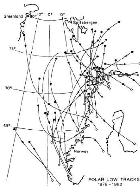
FIG. 2.2 – Trajectoire des polar lows observés par Wilhelmssen entre 1978-1982 (Wilhelmssen, 1985).
