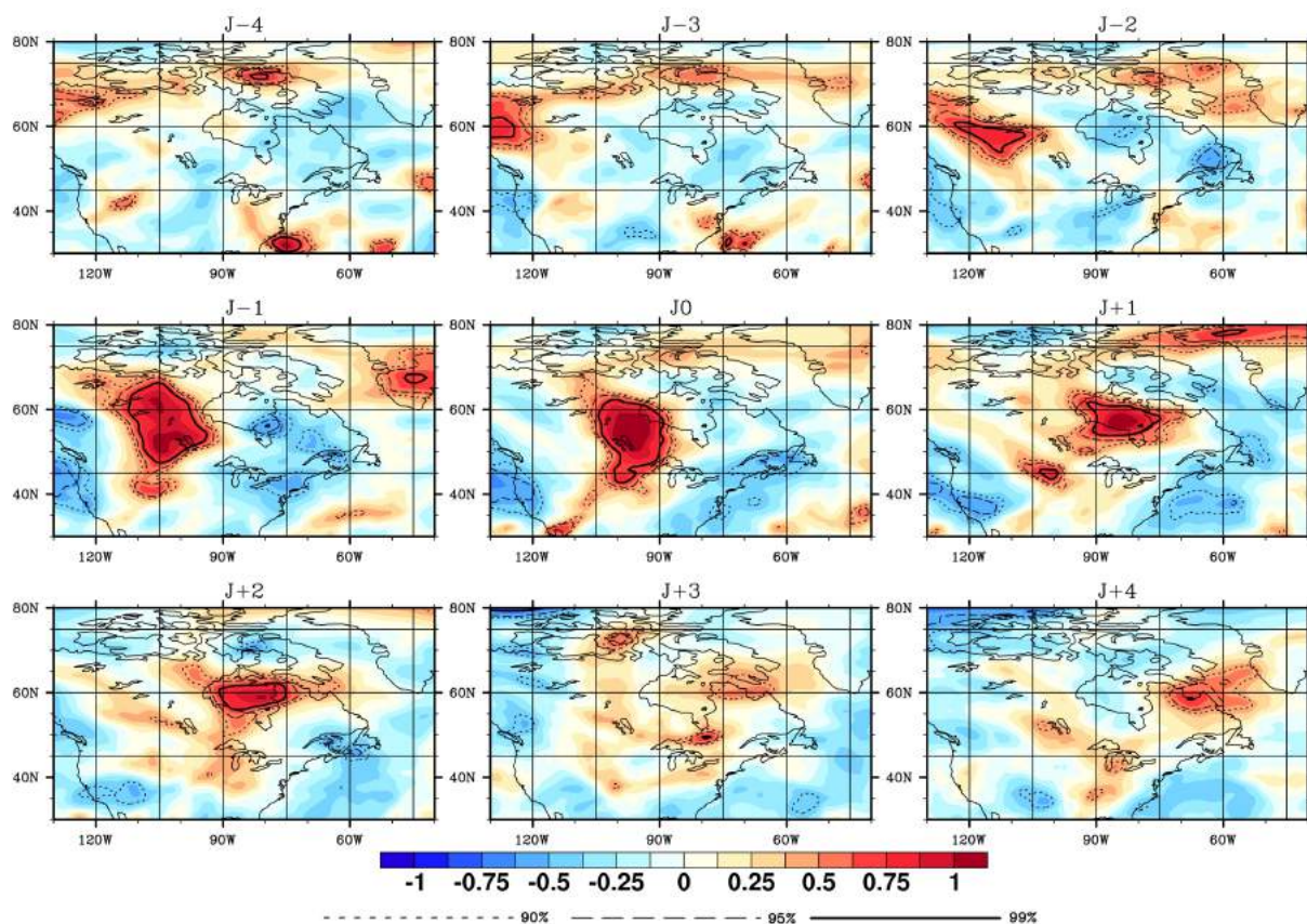
FIG. 3.15 – Évolution du champ d'anomalie de PV300 de 4 jours avant le jour clef à 4 jours après, pour les cas de la liste de Parker en baie d'Hudson ou dans le détroit d'Hudson, pour les mois de saison froide (ONDJFM), de 1977 à 1994. Les niveaux de significativité sont indiqués par des lignes pleines et pointillées.
