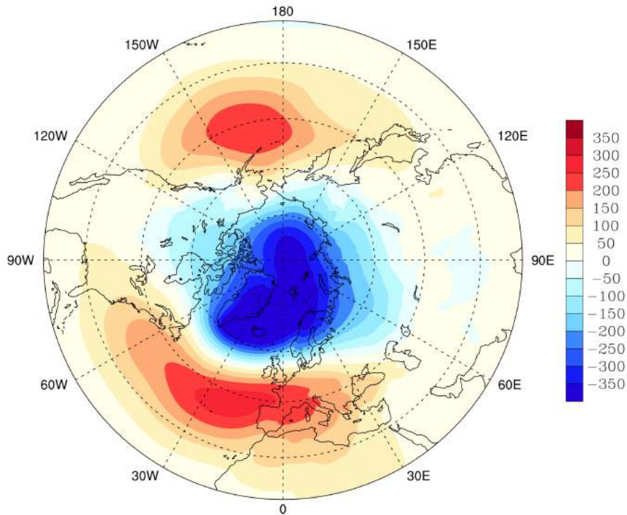
FIG. 4.1 – Structure caractéristique de l'AO : régression linéaire entre l'indice de téléconnexion et la MSLP pour les mois d'hiver (ONDJFM) entre 1979 et 2010 (en Pa).
