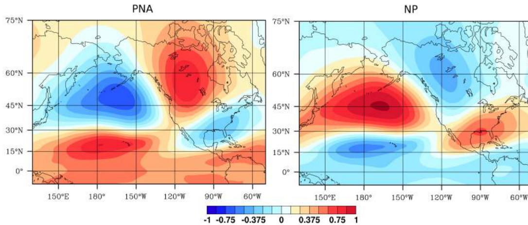
FIG. 4.4 – Structures caractéristiques de la PNA (à gauche) et du NP (à droite) : corrélation entre les indices de téléconnexion et Z500 pour les mois d'hiver (ONDJFM) entre 1979 et 2010.
