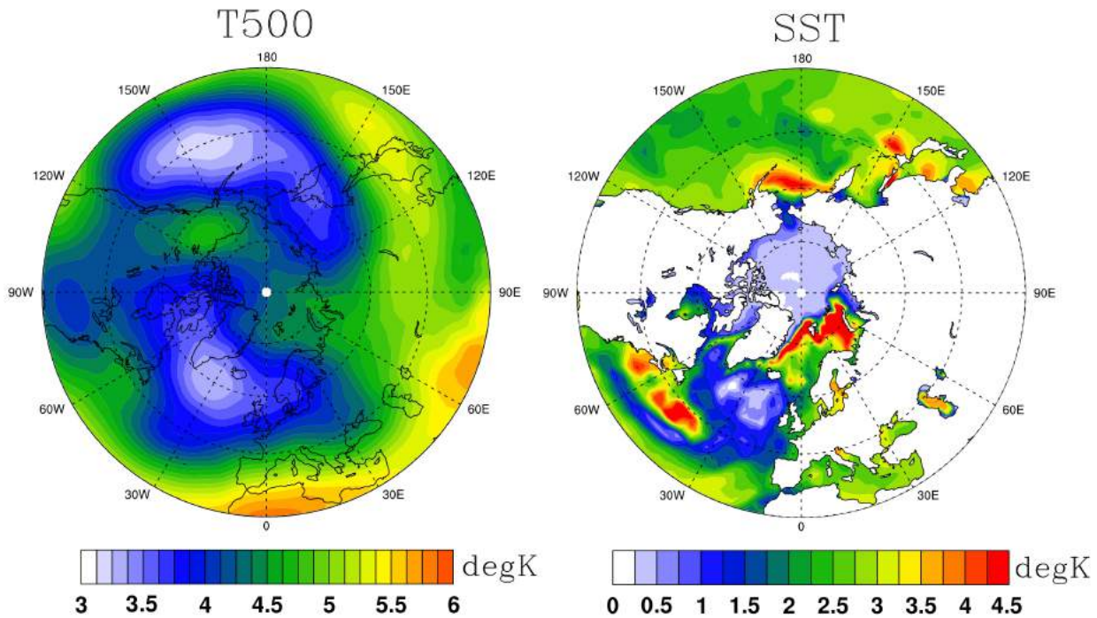
FIG. 5.15 – Différence entre les valeurs hivernales moyennes de T500 (à gauche) et de SST (à droite) entre 1970-1999 (ECHAM5-20C) et 2070-2099 (ECHAM5-A2).
