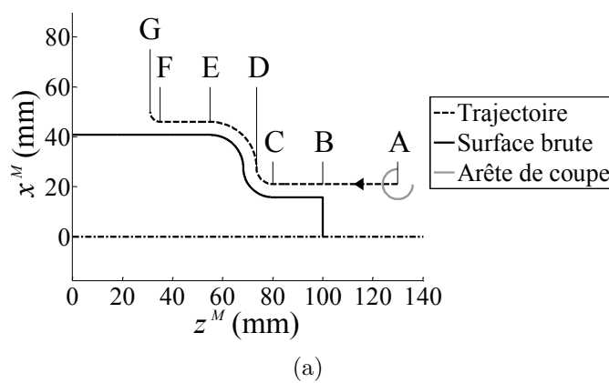
FIGURE 9.2 (a) Trajectoire du contournage ; (b) Essai de contournage instrumenté
