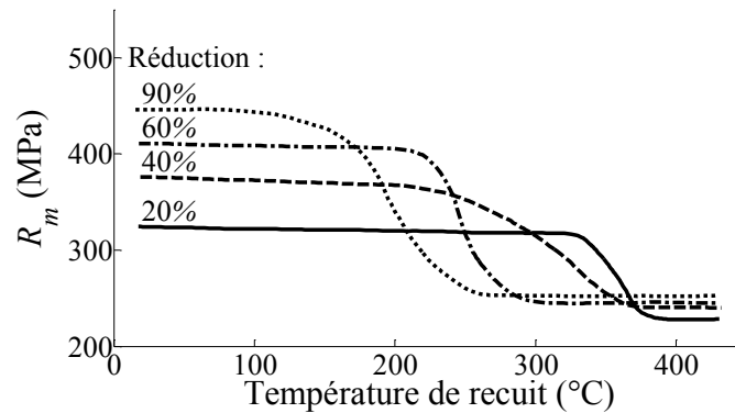
FIGURE 5.1 Lien entre le taux d'écouissage et la température de recuit (30 min) pour du cuivre OFHC (d'après [Barbery 91])
