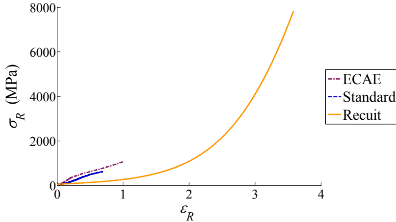
FIGURE 13.11 Courbes rationnelles de traction jusqu'à apparition de la striction
