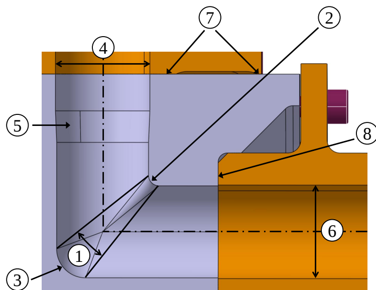
FIGURE 12.4 Détails de conception
