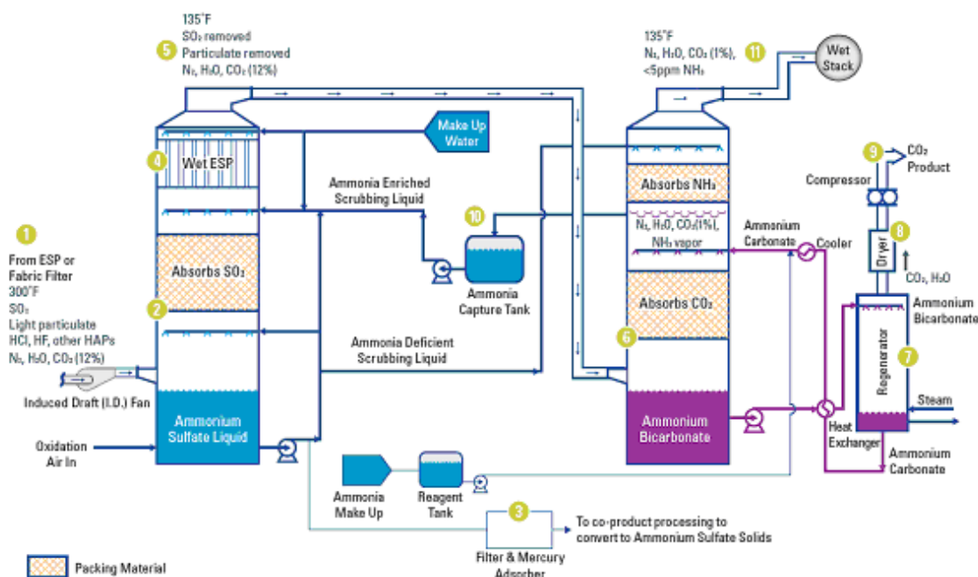
FIGURE 1.6 – Procédé ECO_2
