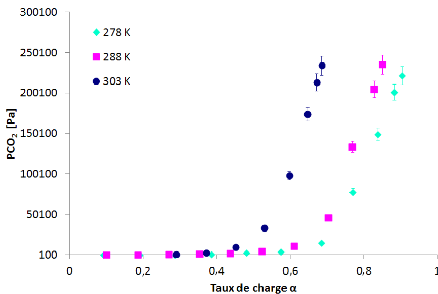
FIGURE 2.6 – Solubilité du CO_2 dans une solution aqueuse d'ammoniac à différentes températures
