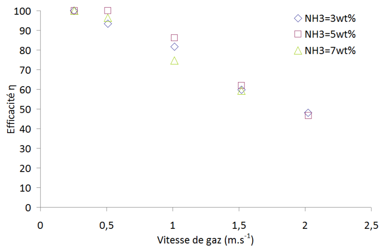
FIGURE 3.12 – Effet de la concentration en NH_3 sur l'efficacité de captage, ( CO_2 = 15 \% , v_{liq} = 0,006 m.s^{-1} )
