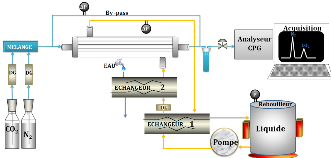
FIGURE 3.2 – Schéma du montage expérimental d'absorption/désorption continu
