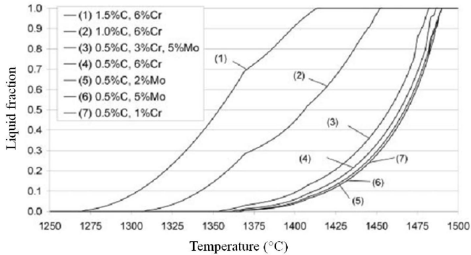
Fig. 1.29. Fraction liquide en fonction de la température pour différentes compositions chimique d'acier: calcul par IDS [70].
