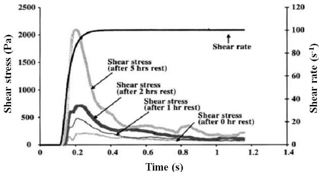
Fig. 1.10. Saut en vitesse de cisaillement de 0 à 100 \text{ s}^{-1} après différents temps d'attente sur un alliage Sn-15Pb avec une fraction solide de 0.36 [18].
