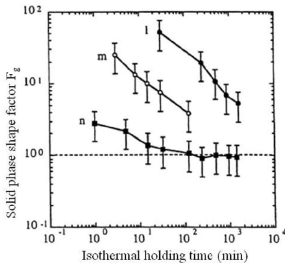
Fig. 1.24. Facteur de forme des particules 1/F_g en fonction du temps de maintien à 580^\circ\text{C} ( f_s=0.5 ) pour un alliage Al-7Si-0.6Mg moulé, sans (l) et avec (m) affinement des grains, et par MHD agitation (n) [63].
