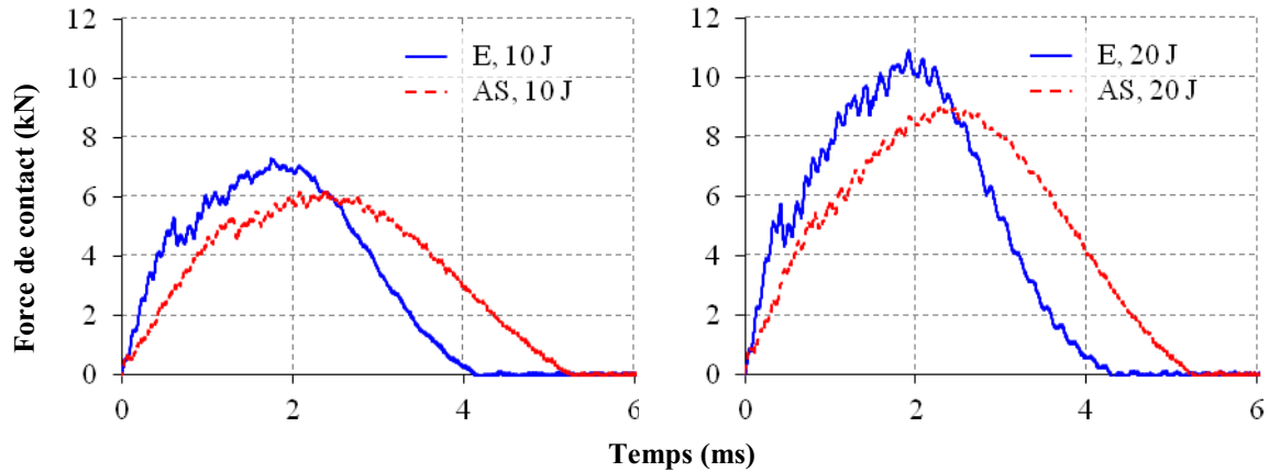
Figure 5.32. Historiques des forces de contact pour l'empilement QI encastré (E) ou simplement appuyé (AS), en impact
