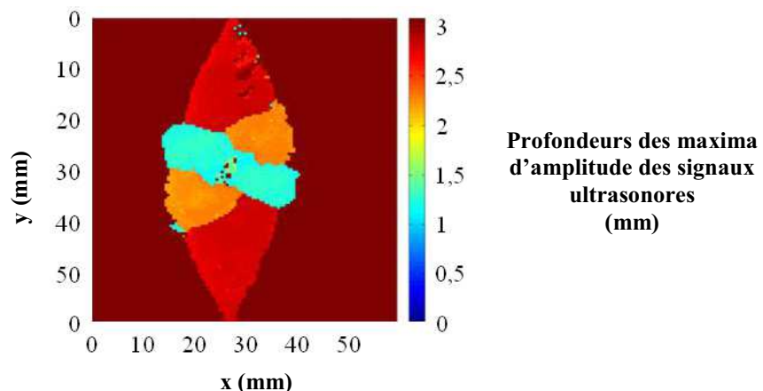
Figure 1.7. Délaminages induits par un impact dans un stratifié de plis unidirectionnels en carbone/époxy [Hautier, 2010]
