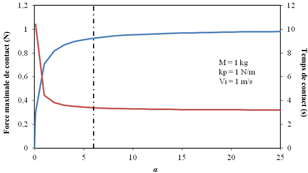
Figure 1.10. Force maximale de contact et temps de contact prévus par le modèle masse-ressort simplifié (Figure 1.9a) en fonction du rapport des raideurs de la plaque et de l'impacteur. La ligne pointillée indique la valeur de \alpha pour laquelle les valeurs asymptotiques sont atteintes à 5 % près.
