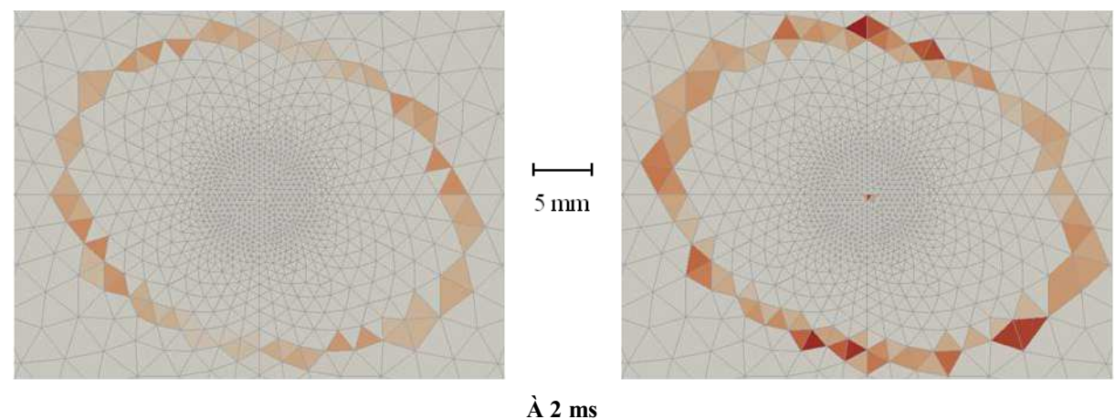
Figure 3.29. Contribution au délaminage, en front de fissure, des différents modes de rupture de la quatrième interface (0°/45°) en partant de la surface non impactée
