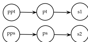
FIGURE 7.6 – L'ensemble pt_{caller} avant l'appel à assignment et sans les champs des structures
