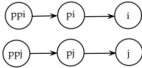
FIGURE 6.1 – Graphe des arcs points-to avant l'appel à swap01
