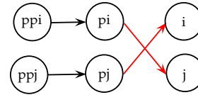
FIGURE 6.2 – Graphe des arcs points-to après l'appel à swap01
