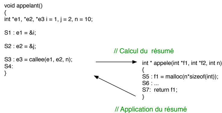
FIGURE 3.8 – Analyse interprocédurale de Wilson
