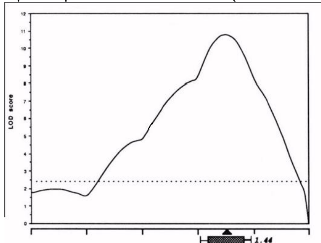
Figure 1.7 : Exemple de profil de vraisemblance (Lander et Botstein, 1989)
