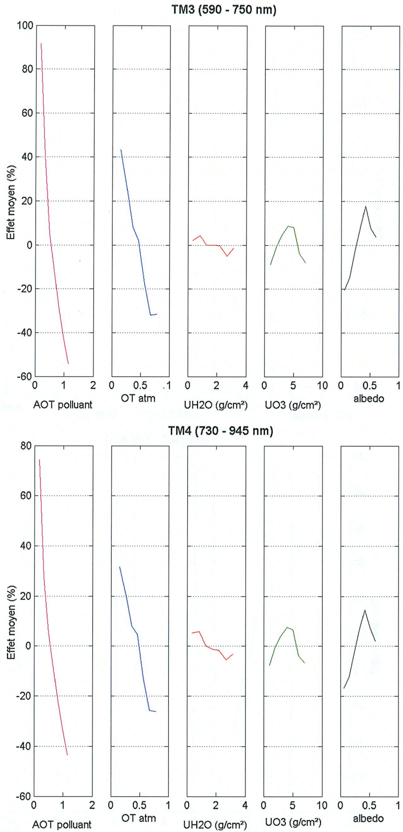
Fig. 5.3 : effet moyen (en %) des paramètres sur la réflectance des canaux TM3 et TM4.
