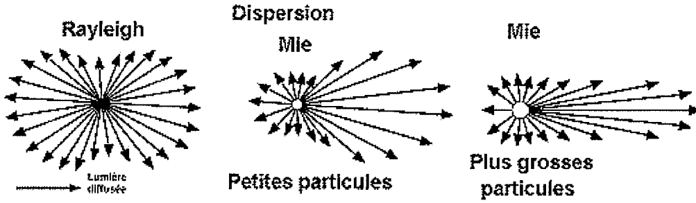
fig. 5.1 : Illustration des différents type de diffusion. Source Wikipédia.
