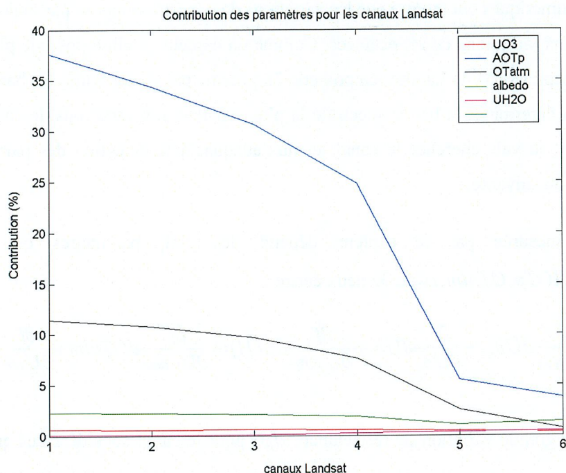
Fig. 5.5 : contribution relative des paramètres aux variations de réflectances du satellite Landsat-TM.
