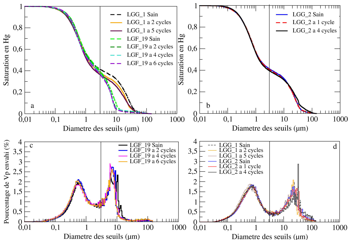
Figure 62 : a) évolutions des courbes de pression capillaires pour le LGG_1 et le LGG_19 séparées de b) par soucis de clarté, b) évolution des courbes capillaires avec l'altération pour LGG_2 c) évolution des courbes des dérivés des pressions capillaires pour LGG_19 et d) LGG_1 et LGG_2
