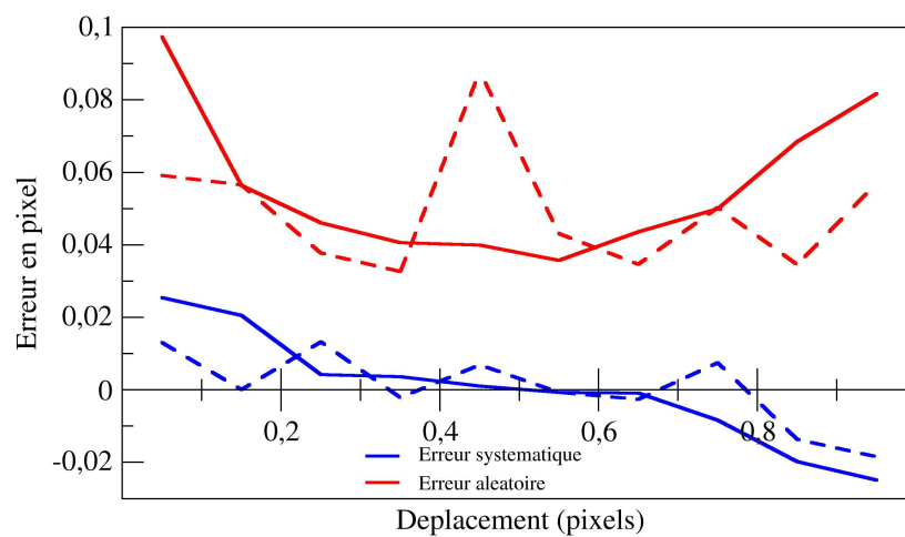
Figure 100 courbes d'erreurs systématiques et aléatoires obtenues sur un mouvement rigide au MEB pour 1600 points de grille: 40x40 domaine de corrélation : 50x50
