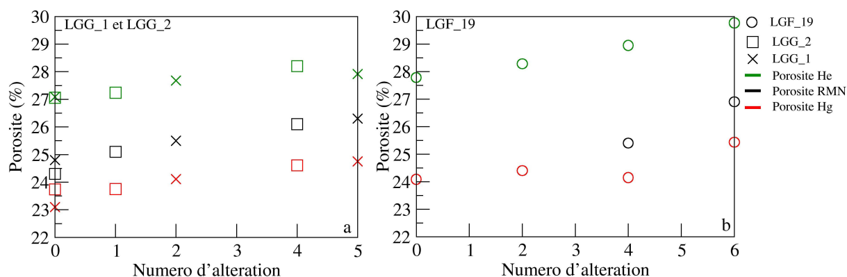
Figure 60 : Comparaison des évolutions de porosité entre a) le LGG_1 et LGG_2 et b) le LGG_1 et LGG_2 et LGF_19 obtenues par porosimétrie mercure, RMN et Hélium
