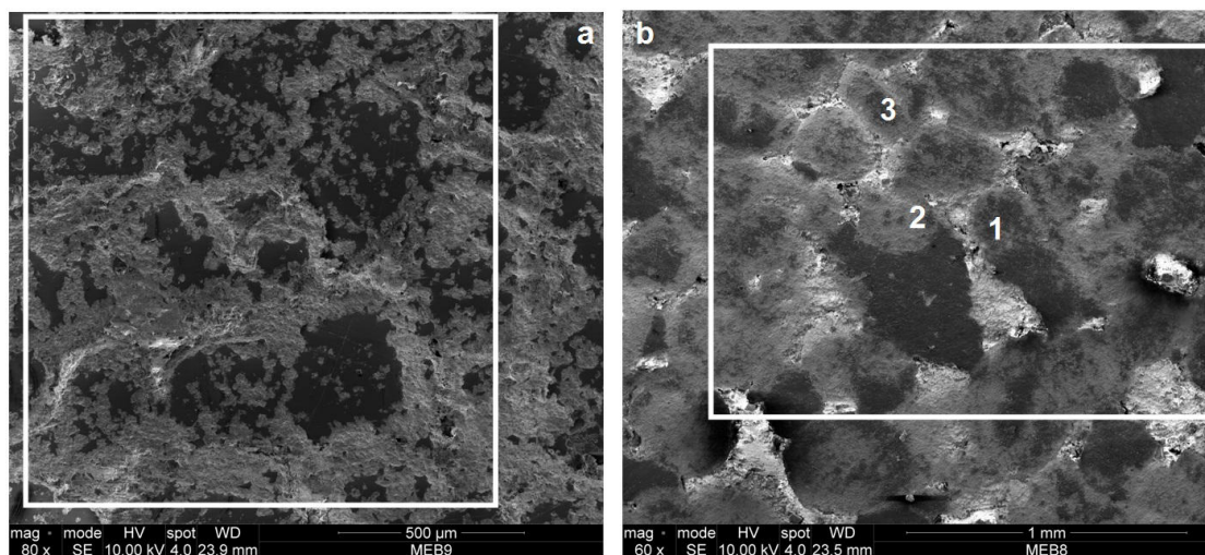
Figure 105: a) microstructure de l'échantillon sain LGG_MEB_9 b) microstructure de l'échantillon altéré six fois LGG_AMEB_5
