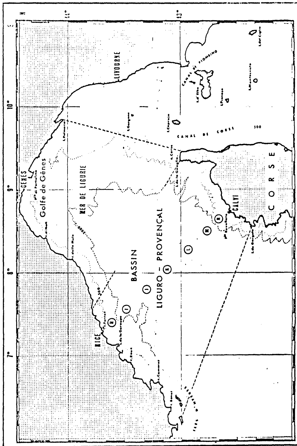
Fig.II.1 Carte du bassin liguro-provençal et position des stations. In GOSTAN (1968)
