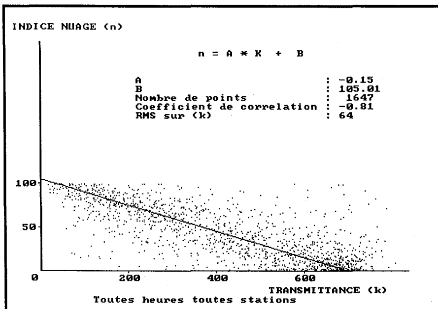
Figure 4.27 : L'indice d'ennuage (n) en fonction de la transmittance globale de l'atmosphère (K) pour les hauteurs du soleil comprises entre 33° et 37° pour l'année 1984.
