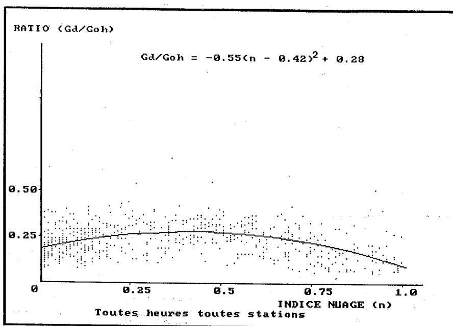
Figure [6.8] : G_d/G_{oh} en fonction de l'indice d'ennuage ( n ) pour les hauteurs du soleil comprises entre 38^\circ et 42^\circ (année 1984).
