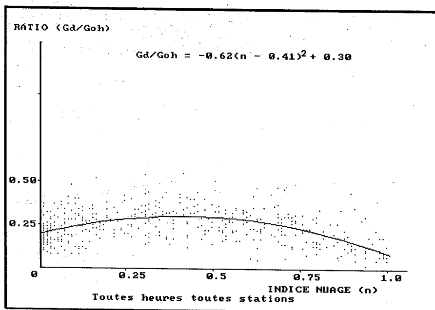
Figure [6.9] : G_d/G_{oh} en fonction de l'indice d'ennuage ( n ) pour les hauteurs du soleil comprises entre 43^\circ et 47^\circ (année 1984).
